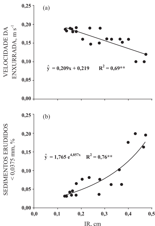
Figura 5. Relação da velocidade da enxurrada (a) e do percentual (base de massa) dos sedimentos erodidos com tamanho < 0,0375 mm (b), ambos avaliados na condição de equilíbrio da enxurrada, com o índice IR da rugosidade superficial do solo criada pelo preparo.
