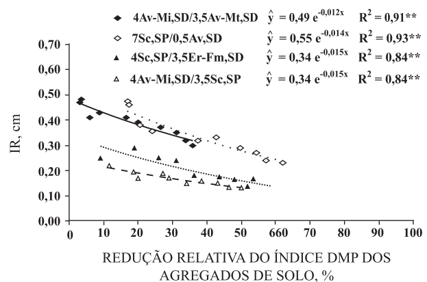
Figura 3. Relação do índice IR da rugosidade superficial do solo criada pelo preparo com a redução relativa percentual (base de massa) do diâmetro médio ponderado (DMP) dos seus agregados nas sequências culturais estudadas (obs.: resultados relativos aos testes de erosão com chuva simulada T3 a T7; em cada um o solo se apresentava mobilizado com grade leve e descoberto).
