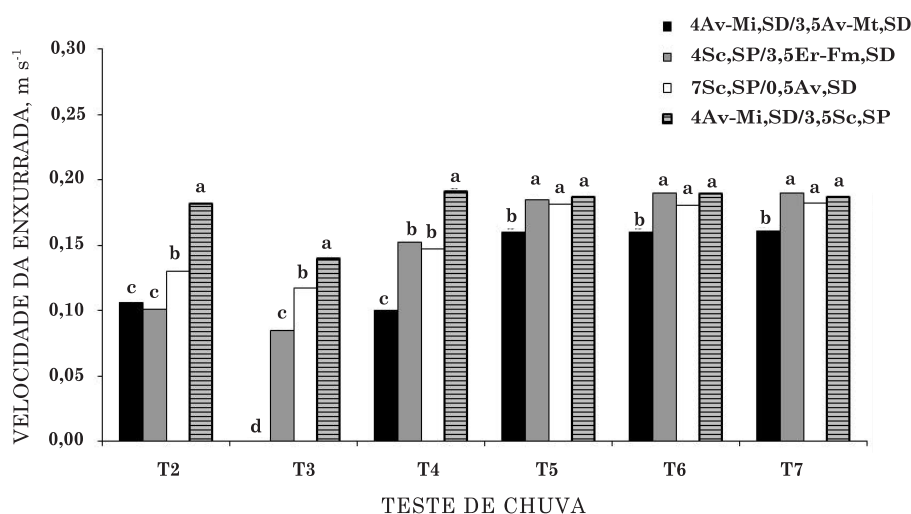
Figura 4. Velocidade da enxurrada na sua condição de equilíbrio, nos testes de erosão com chuva simulada (condição superficial nos testes: T1=solo não mobilizado e completamente coberto; T2=solo não mobilizado e descoberto; T3 a T7=solo sucessivamente mobilizado com grade leve e descoberto) nas sequências culturais estudadas (valores médios de duas repetições por tratamento). Colunas sobrepostas com a mesma letra, no mesmo teste de chuva, não diferem estatisticamente entre si (Duncan, p < 0,05 ).
