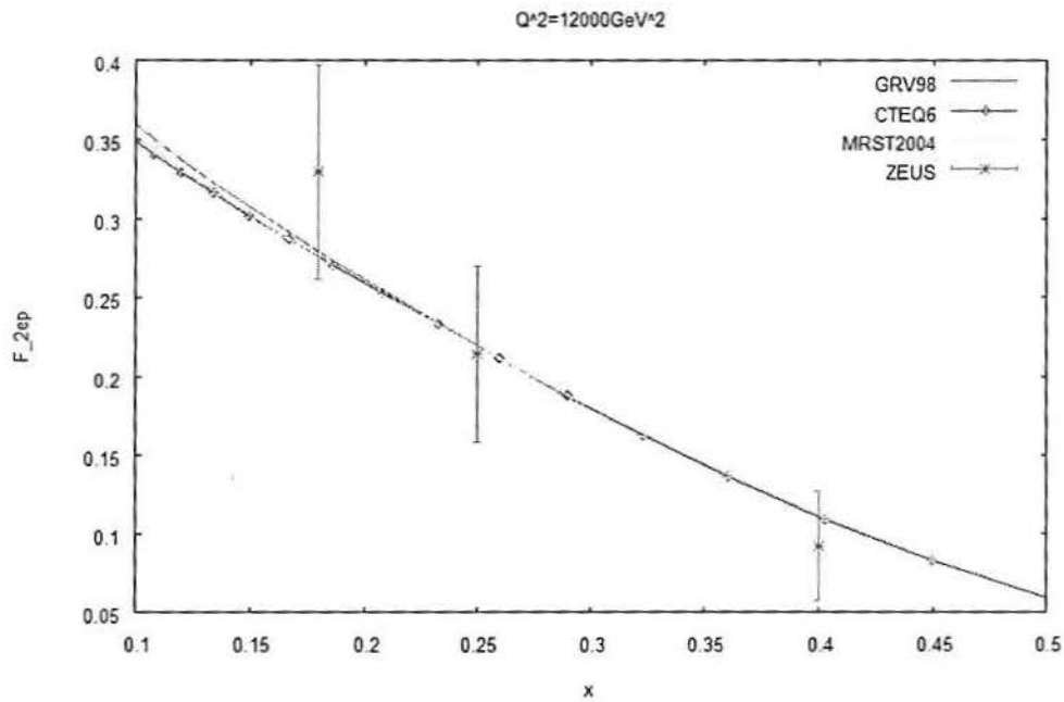
Figura 5.4: Funções de estrutura F_2 , comparadas com os dados obtidos a partir do detetor ZEUS, para Q^2 = 12000\text{GeV}^2 .
