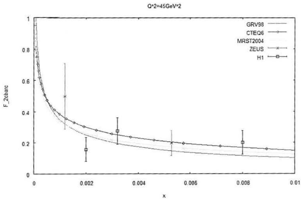
Figura 5.8: Funções de estrutura F_2^{c\bar{c}} , comparadas com os dados obtidos a partir do detetor ZEUS e do detetor H1, para Q^2 = 45\text{GeV}^2 .
