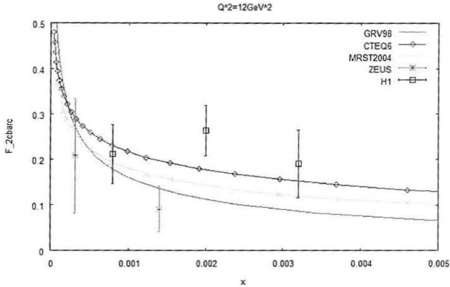
Figura 5.6: Funções de estrutura F_2^{c\bar{c}} , comparadas com os dados obtidos a partir do detector ZEUS e do detector H1, para Q^2 = 12\text{GeV}^2 .
