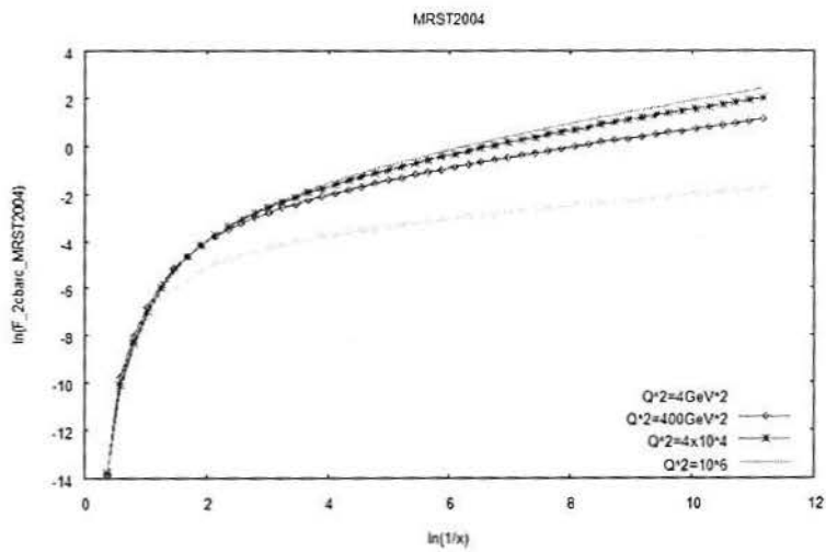
Figura 4.6: Funções de estrutura F_2^{c\bar{c}} , para determinados valores de Q^2 em função de \ln(1/x) , obtida a partir da distribuição partônica MRST2004.
