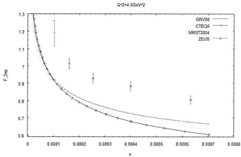
Figura 5.1: Funções de estrutura F_2 , comparadas com os dados obtidos a partir do detector ZEUS, para Q^2 = 4.5\text{GeV}^2 .
