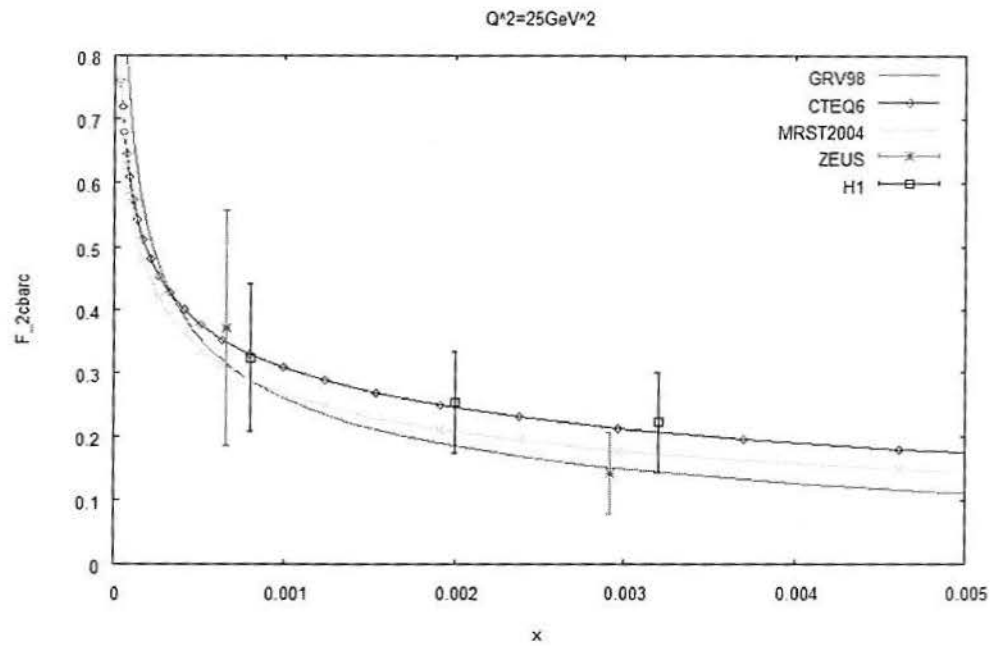
Figura 5.7: Funções de estrutura F_2^{c\bar{c}} , comparadas com os dados obtidos a partir do detetor ZEUS e do detetor H1, para Q^2 = 25\text{GeV}^2 .
