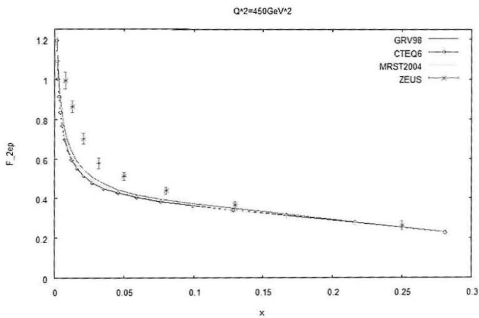
Figura 5.2: Funções de estrutura F_2 , comparadas com os dados obtidos a partir do detector ZEUS, para Q^2 = 450\text{GeV}^2 .
