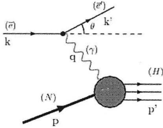
Figura 1.1: Espalhamento de um elétron com um próton.
