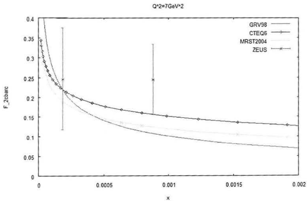
Figura 5.5: Funções de estrutura F_2^{c\bar{c}} , comparadas com os dados obtidos a partir do detetor ZEUS, para Q^2 = 7\text{GeV}^2 .
