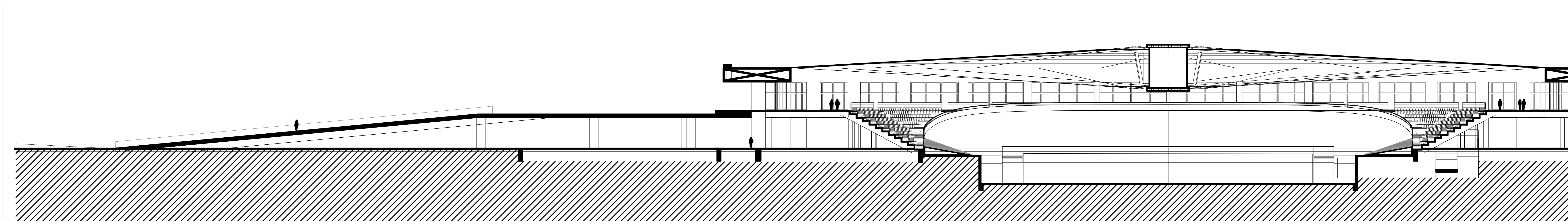
VELÓDROMO - CORTE TRANSVERSAL - esc.: 1/250
