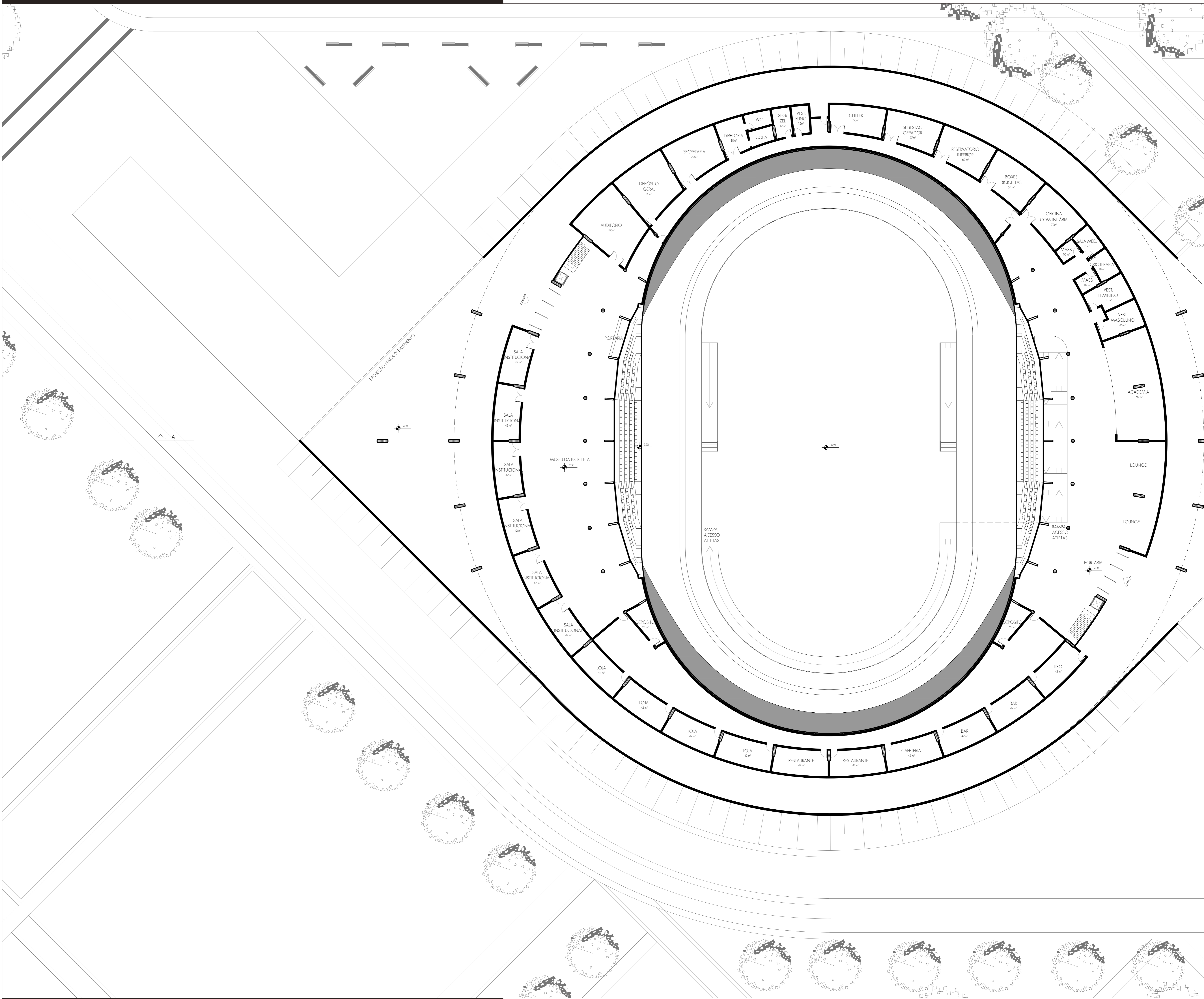
VELÓDROMO - FACHADA SUDOESTE- esc.: 1/250
