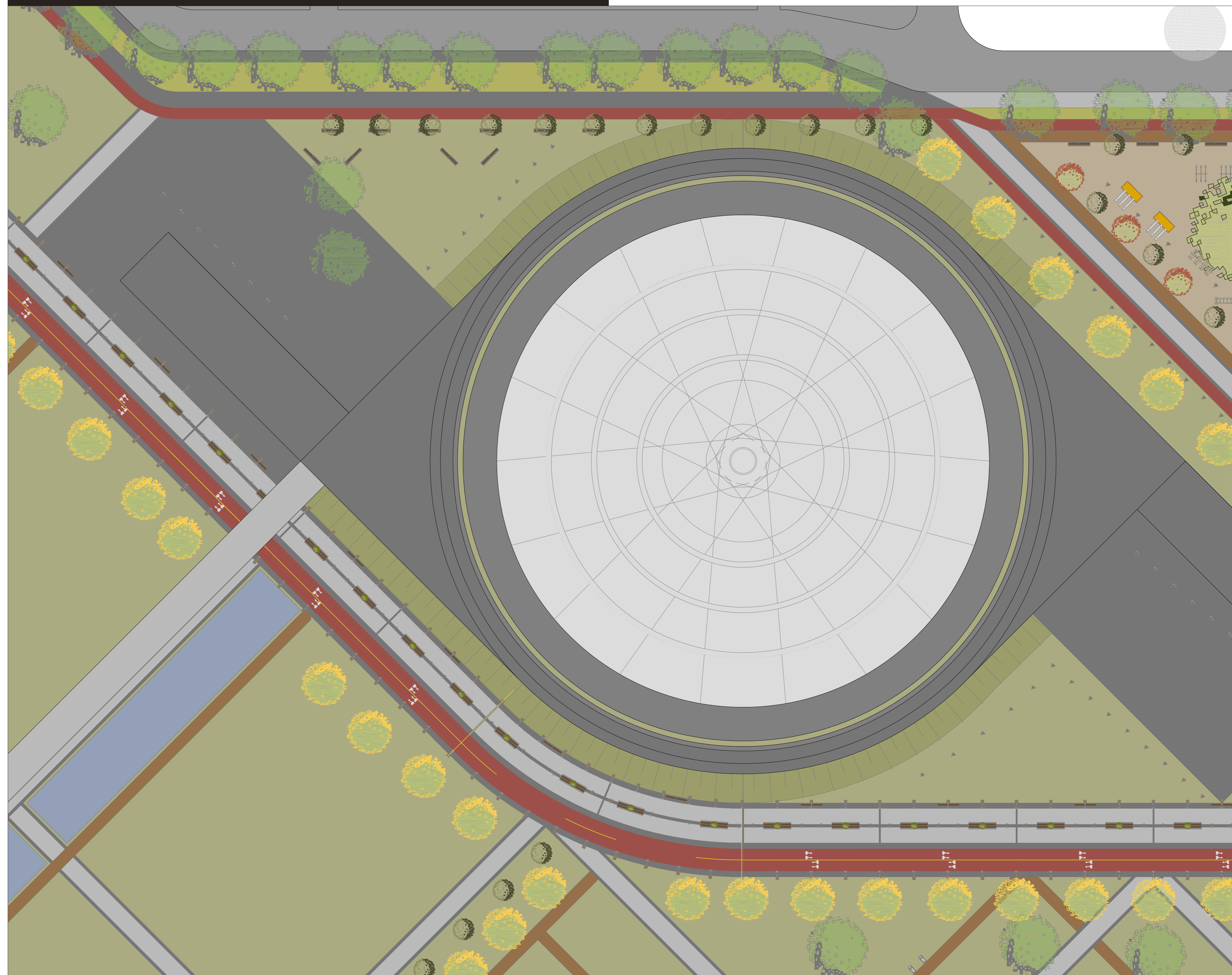
PRAÇA SECA- esc.: 1/500
