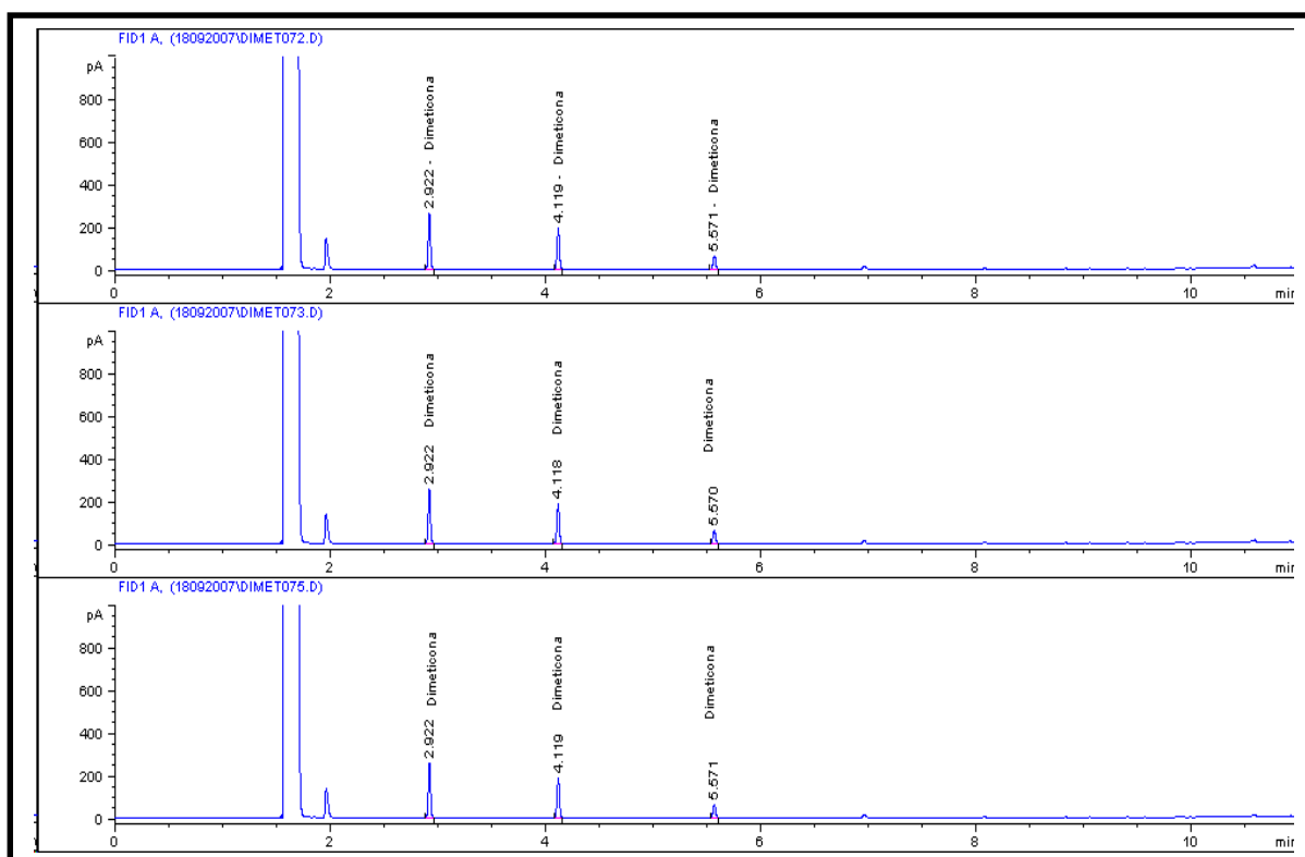
Figura 22: Cromatogramas das triplicatas do padrão de referência de dimeticona por cromatografia gasosa para matéria-prima de simeticona 100%
