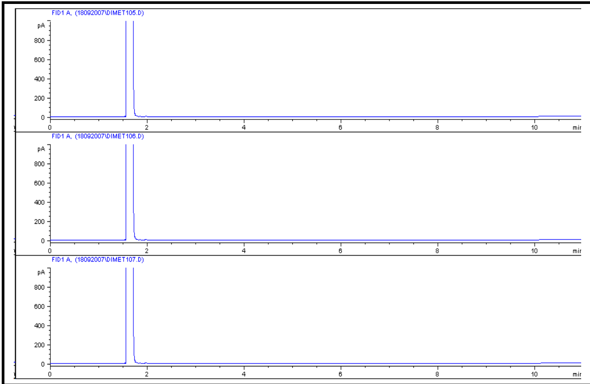
Figura 23: Cromatogramas das triplicatas da amostra Branco (hexano) por cromatografia gasosa para a matéria-prima de Simeicona 100%
