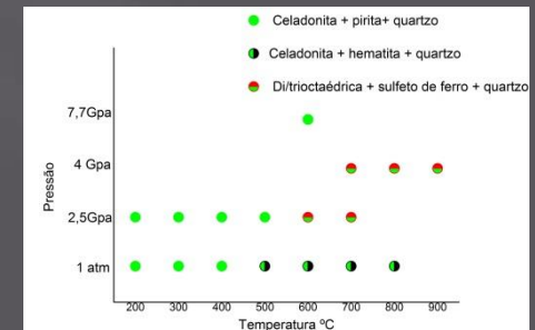
Figura 6 : Diagrama Pressão x Temperatura
