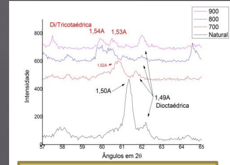
Figura 4 : Processamentos a 4Gpa.
