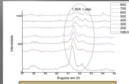
Figura 3 : Processamentos a 1 Atm.
