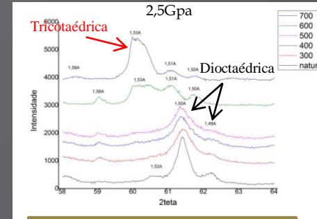
Figura 2: DRX com passo de 8s no intervalo entre 58° e 64°.
