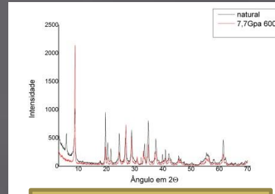
Figura 5 : Processamento a 7,7Gpa
