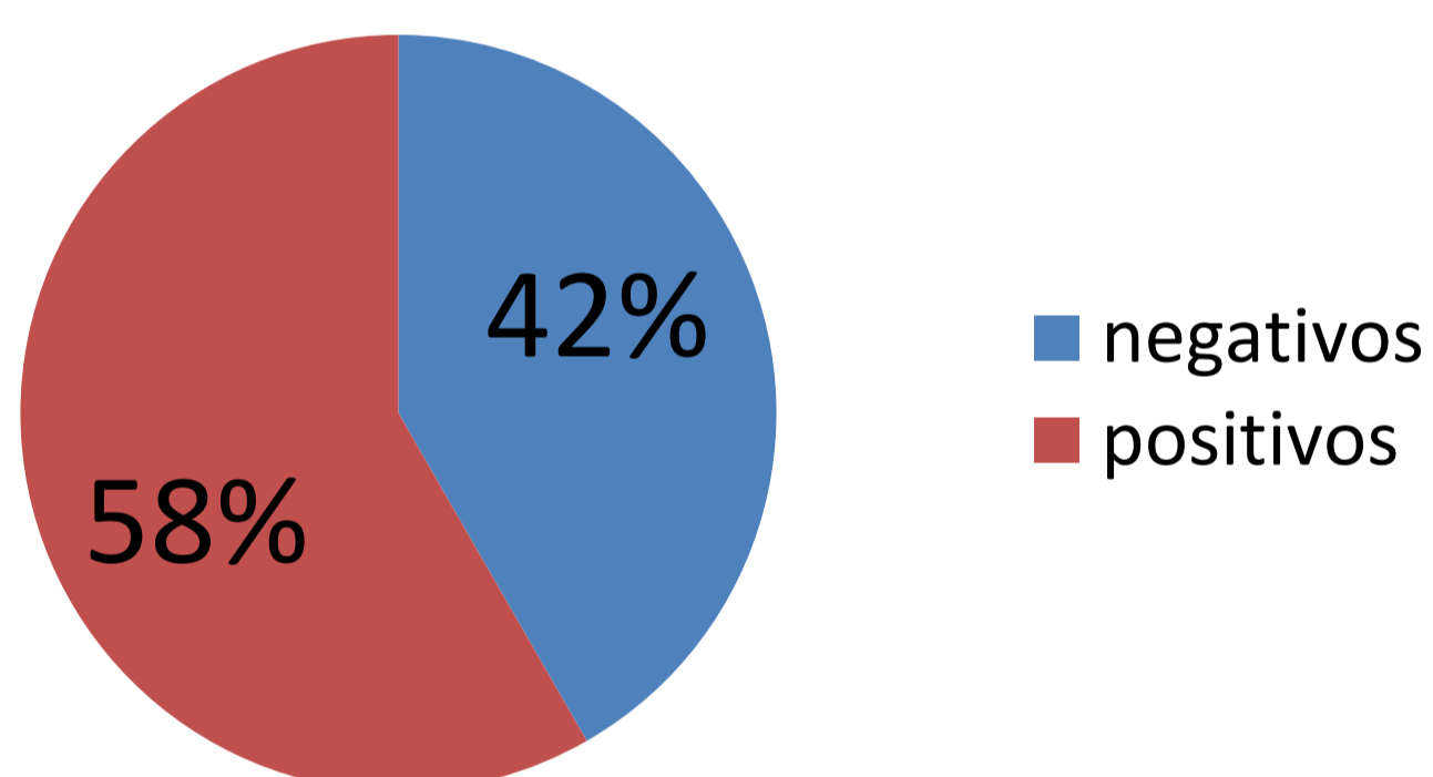
Figura 2. Confirmação laboratorial de suspeitas clínicas da raiva bovina, IPVDF 2011 a 2015 (N=988).
