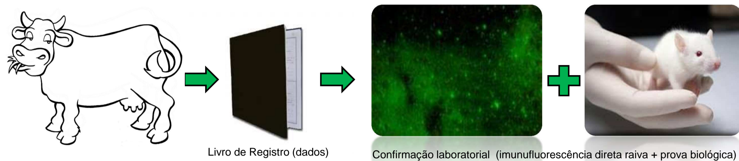
Figura 1. Fluxograma da investigação laboratorial de suspeita de raiva (MAPA, 2009)
