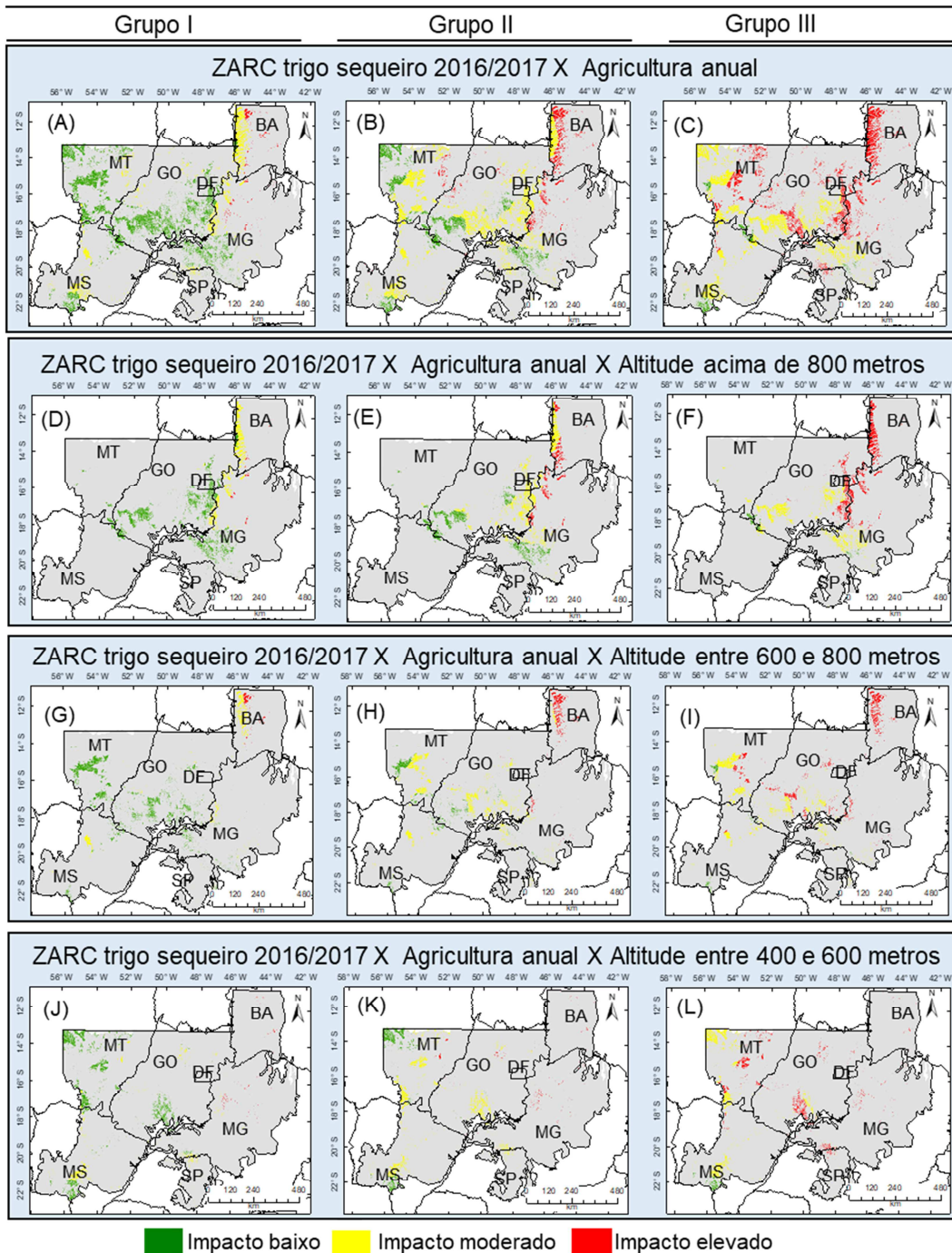
FIGURA 20. Distribuição espacial das áreas favoráveis para cultivares de trigo sequeiro, Grupo I (A, D, G, J), Grupo II (B, E, H, K) e Grupo III (C, F, I, L), considerando os níveis de impacto por restrição hídrica baixo, moderado e elevado, na Região Homogênea de Adaptação de Cultivares de Trigo 4 (RHACT 4), bioma Cerrado, solos Tipo 3 com capacidade de armazenamento de água disponível de 75 mm , nível de risco de 40% , considerando o cruzamento dos planos de informação do ZARC trigo sequeiro 2016/2017 com a agricultura anual (A, B e C) e deste cruzamento com a faixa de altitude acima de 800 m (D, E e F), entre 600 e 800 m (G, H e I) e entre 400 e 600 m (J, K, L) para semeadura em 5 de fevereiro. Fonte: adaptada de BRASIL (2015 e 2016) e USGS (2016).
