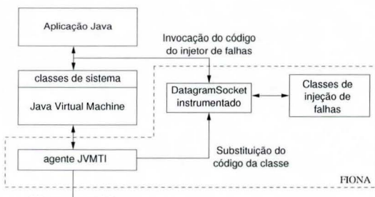
Figura 1: Arquitetura de FIONA
