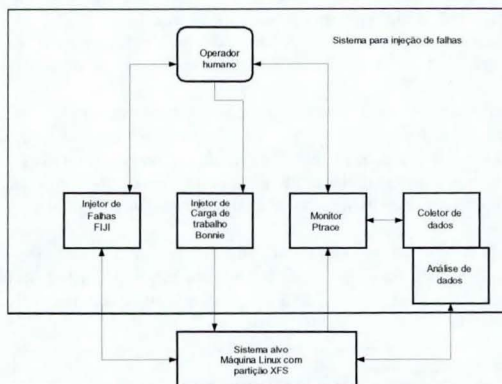
Figura 1 – Ambiente para injeção de falhas
