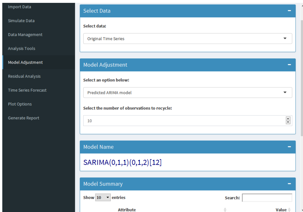
Figura 5.35: Tela de Model Adjustment “reciclando” as 10 últimas observações da série com o objetivo de testar a previsão do modelo
