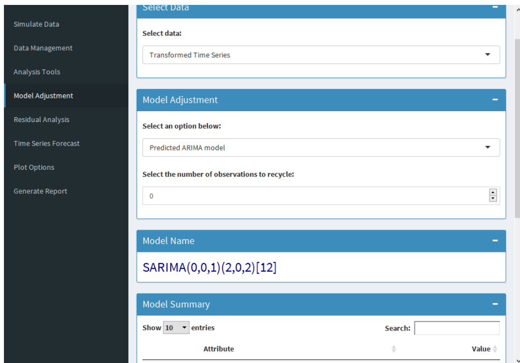
Figura 5.22: Tela de Model Adjustment com o modelo predito da família SARIMA para a série transformada, suas estimativas, erros padrões e AIC
