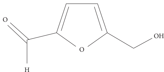
5-hidroximetil-2-furaldeído HMF
