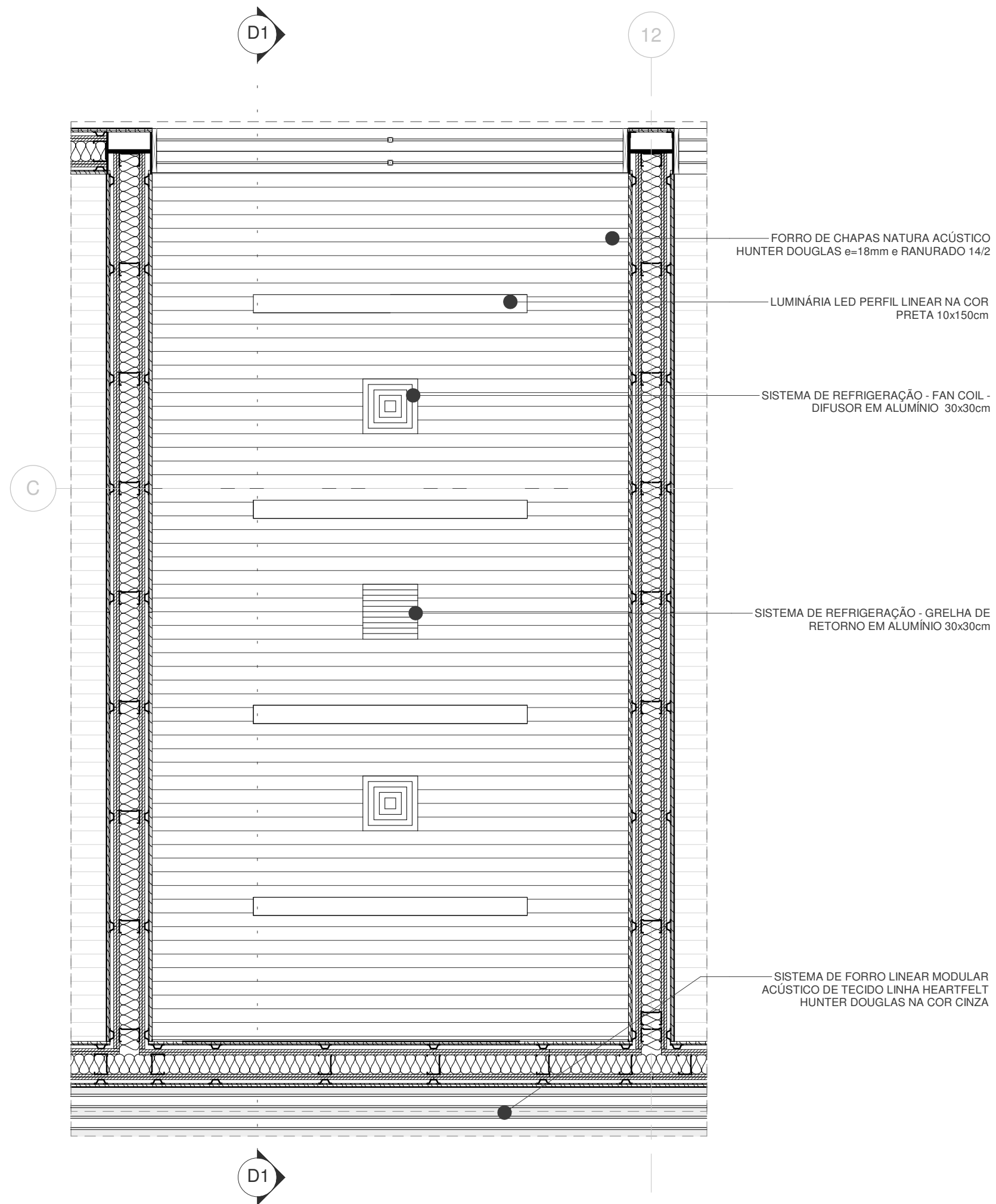
PLANTA DE FORRO - SALA DE MÚSICA
