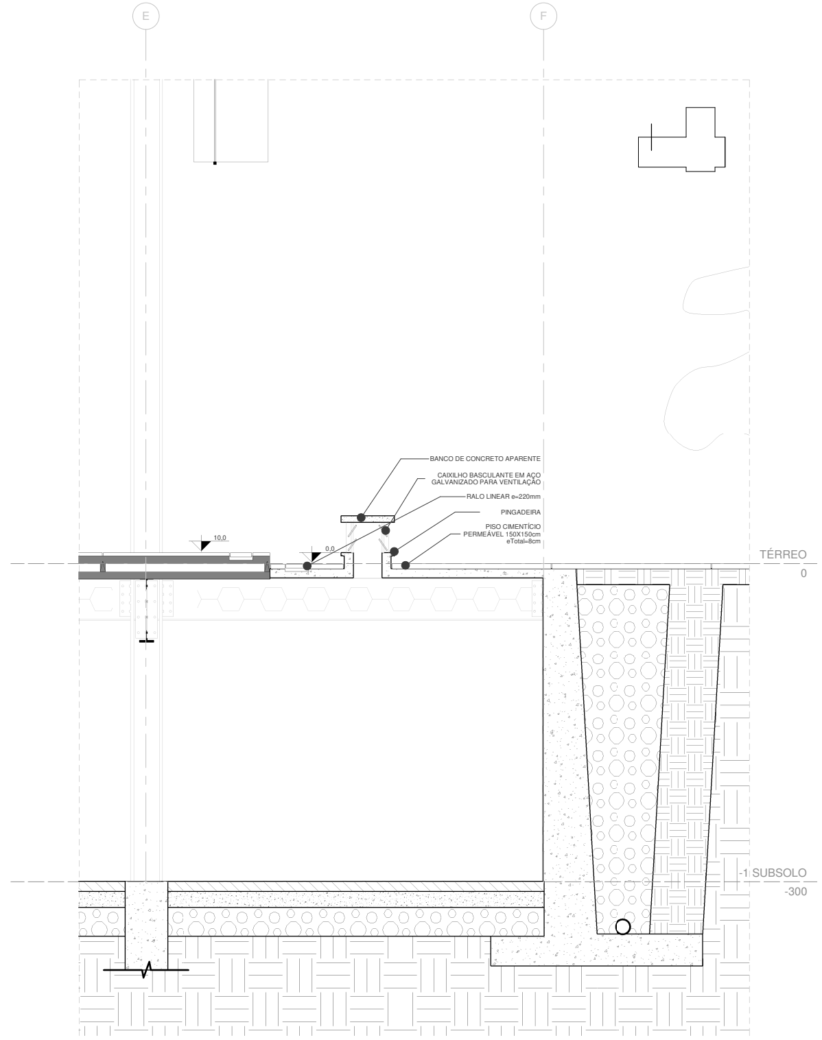
CORTE D2 - BANCO COM VENTILAÇÃO
