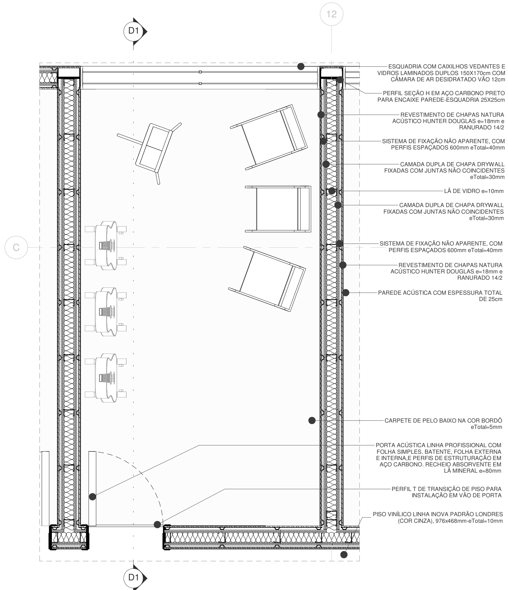
PLANTA BAIXA - SALA DE MÚSICA
