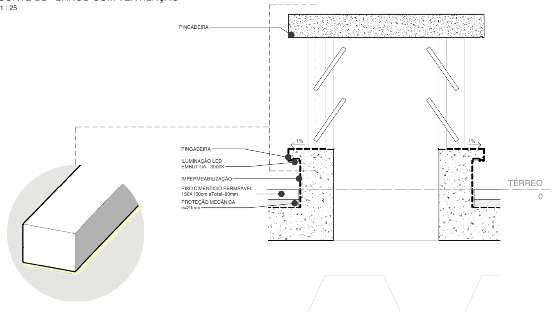
CORTE D2 - BANCO COM VENTILAÇÃO
