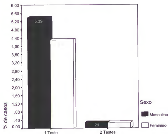
Gráfico 1 – Ocorrência de indivíduos classificados acima do percentil 98 nas variáveis da bateria de DTM.
