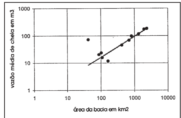
Figura 2. Vazão média de enchente, \bar{Q} função da área das bacias para postos na região metropolitana de Curitiba.
