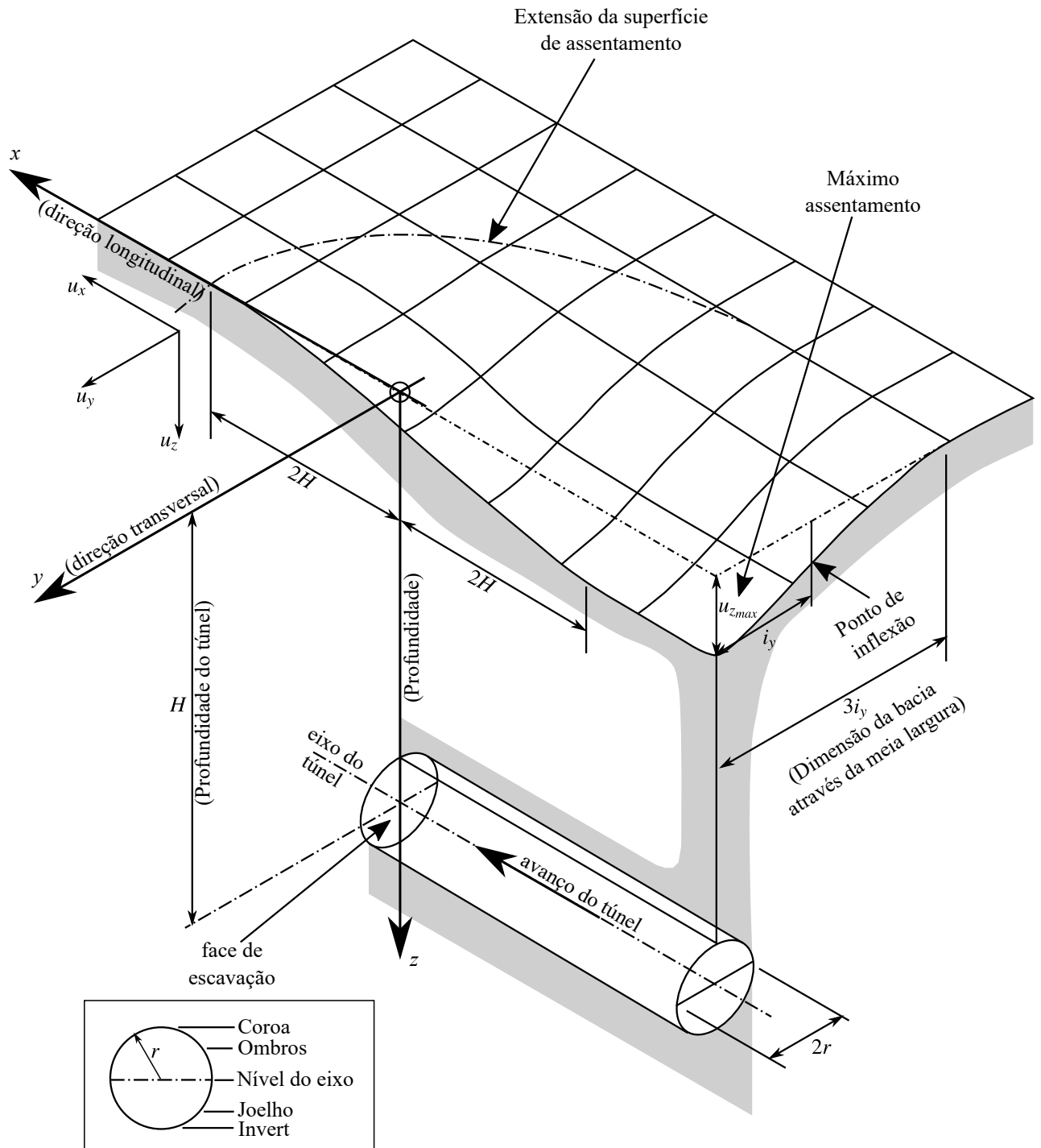
Figura 4.25 – Representação tridimensional da bacia de assentamento superficial durante a construção de um túnel superficial (adaptado de: Yeates e Geddes (1985) apud Rankin (1988, p. 80))
