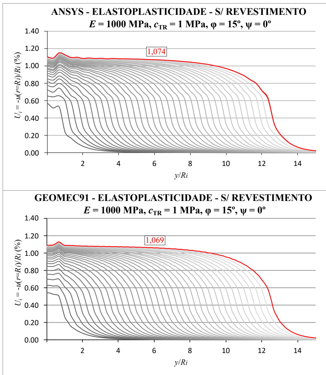
Figura 7.11 – Verificação solução numérica elastoelasticidade sem revestimento E = 1000 \text{ MPa} , c_i = c_p = c_r = \sqrt{3}/2 \text{ MPa} , \phi=15^\circ e \psi=0^\circ
