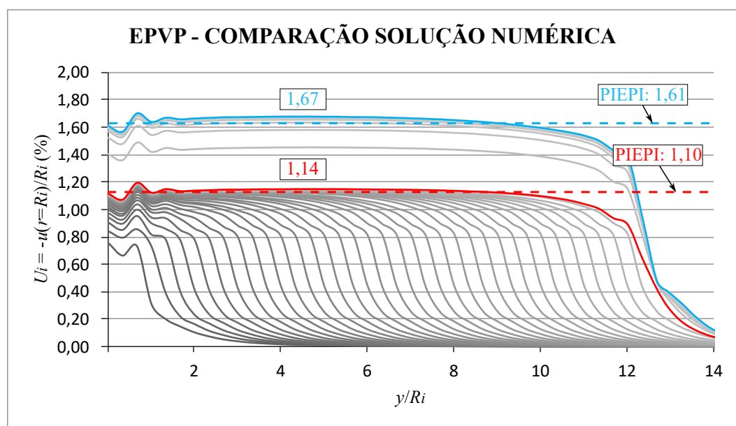
Figura 7.23 – Verificação com a solução de Piepi (1995) do modelo elastoplástico-viscoplástico com revestimento
