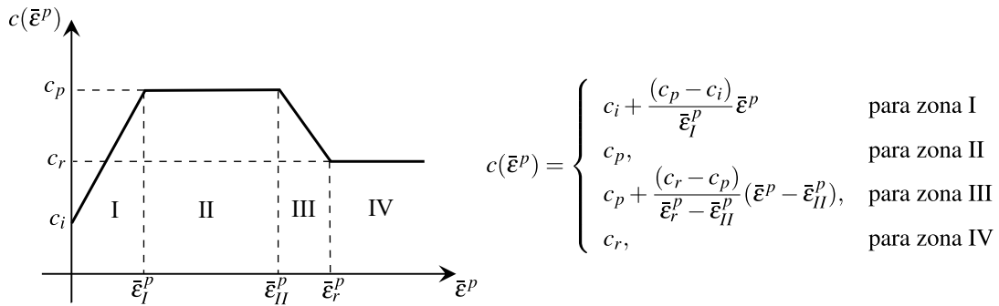
Figura 5.10 – Função linear definida por partes para representar o endurecimento/amolecimento através do parâmetro coesivo (adaptado de: Potts e Zdravkovic (1999, p. 158))
