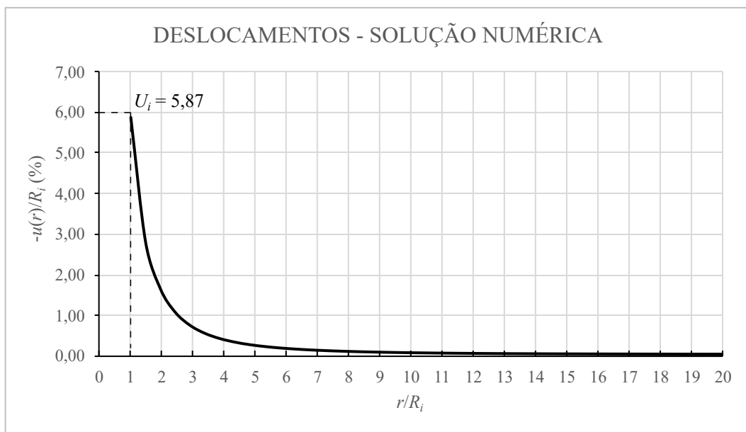
Figura 7.4 – Solução numérica considerando elastoplasticidade com endurecimento
