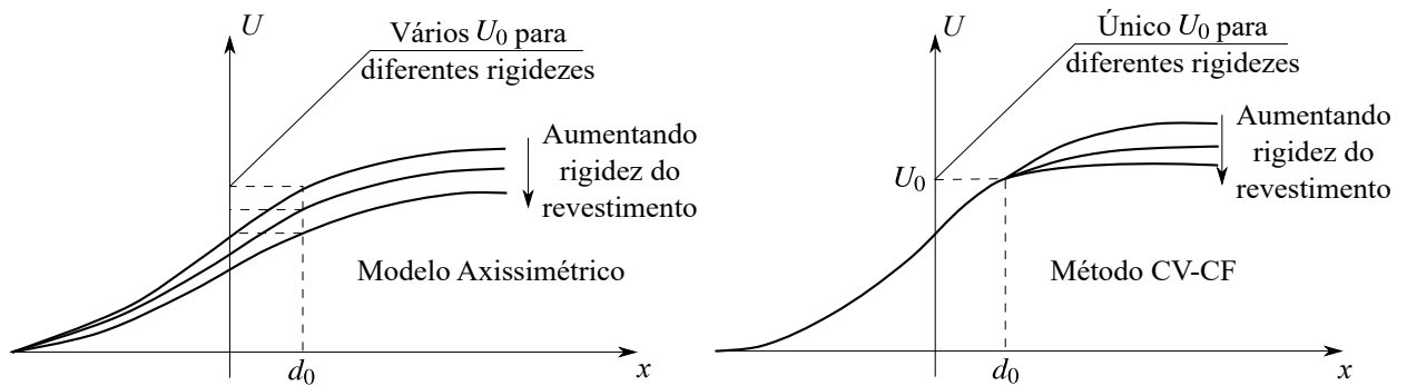
Figura 4.31 – Influência da rigidez do revestimento no perfil de convergências do túnel e no parâmetro U_0 (adaptado de: Bernaud e Rousset (1992, p. 13))
