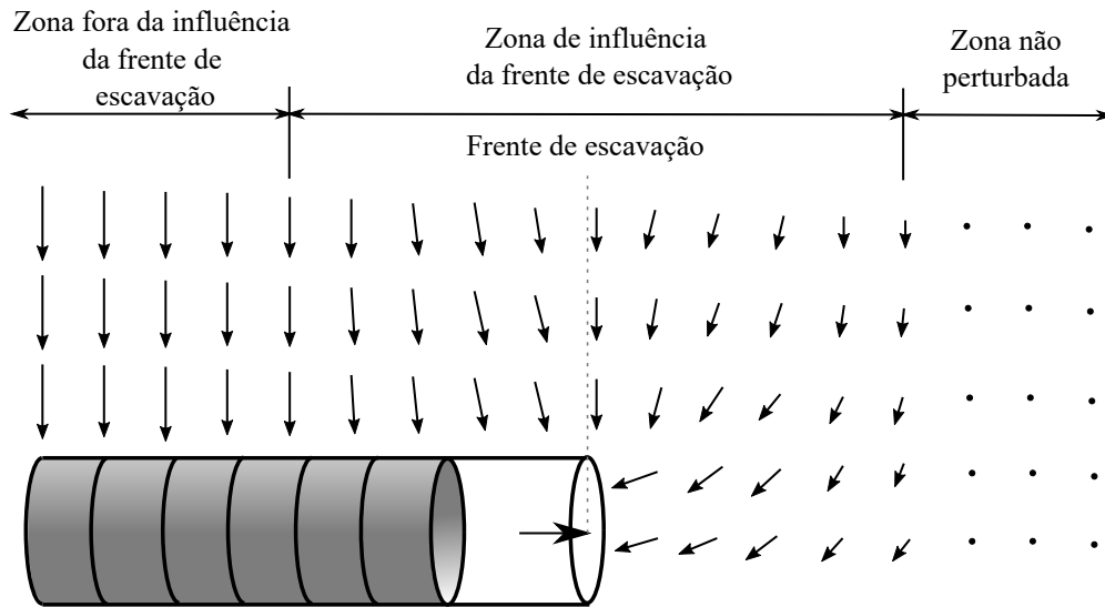
Figura 4.2 – Campo vetorial de deslocamentos no maciço durante a escavação de um túnel (adaptado de: França (2006, p. 12))
