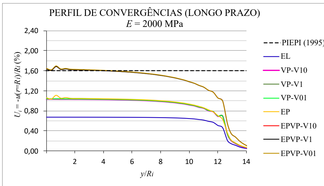
Figura 7.19 – Perfil de convergências no longo prazo para os diversos comportamentos implementados, considerando os parâmetros físicos do maciço de acordo com Piepi (1995) com E = 2000 \text{ MPa}
