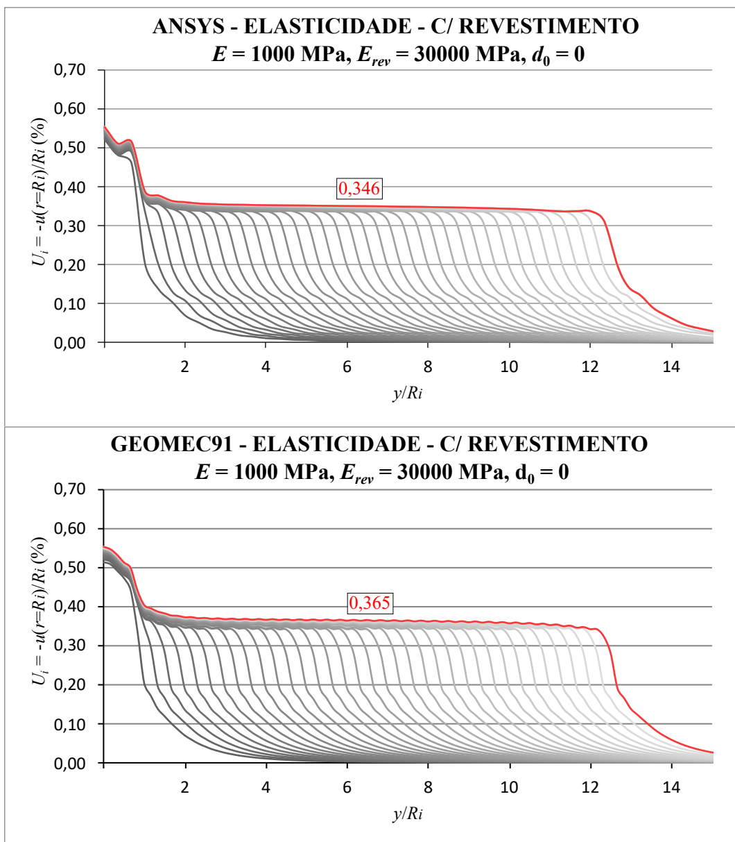
Figura 7.7 – Verificação solução numérica em elasticidade com revestimento - E = 1000 \text{ MPa}, E_{rev} = 30000 \text{ MPa}, d_0 = 0
