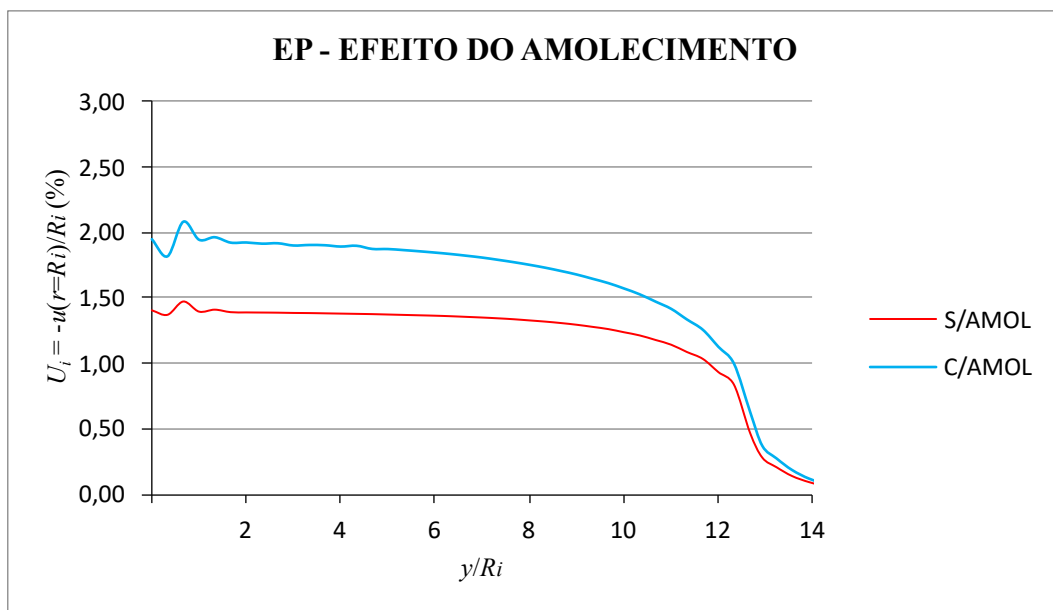
Figura 7.25 – Efeito do amolecimento no perfil de convergências para o caso elastoplástico
