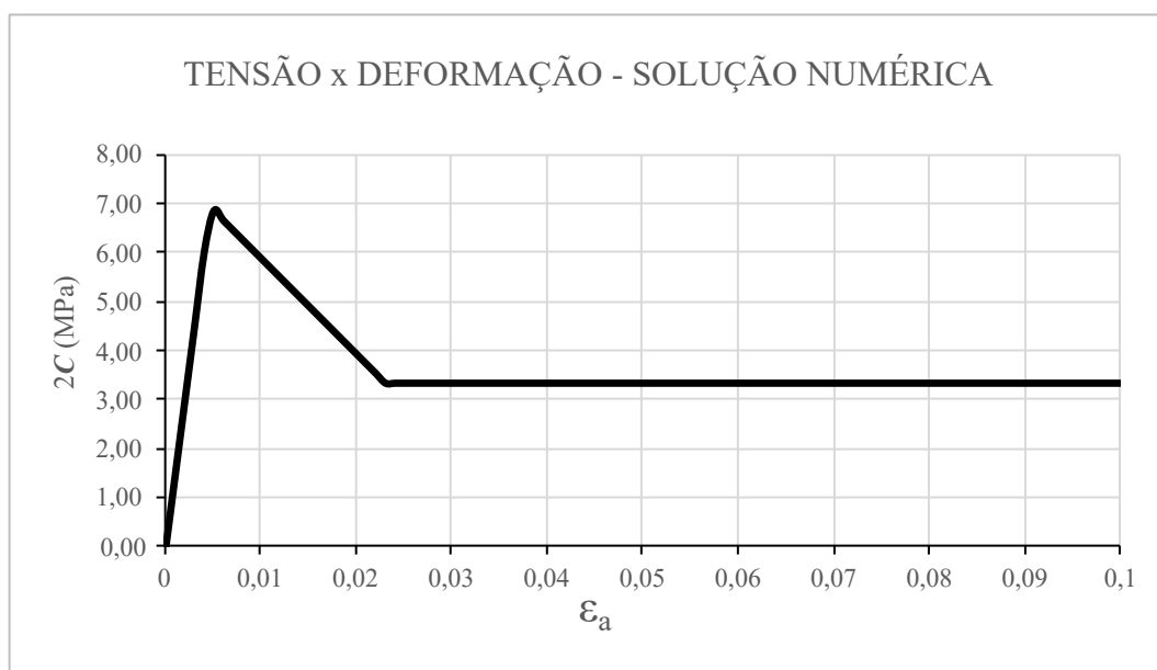
Figura 7.24 – Curva tensão versus deformação obtido pelo modelo com amolecimento
