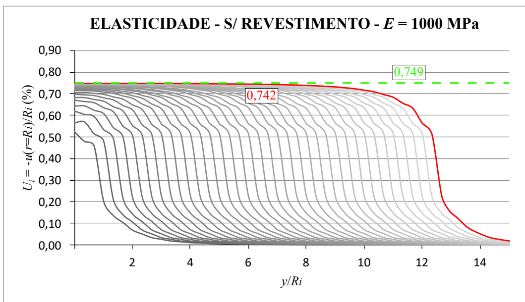
Figura 7.5 – Verificação solução numérica em elasticidade sem revestimento - E = 1000 MPa
