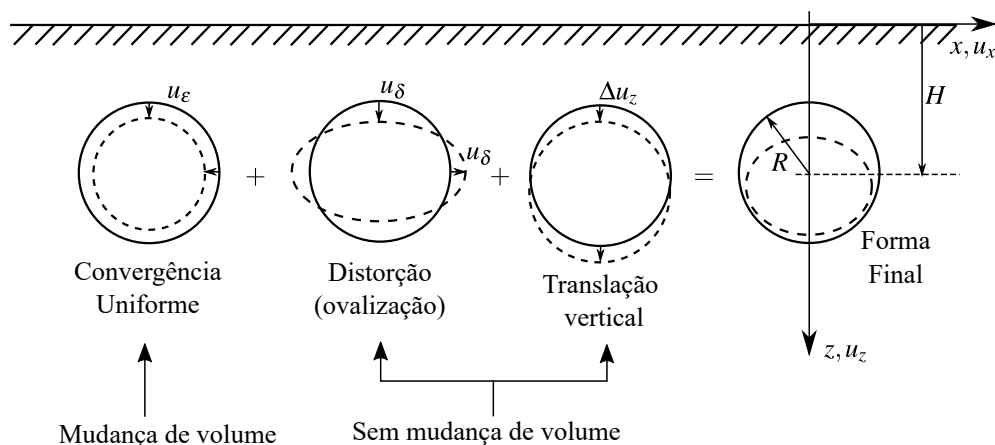
Figura 4.24 – Modos de deformações em túneis superficiais de seção circular (adaptado de: Pinto e Whittle (2014, p. 4))
