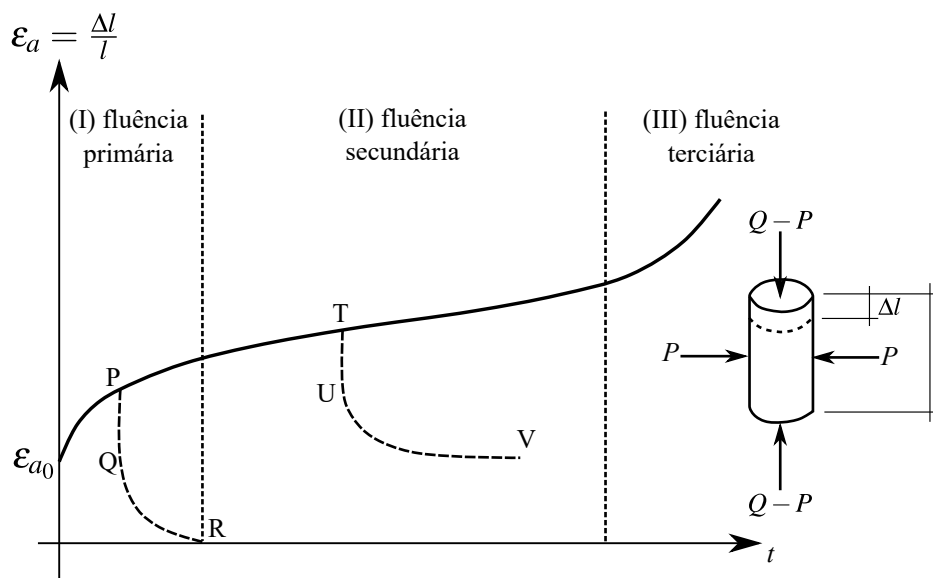
Figura 4.15 – Curva característica em um ensaio de fluência com os três estágios de comportamento (adaptado de: Costa (1984, p. 107))
