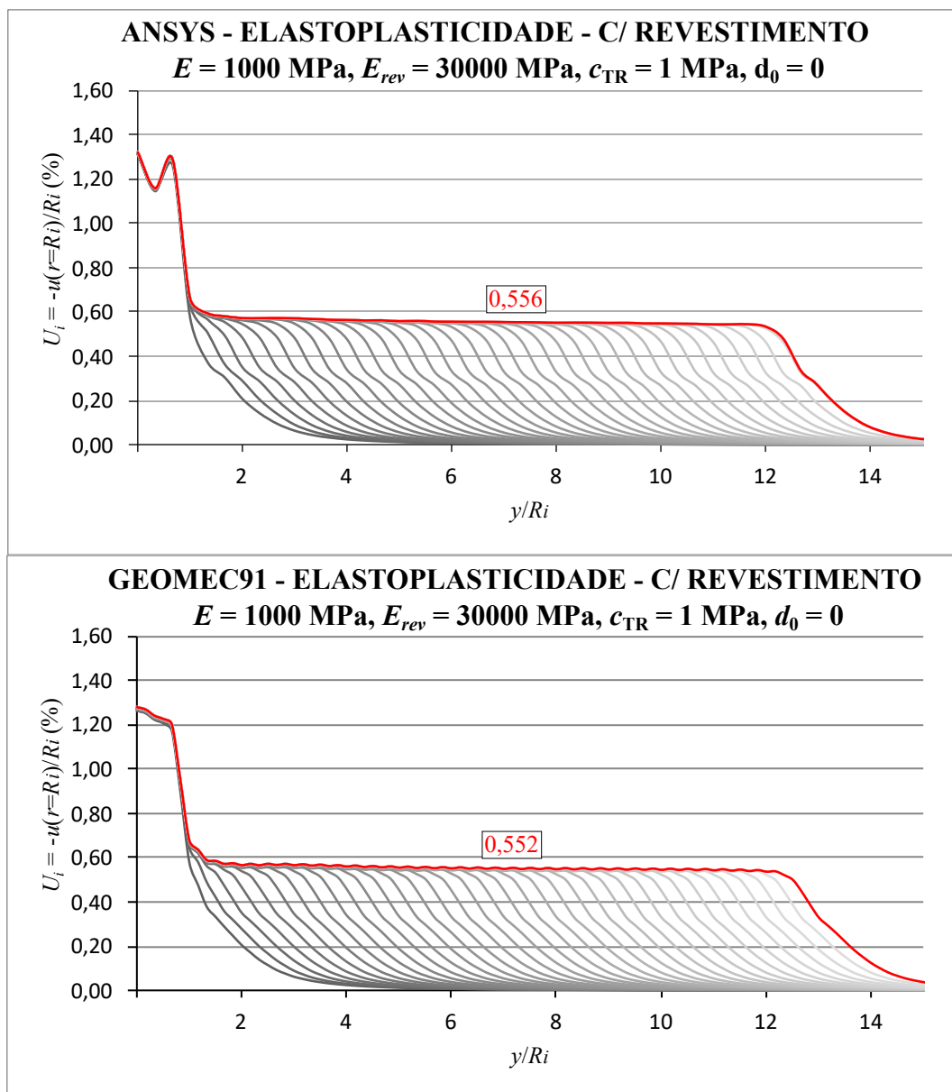
Figura 7.12 – Verificação solução numérica em elastoelasticidade com revestimento - E = 1000 \text{ MPa} , E_{rev} = 30000 \text{ MPa} , d_0 = 0 , c_i = c_p = c_r = \sqrt{3}/2 \text{ MPa}
