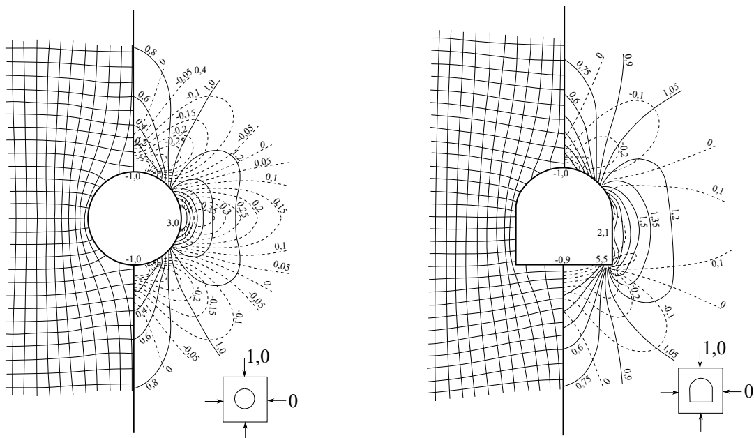
Figura 4.22 – Trajetória das tensões principais e linhas de isotensão da maior e menor tensão principal para seção circular (à esquerda) e ferradura (à direita) considerando K = 0 (adaptado de: Hoek e Brown (1980, p. 468,483))
