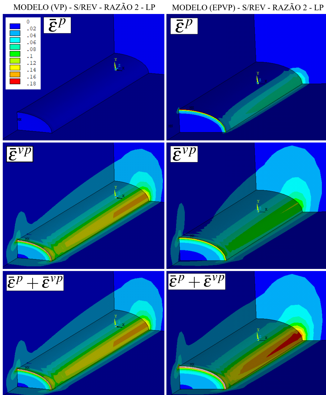
Figura 7.35 – Campo de deformações equivalentes para o modelo (VP) e (EPVP), sem revestimento, com razão de aspecto 2 e no longo prazo
