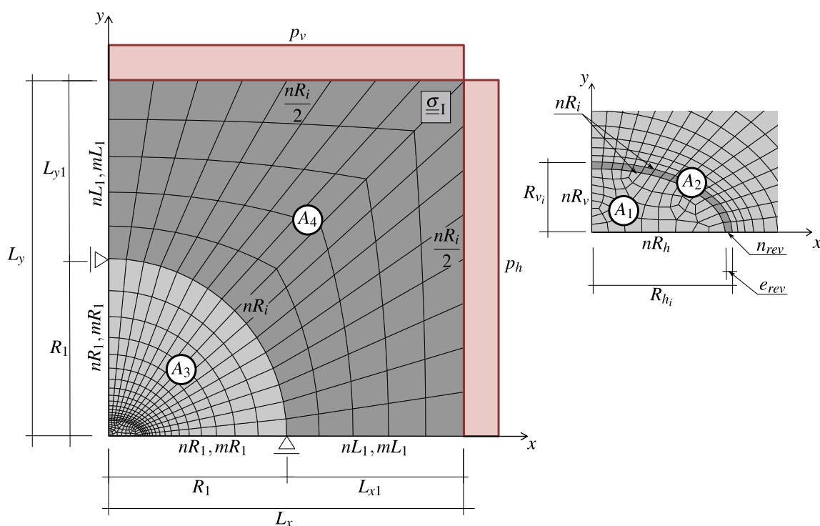
Figura 6.12 – Domínio, parâmetros geométricos, condições de contorno e malha para o modelo em estado plano de deformações
