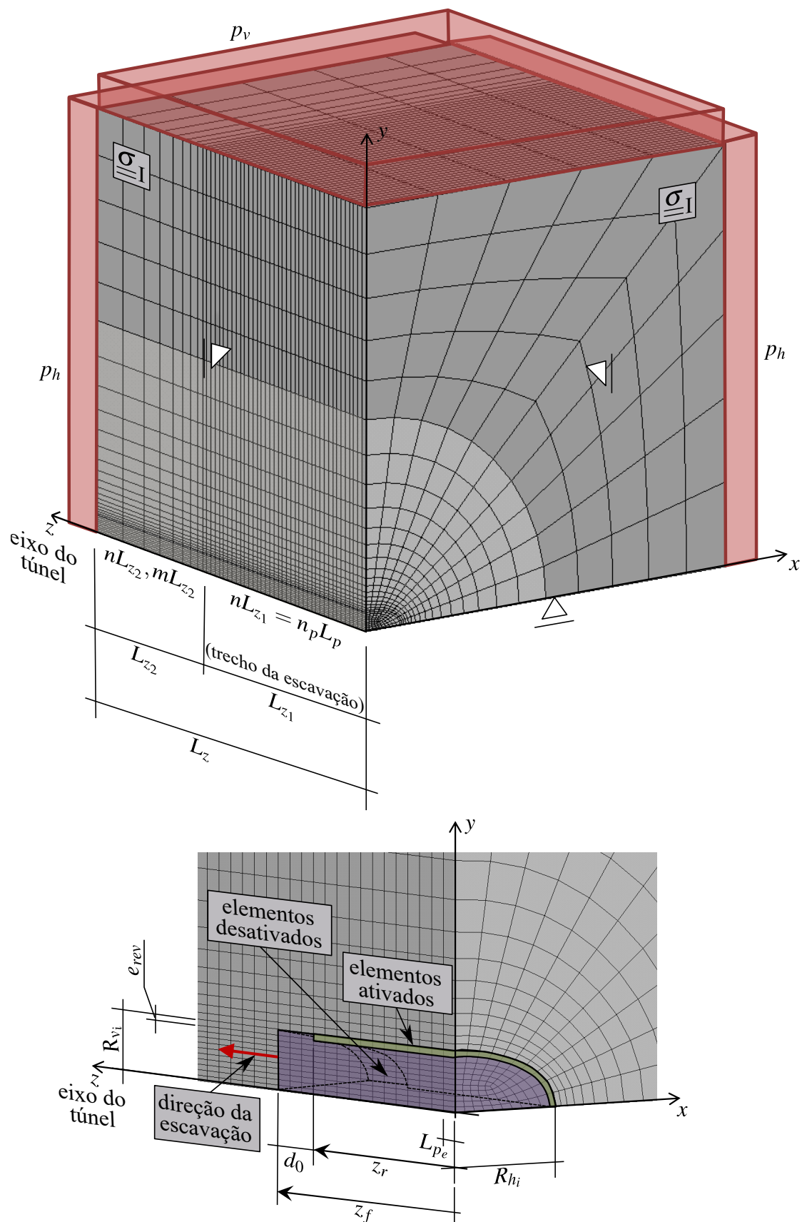
Figura 6.13 – Domínio, parâmetros geométricos, condições de contorno e malha para o modelo tridimensional
