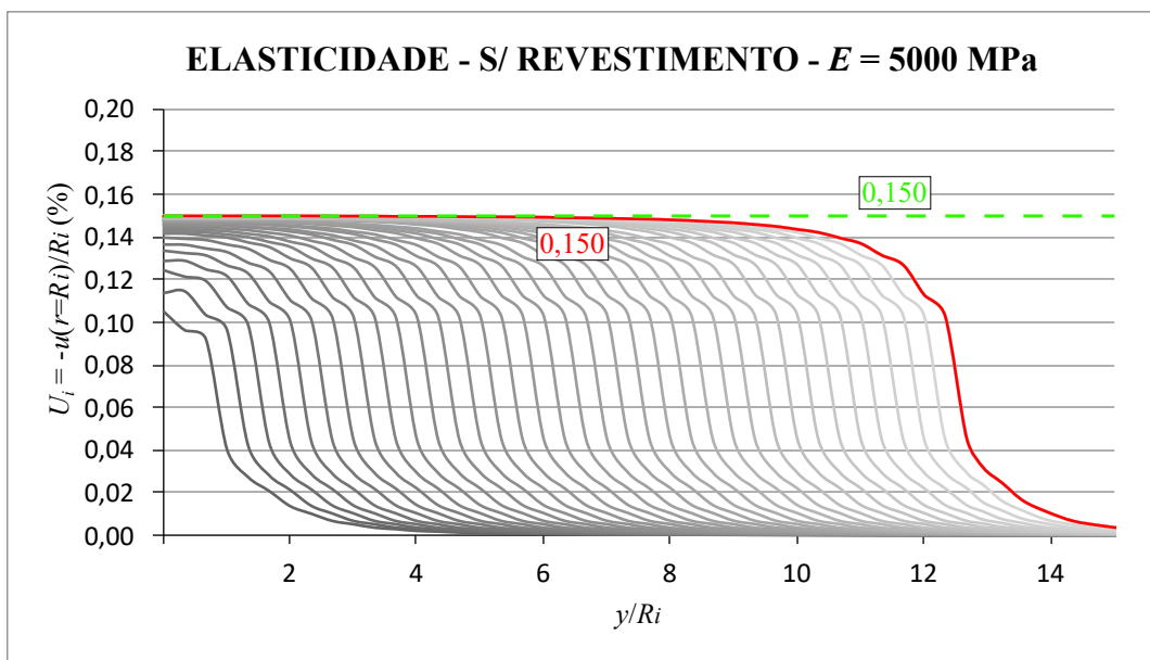
Figura 7.6 – Verificação solução numérica em elasticidade sem revestimento - E = 5000 MPa
