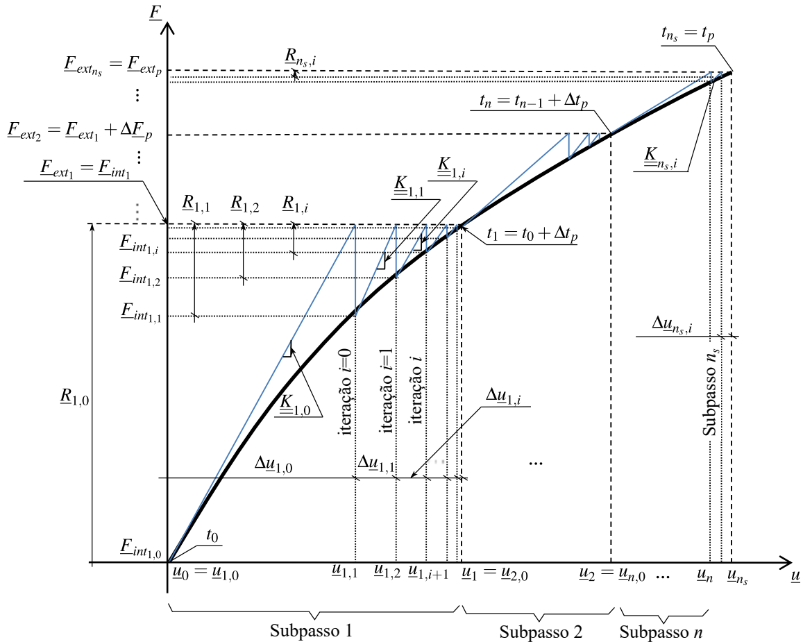
Figura 6.5 – Ilustração das iterações do método de Newton-Raphson (adaptado de: Chen e Han (1988, p. 301))
