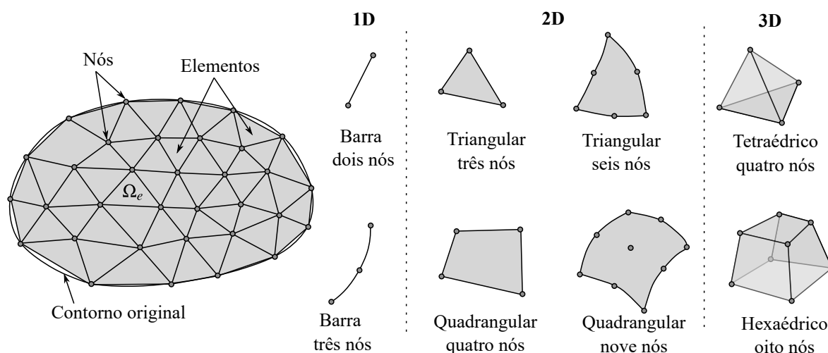
Figura 6.1 – Discretização de um domínio genérico em elementos finitos (adaptado de: de Souza (2003, p. 1-2))
