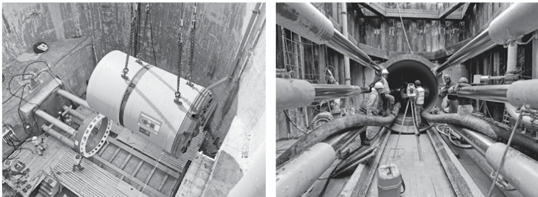
Figura 3.9 – À esquerda: vista de cima de um poço de macacos hidráulicos com a descida da TBM; à direita: vista frontal do túnel (fonte: Chapman, Metje e Stärk (2018, p. 227))
