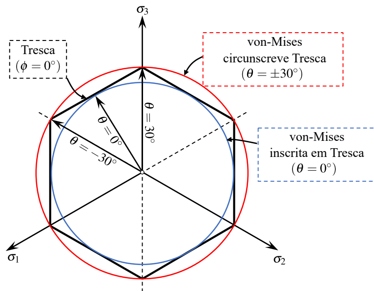
Figura 5.7 – Representação no plano desviador da aproximação da superfície de Tresca pela superfície de von-Mises (adaptado de: de SOUZA NETO; PERI; OWEN, 2008, p. 159, 164)
