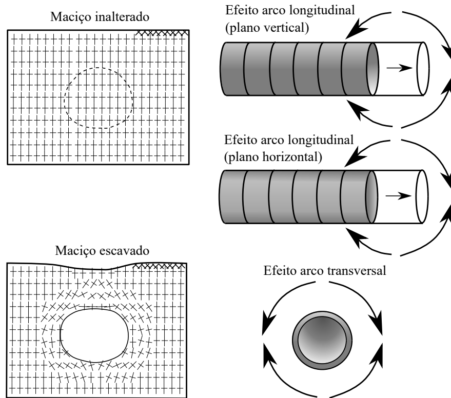
Figura 4.1 – Ilustração do arqueamento das tensões principais (adaptado de: França (2006, p. 10-11))
