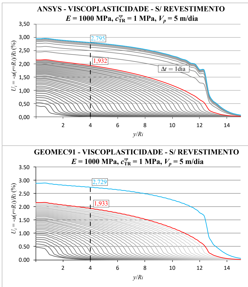
Figura 7.13 – Verificação solução numérica em elastoplasticidade com revestimento - E = 1000 \text{ MPa} , c^{vp} = \sqrt{3}/2 \text{ MPa} , V_p = 5 \text{ m/dia}
