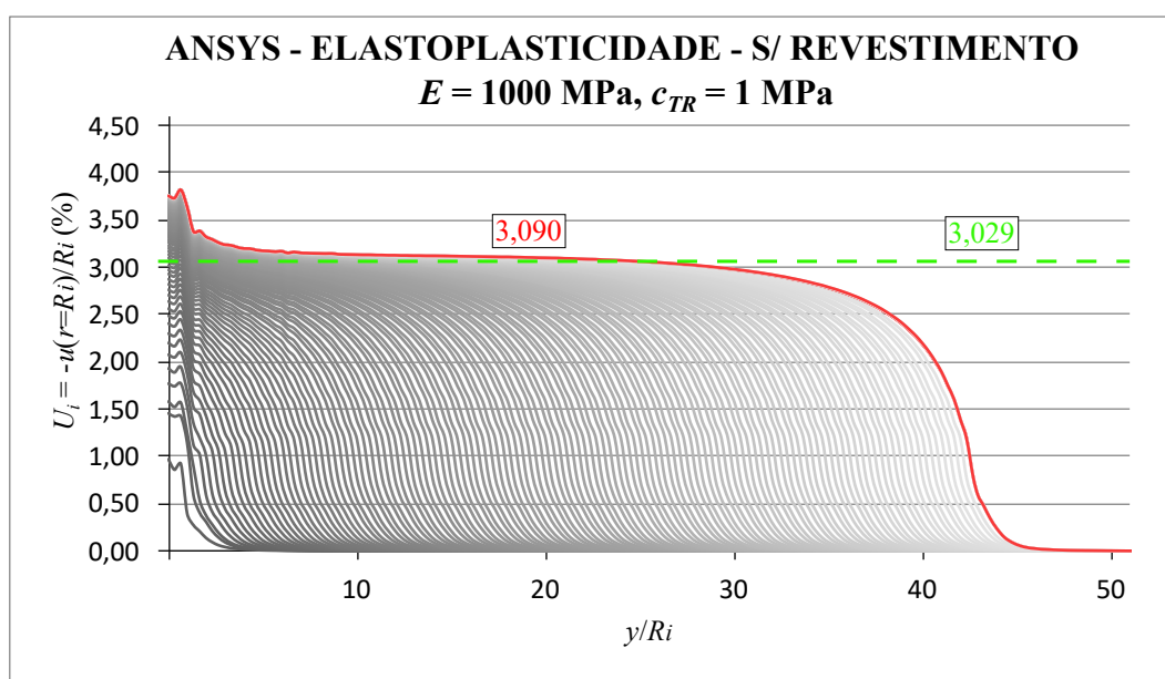
Figura 7.9 – Verificação solução numérica em elastoplasticidade sem revestimento - E = 1000 MPa, c_i = c_p = c_r = \sqrt{3}/2 MPa
