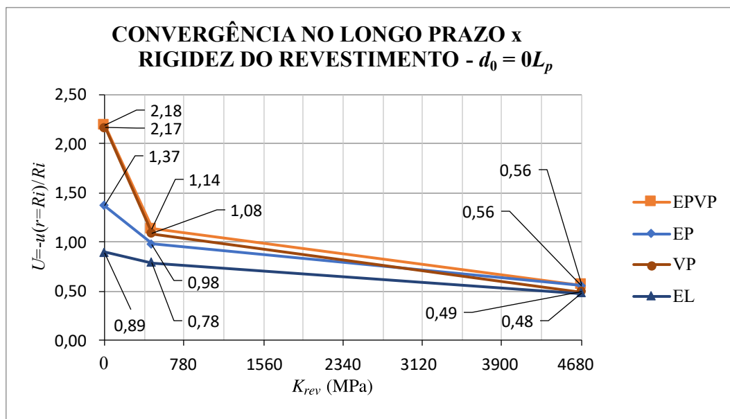
Figura 7.28 – Convergência no longo prazo versus módulo de elasticidade do revestimento para uma distância não revestida d_0 = 0
