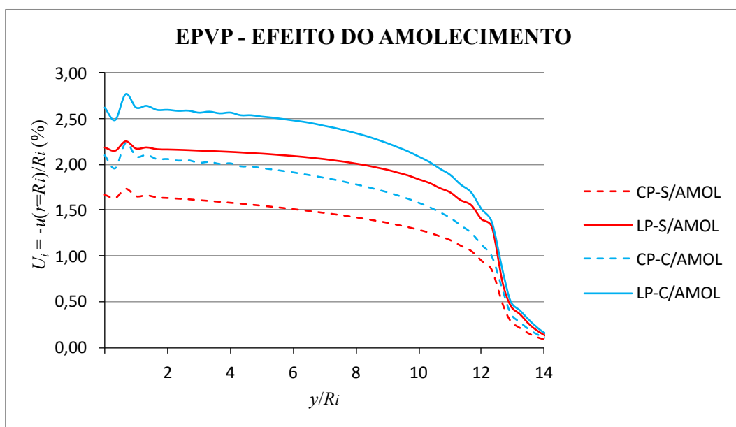
Figura 7.26 – Efeito do amolecimento no perfil de convergências para o caso elastoplástico-viscoplástico
