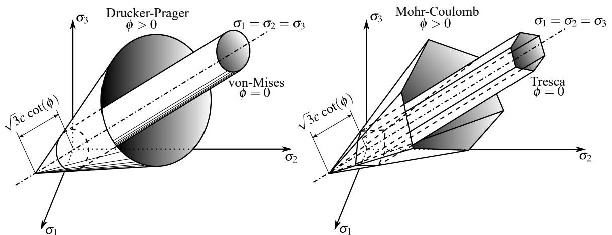
Figura 5.5 – Funções de escoamento de a) Drucker-Prager e b) Mohr-Coulomb (adaptado de: Zienkiewicz e Corneau (1974, p. 824))
