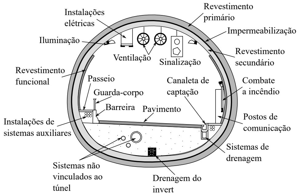
Figura 3.11 – Ilustração do revestimento e elementos internos de um túnel rodoviário (adaptado de: DEPARTAMENTO DE ESTRADAS E RODAGEM (SÃO PAULO) (2005, p. 20))
