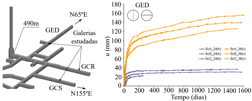
Figura 4.11 – Evolução do fechamento da seção (convergência) na galeria GED do laboratório Meuse/Haute-Marne (adaptado de: Guayacán-Carrillo et al. (2016, p. 103))
