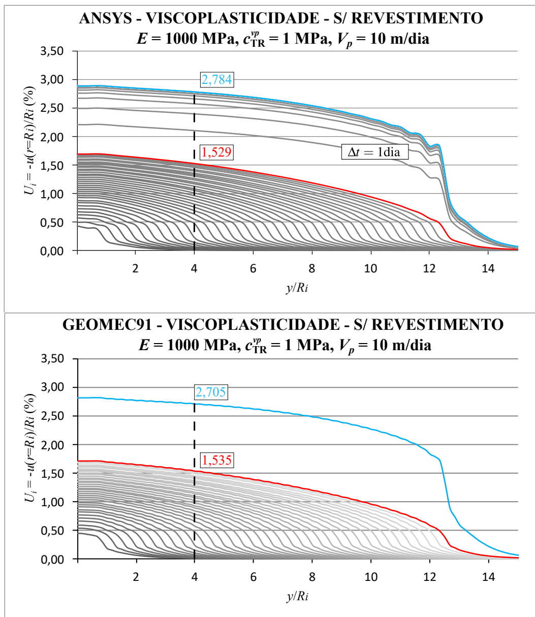
Figura 7.14 – Verificação solução numérica em viscoplasticidade com revestimento - E = 1000 \text{ MPa} , c^{vp} = \sqrt{3}/2 \text{ MPa} , V_p = 10 \text{ m/dia}
