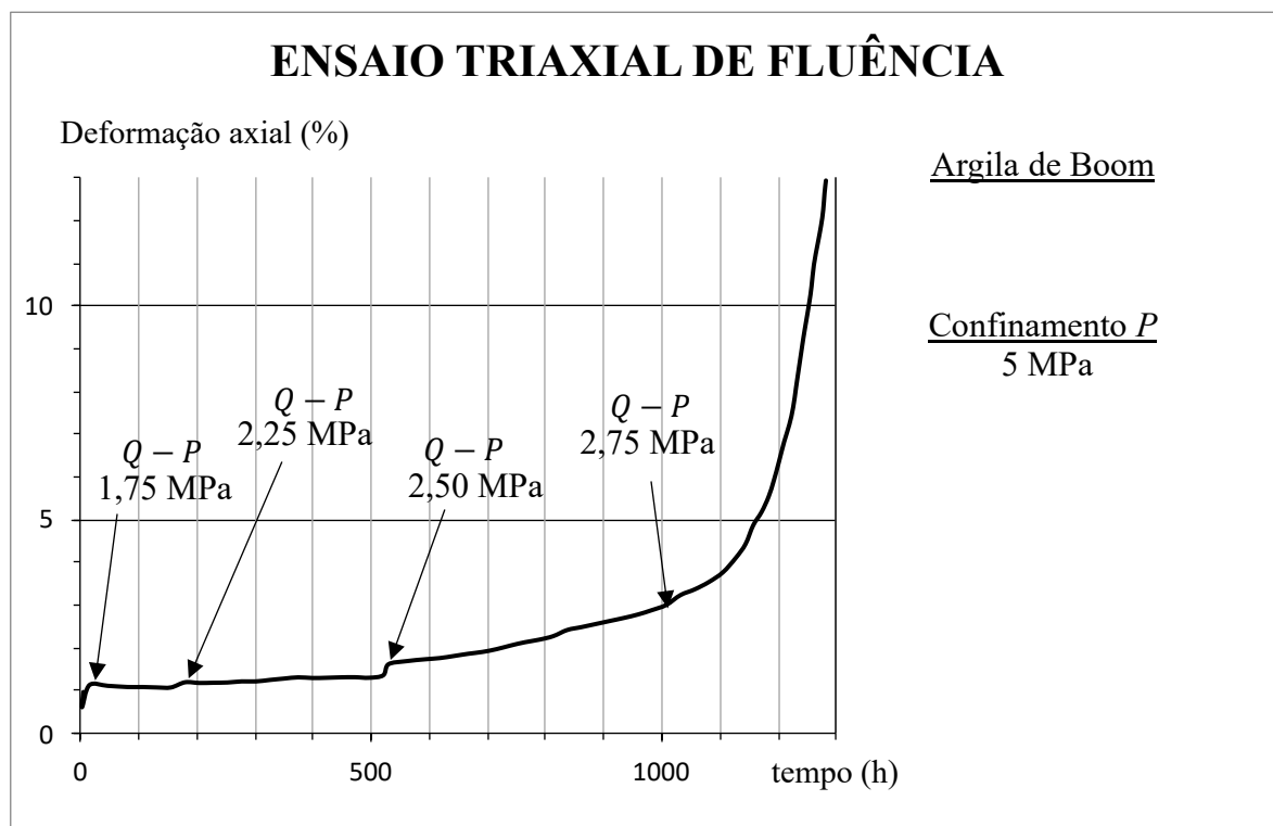
Figura 4.16 – Ensaio triaxial de fluência da Argila de Boom (adaptado de: Rousset (1988, p. 42))
