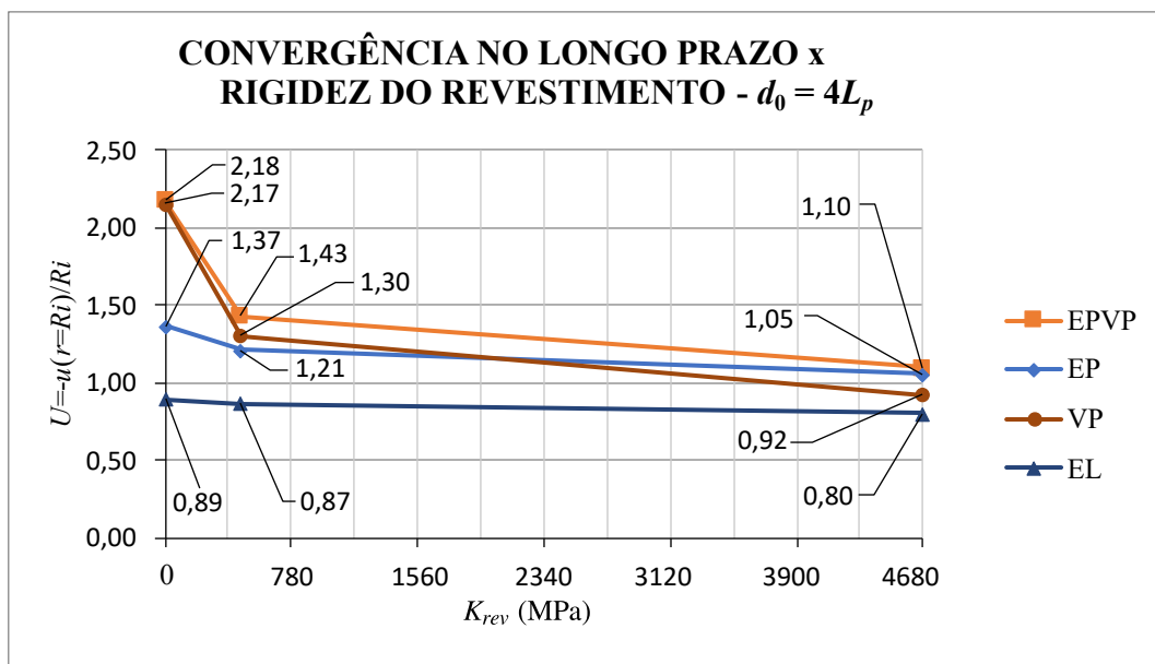
Figura 7.30 – Convergência no longo prazo versus módulo de elasticidade do revestimento para uma distância não revestida d_0 = 4L_p
