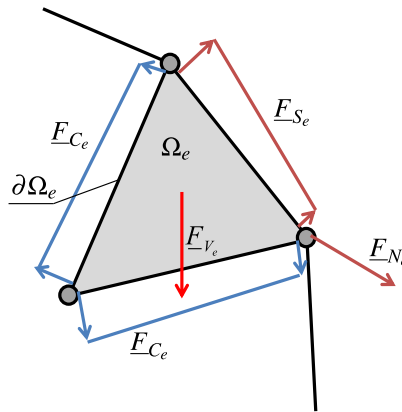
Figura 6.2 – Diagrama de corpo livre de um elemento finito (adaptado de: Lizarza (2011, p. 19))
