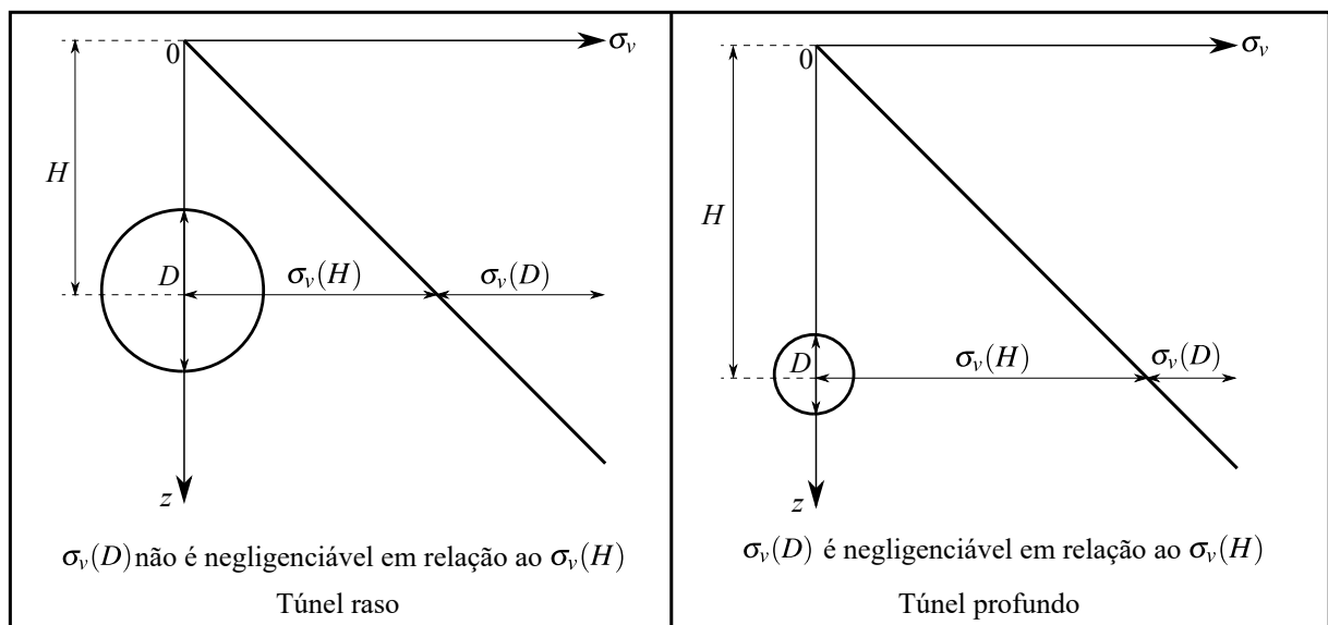
Figura 4.21 – Princípio para se desconsiderar a variação da tensão vertical na região próxima ao túnel (adaptado de: Benamar (1996, p. 8))
