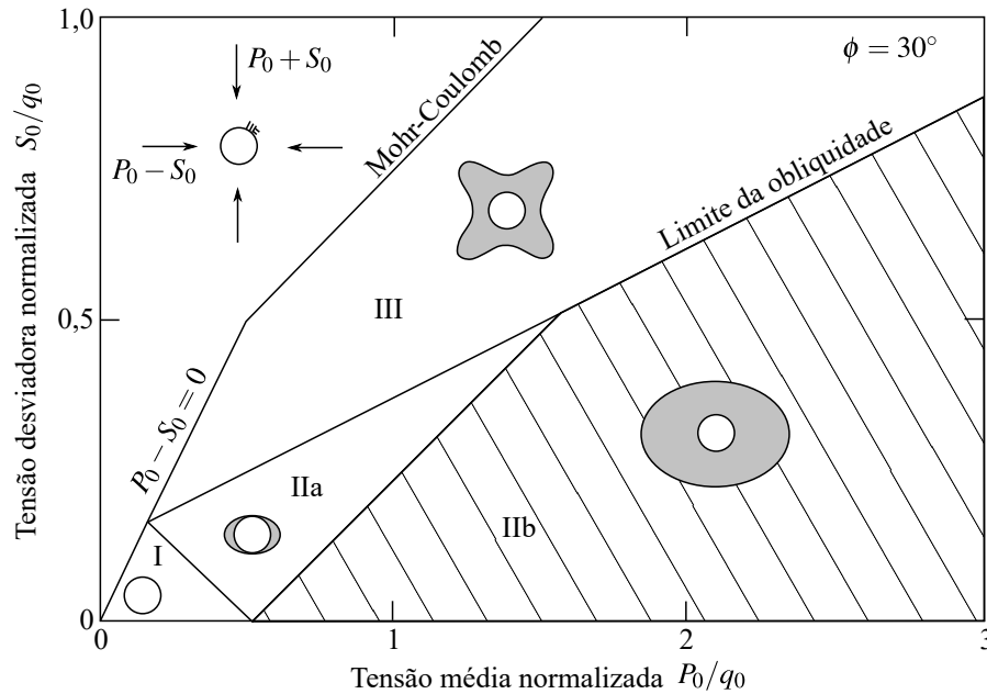
Figura 4.23 – Relação entre o estado de tensões iniciais e os modos de falha, onde q_0 é a resistência à compressão do maciço (adaptado de: Detournay e St. John (1988, p. 121))
