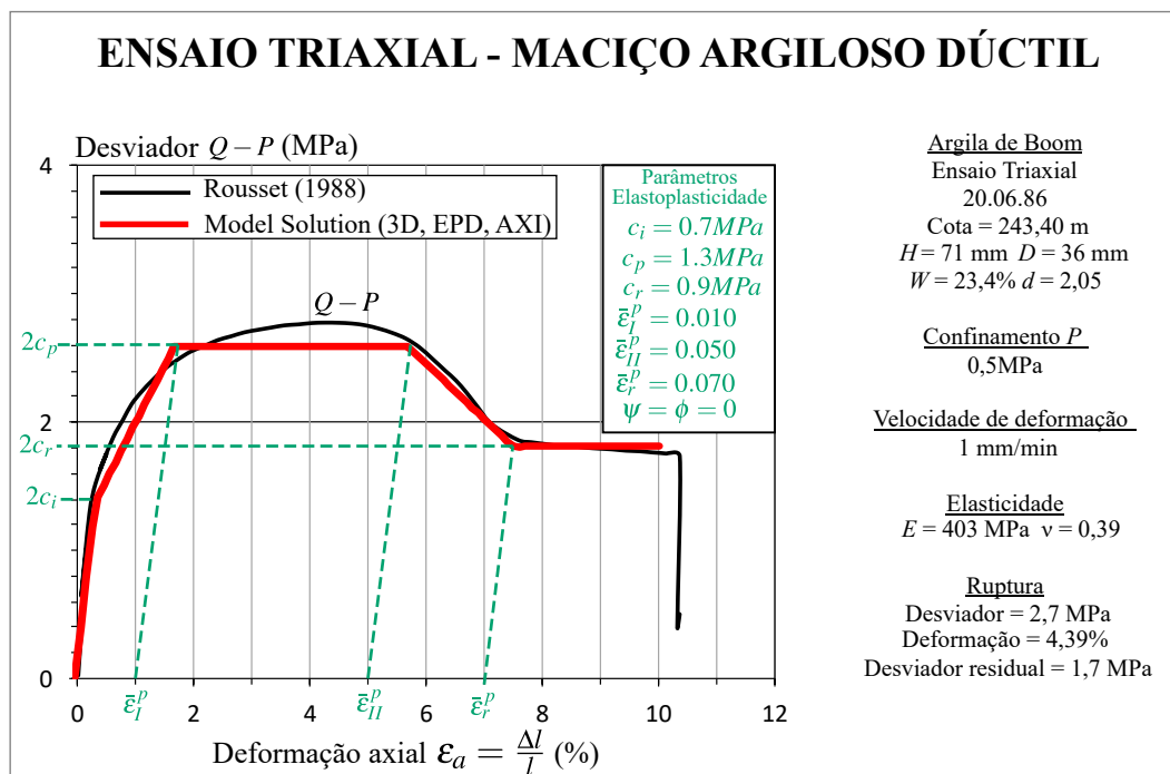
Figura 7.2 – Validação da lei de endurecimento/amolecimento
