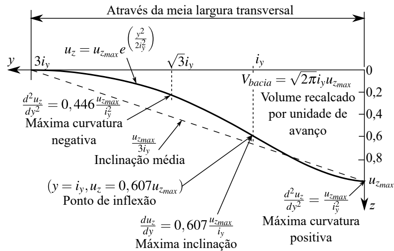
Figura 4.26 – Perfil idealizado de assentamento transversal com distribuição normal (adaptado de: O'Reilly e New (1982) apud Rankin (1988, p. 80))
