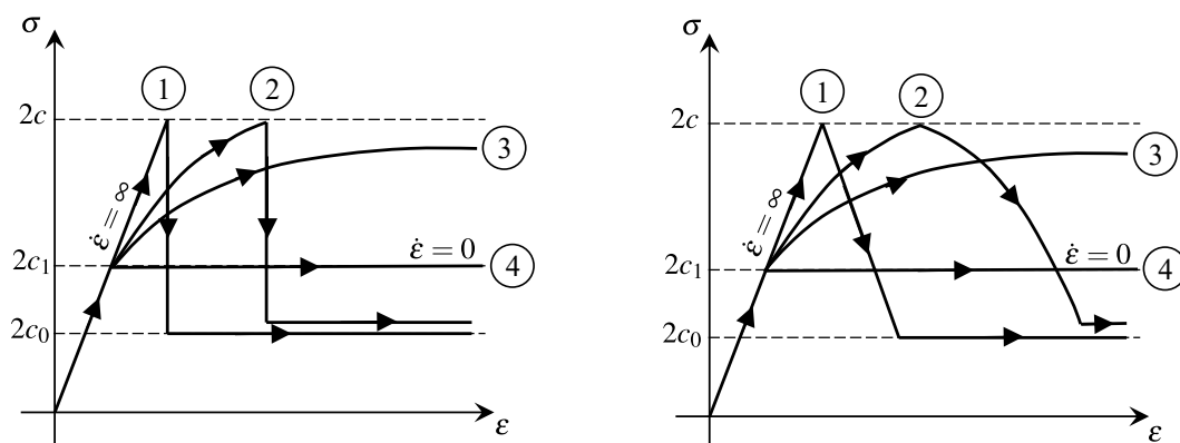
Figura 5.14 – Resposta do sistema a uma solicitação \dot{\epsilon} = \text{const.} Ruptura frágil (à esquerda) e ruptura dúctil (à direita) (adaptado de: Rousset (1988, p. 221))
