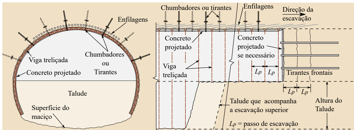
Figura 3.12 – Ilustração de alguns elementos de pré-suporte e revestimento (adaptado de: FEDERAL HIGHWAY ADMINISTRATION (U.S.) (2009, p. 9-14))
