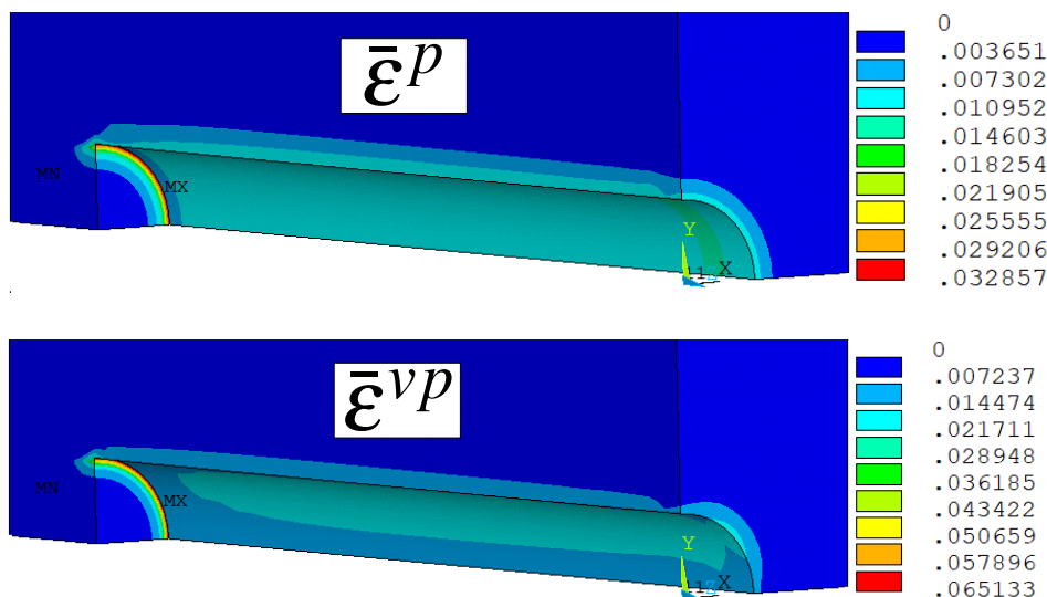
Figura 7.21 – Campo de deformações plásticas e viscosas no longo prazo para o caso elastoplástico-viscoplástico com E = 1500 MPa e V_p = 0,1 m/dia
