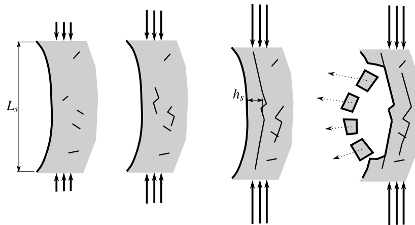
Figura 4.8 – Mecanismo de ruptura por Spalling de um comprimento L_s junto à seção do túnel: detalhamento do crescimento das fissuras e flambagem de uma profundidade h_s da rocha no contorno da seção (adaptado de: Germanovich e Dyskin (2000, p. 267))
