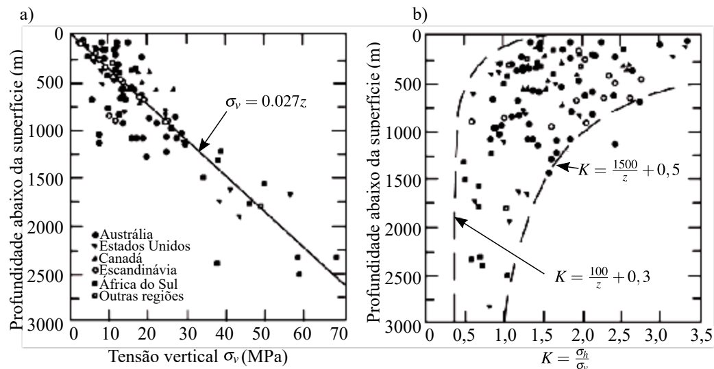
Figura 4.20 – a) tensões verticais e b) razão entre a tensão horizontal e vertical (coeficiente de empuxo K ) (adaptado de: Hoek e Brown (1980, p. 99-100))
