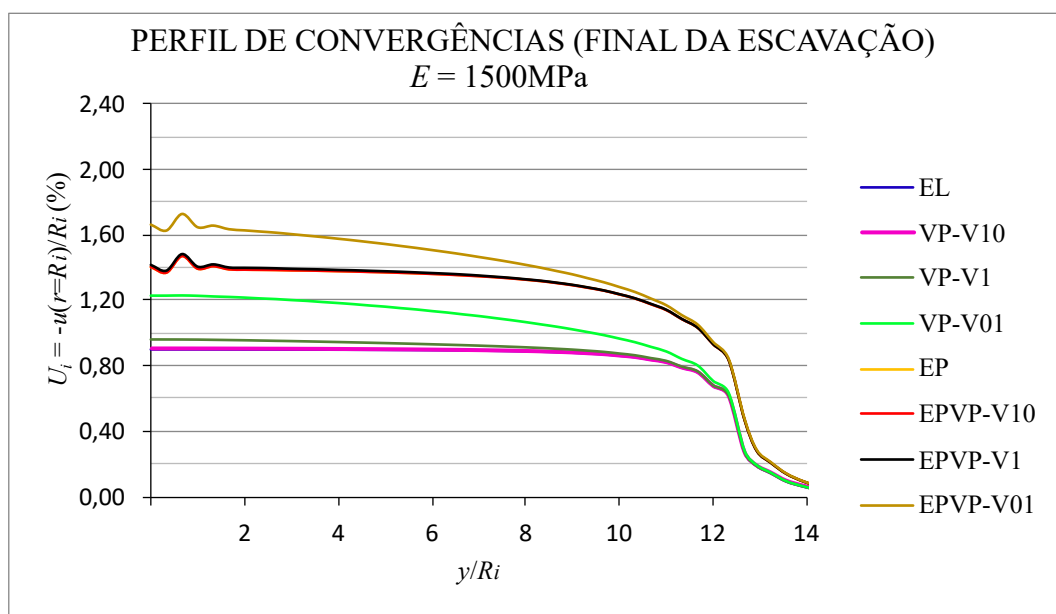
Figura 7.16 – Perfis de convergências no final da escavação para os diversos comportamentos implementados, considerando os parâmetros físicos do maciço de acordo com Piepi (1995) com E = 1500\text{ MPa}
