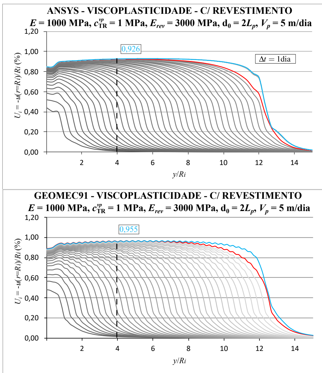
Figura 7.15 – Verificação solução numérica em viscoplasticidade com revestimento - E = 1000 MPa, c^{vp} = \sqrt{3}/2 MPa, E_{rev} = 3000 MPa, d_0 = 2L_p , V_p = 5 m/dia
