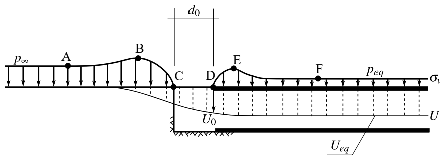
Figura 4.27 – Perfil de tensões verticais e de convergências ao longo de uma linha longitudinal situada no teto do túnel (adaptado de: Eisenstein, Heinz e Negro (1984) apud Couto (2011, p. 41))
