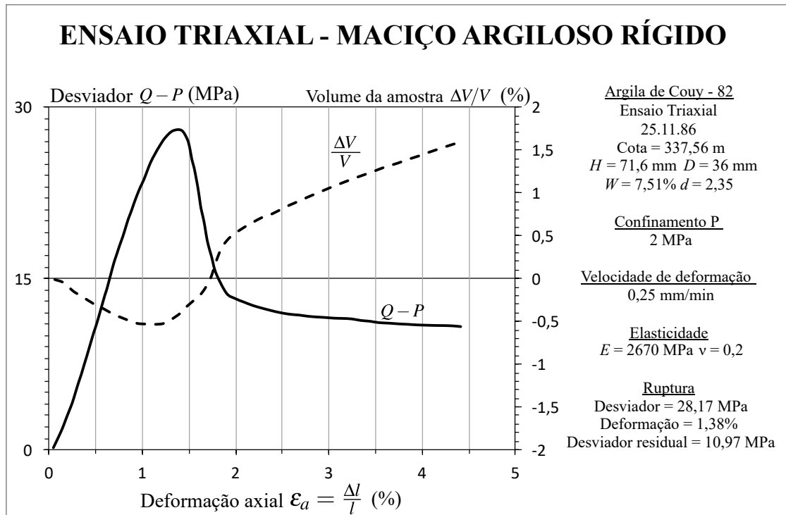
Figura 4.12 – Ensaio triaxial com medição da variação do volume para o caso de um maciço argiloso rígido (adaptado de: Rousset (1988, p. 35))
