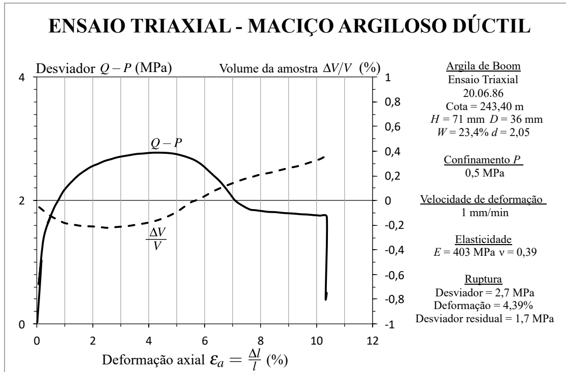
Figura 4.13 – Ensaio triaxial com medição da variação do volume para o caso de um maciço argiloso dúctil (adaptado de: Rousset (1988, p. 35))
