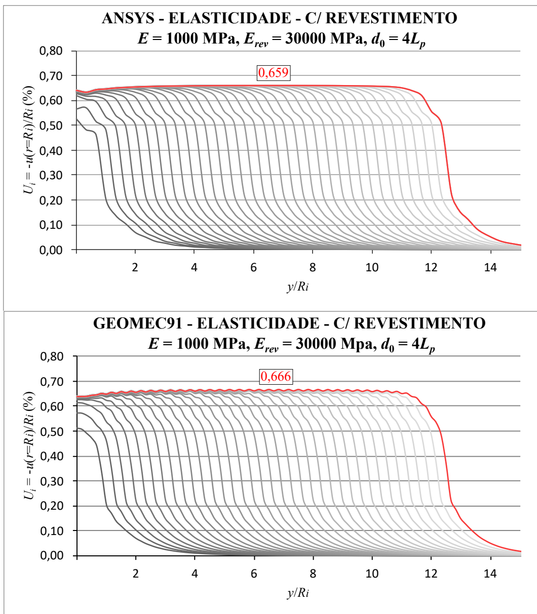
Figura 7.8 – Verificação solução numérica em elasticidade com revestimento - E = 1000 \text{ MPa} , E_{rev} = 30000 \text{ MPa} , d_0 = 4L_p
