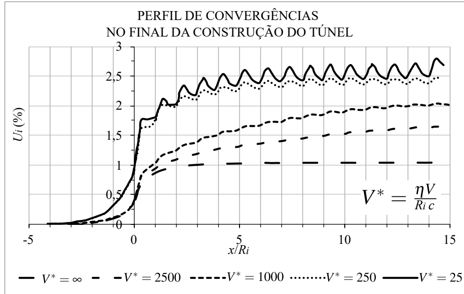
Figura 4.28 – Perfil de convergência em função da velocidade adimensional de avanço no final da construção do túnel (adaptado de: Bernaud (1991, p. 214))
