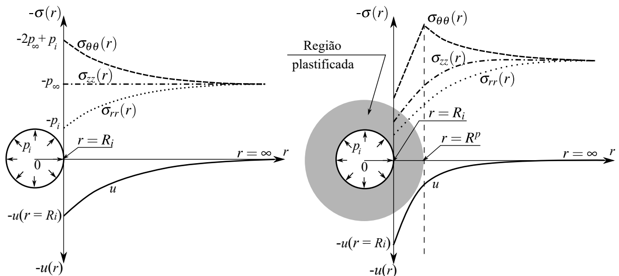
Figura 4.14 – Deslocamentos e tensões no entorno de um maciço submetido à pressão geostática-hidroestática p_\infty e pressão interna p_i no interior da seção do túnel. À esquerda, maciço elástico e à direita, elastoplástico (elaborado pelo autor)
