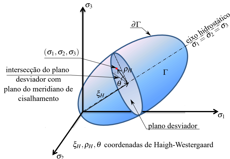
Figura 5.4 – Domínio genérico plasticamente admissível \Gamma no espaço das tensões principais
