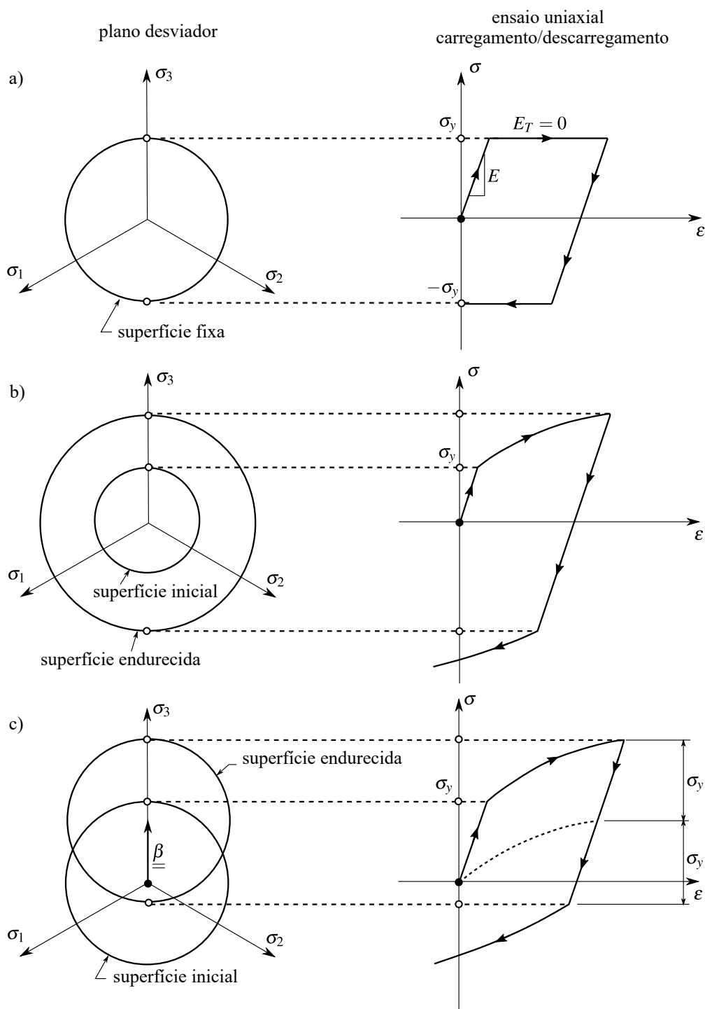
Figura 5.9 – Representação dos tipos de endurecimento no plano desviador e na curva tensão-deformação: a) elastoplasticidade perfeita, b) endurecimento isotrópico e c) endurecimento cinemático (adaptado de: de SOUZA NETO; PERI; OWEN, 2008, p. 178, 179, 186)
