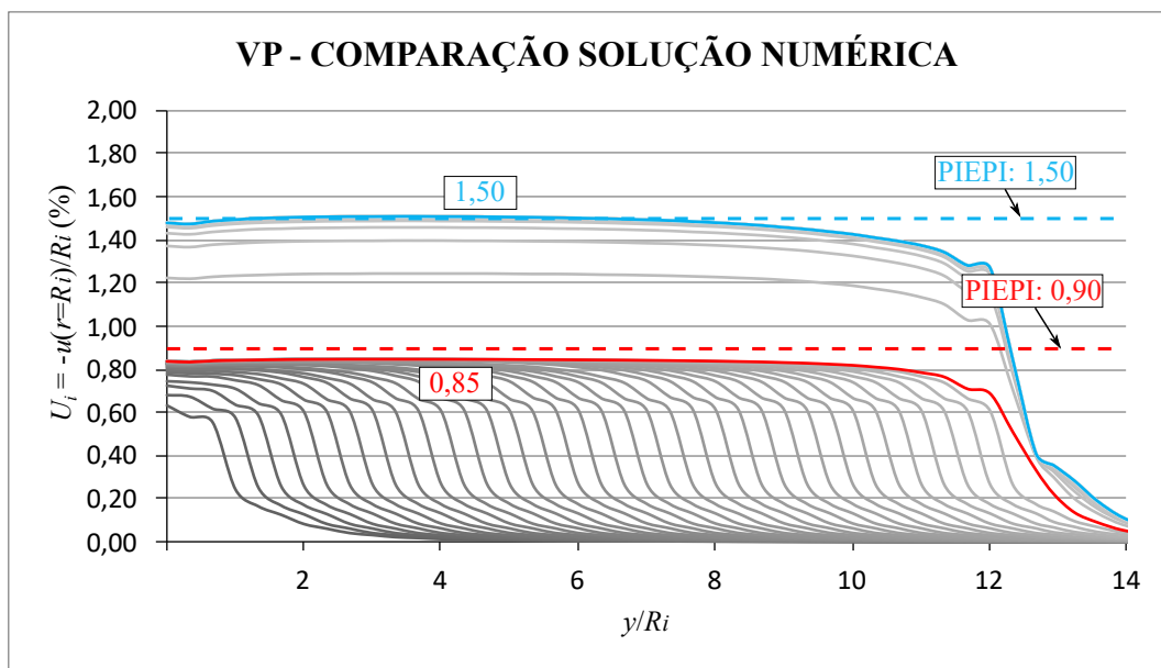
Figura 7.22 – Verificação com a solução de Piepi (1995) do modelo viscoplástico com revestimento
