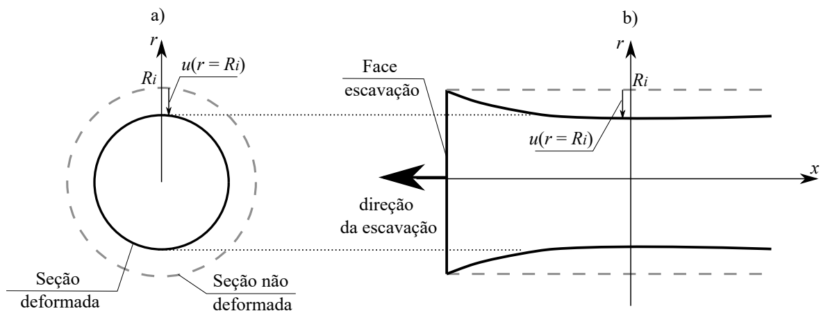
Figura 4.3 – Ilustração das medidas geométricas que compõem a convergência de uma seção circular: a) corte transversal, b) corte longitudinal (elaborado pelo autor)
