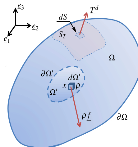
Figura 5.2 – Sistema material \Omega' com condição de contorno \underline{T}^d imposta na fronteira S_T
