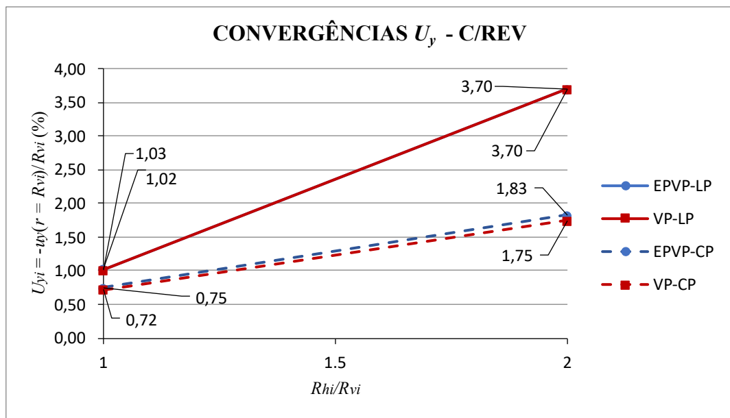
Figura 7.34 – Convergências na direção y versus razão de aspecto da seção com revestimento
