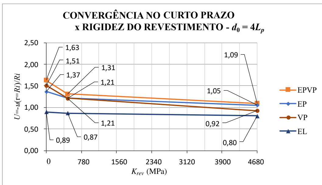
Figura 7.29 – Convergência no final da construção versus módulo de elasticidade do revestimento para uma distância não revestida d_0 = 4L_p
