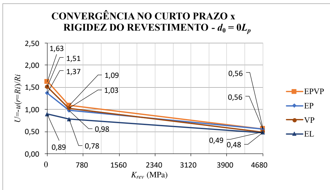
Figura 7.27 – Convergência no final da construção versus módulo de elasticidade do revestimento para uma distância não revestida d_0 = 0
