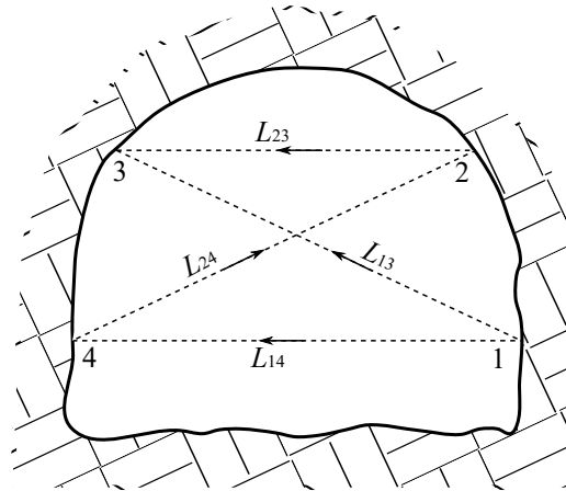
Figura 4.4 – Medidas da convergência em quatro direções de uma seção não circular (adaptado de: Panet (1995, p. 8))
