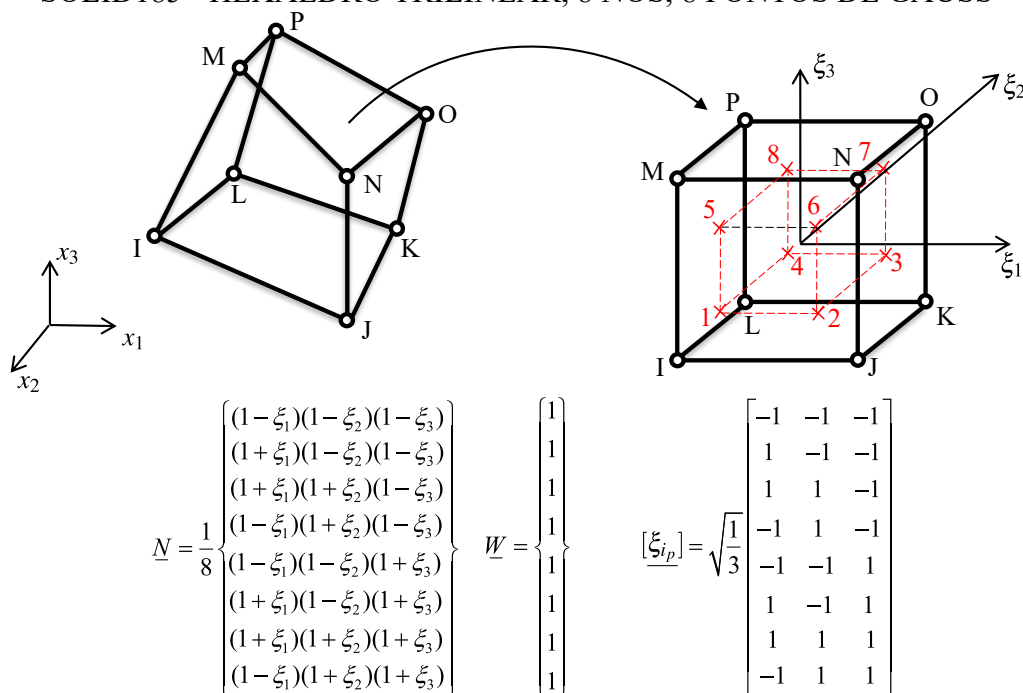
Figura 6.4 – Funções de interpolação, pesos e coordenadas dos pontos de Gauss para o elemento hexaedro trilinear isoparamétrico SOLID185 (adaptado de: ANSYS Inc (2018b, p. 345, 369-370))
