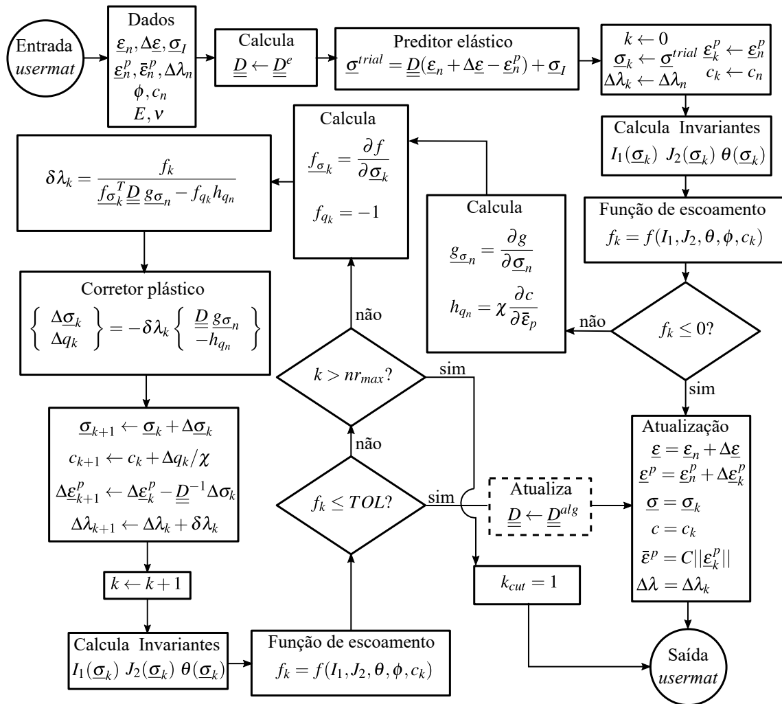
Figura 6.8 – Algoritmo de integração para elastoplasticidade utilizando um esquema de Euler semi-implícito (omitindo o índice n+1 ).
