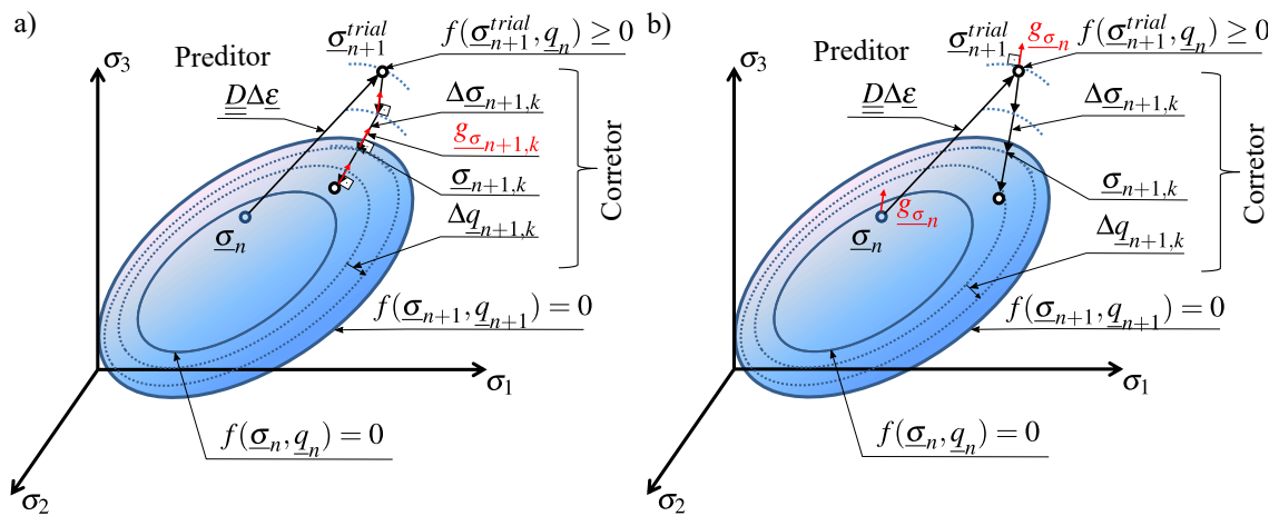
Figura 6.7 – Ilustração do algoritmo de retorno mapeado genérico com k iterações locais de Newton-Raphson: a) totalmente implícito e b) semi-implícito.
