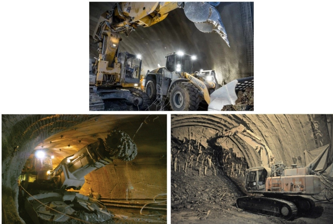
Figura 3.4 – Superior: escavadeiras (fonte: Pierrat (2014, p. 1)); inferior à esquerda: escavadeira rotativa (fonte: Mitterndorfer (2013, p. 1)) e inferior à direita: martelo hidráulico (fonte: WORD HIGHWAYS (2015, p. 1))
