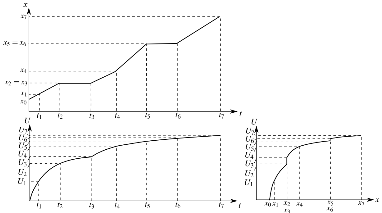
Figura 4.17 – Evolução da convergência U no tempo t em função do avanço da escavação x (adaptado de: Panet (1995, p. 12))
