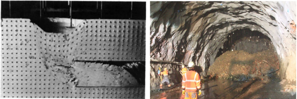
Figura 3.10 – À esquerda, simulação da falha na face de um túnel (fonte: Schofield (1980, p. 245)); à direita, o colapso progressivo da face do túnel rodoviário Vadlaheidi na Islândia (fonte: Reynolds (2015, p. 1))
