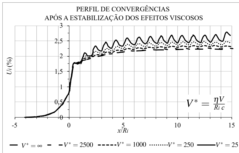
Figura 4.29 – Perfil de convergência em função da velocidade de construção adimensionalizada no final da construção do túnel (adaptado de: Bernaud (1991, p. 214))
