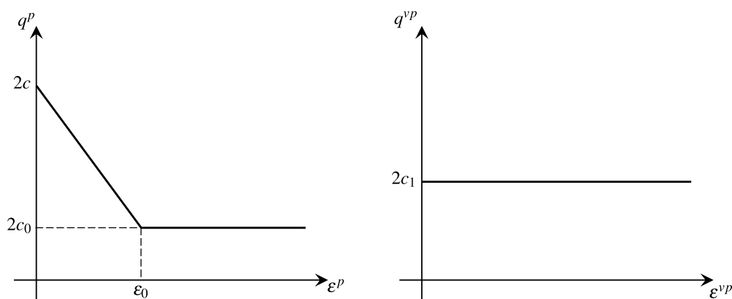
Figura 5.12 – Leis de endurecimento e amolecimento para a parcela elastoplástica (à esquerda) e viscoplástica (à direita) (adaptado de: Rousset (1988, p. 220))
