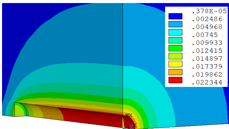
Figura 7.20 – Campo de deslocamentos no longo prazo para o caso elastoplástico-viscoplástico com E = 1500 \text{ MPa} e V_p = 0,1 \text{ m/dia}
