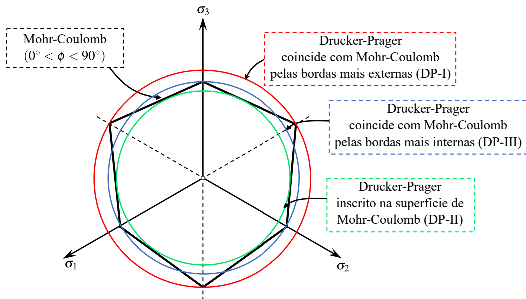
Figura 5.6 – Representação no plano desviador da aproximação da superfície de Mohr-Coulomb pela superfície de Drucker-Prager (adaptado de: de SOUZA NETO; PERI; OWEN, 2008, p. 169 e BERNAUD, 1991, p. 89)
