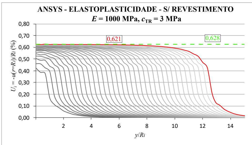
Figura 7.10 – Verificação solução numérica em elastoplasticidade sem revestimento - E = 1000\text{MPa} , c_i = c_p = c_r = 3\sqrt{3}/2\text{MPa}
