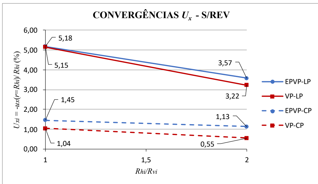
Figura 7.31 – Convergências na direção x versus razão de aspecto da seção sem revestimento
