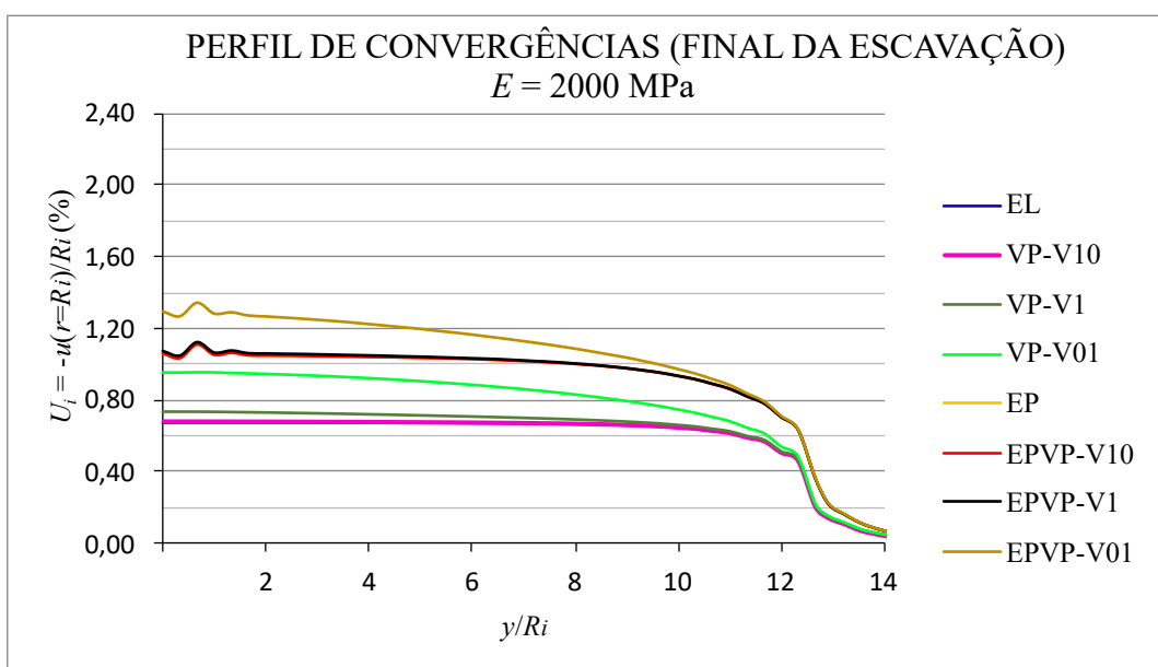
Figura 7.18 – Perfis de convergências no final da escavação para os diversos comportamentos implementados, considerando os parâmetros físicos do maciço de acordo com Piepi (1995) com E = 2000 \text{ MPa}
