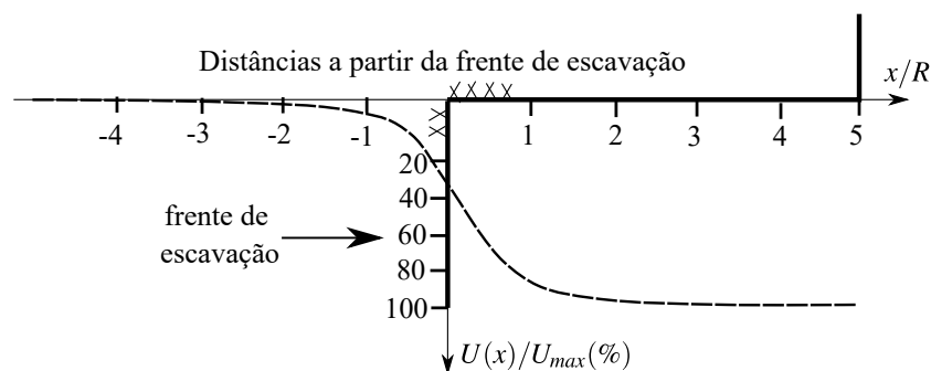
Figura 4.5 – Perfil de convergências próximo à frente de escavação (adaptado de: Hanafy e Emery (1980) apud Couto (2011, p. 42))
