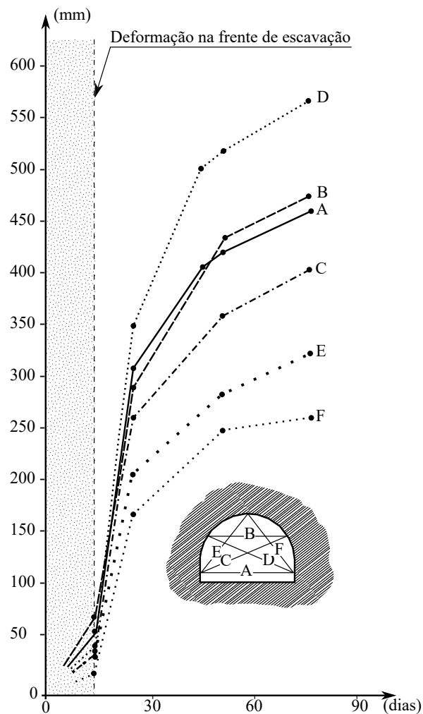
Figura 4.10 – Evolução da convergência do túnel Fréjus (adaptado de: Lunardi (1980, p. 17))
