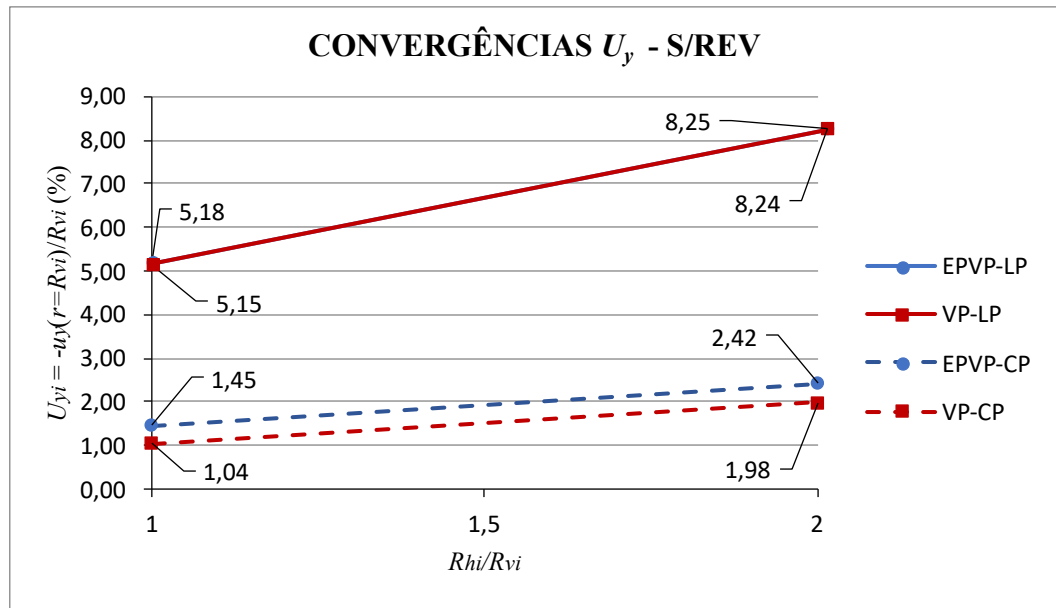
Figura 7.33 – Convergências na direção y versus razão de aspecto da seção sem revestimento
