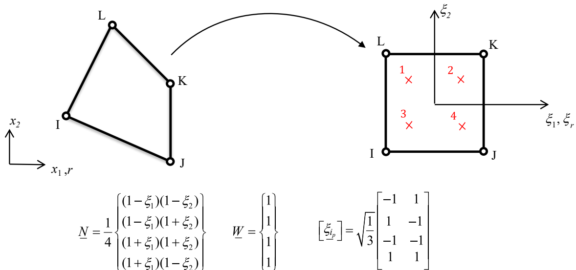
Figura 6.3 – Funções de interpolação, pesos e coordenadas dos pontos de Gauss para o elemento quadrilátero linear isoparamétrico PLANE182 (adaptado de: ANSYS Inc (2018b, p. 334, 369-370))
