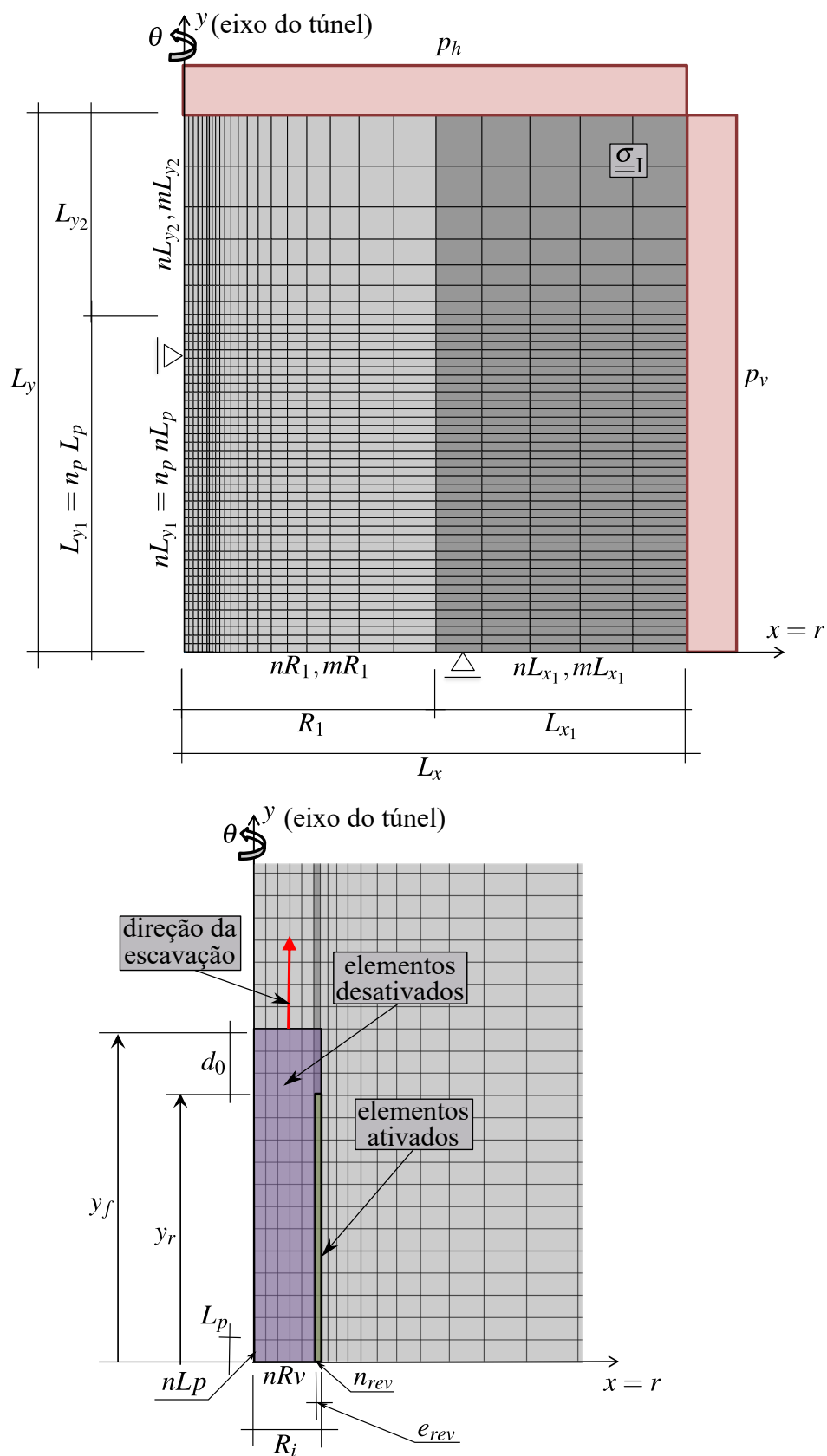
Figura 6.14 – Domínio, parâmetros geométricos, condições de contorno e malha para o modelo axissimétrico
