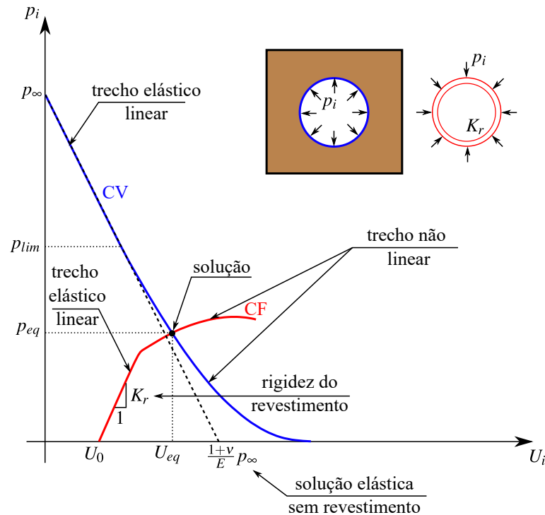
Figura 4.30 – Método da Convergência-Confinamento (adaptado de: Bernaud, Benamar e Rousset (1994, p. 6))
