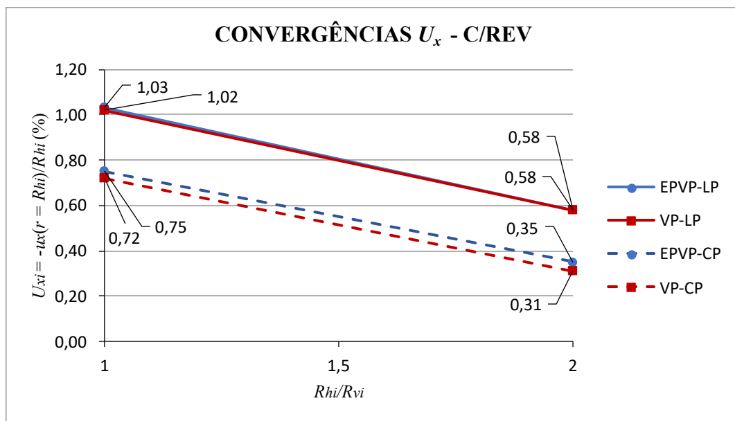
Figura 7.32 – Convergências na direção x versus razão de aspecto da seção com revestimento
