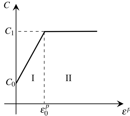
Figura 7.3 – Variação da coesão: I - trecho de endurecimento linear e II - comportamento perfeitamente plástico (Bernaud e Quevedo (2020, p. 4))
