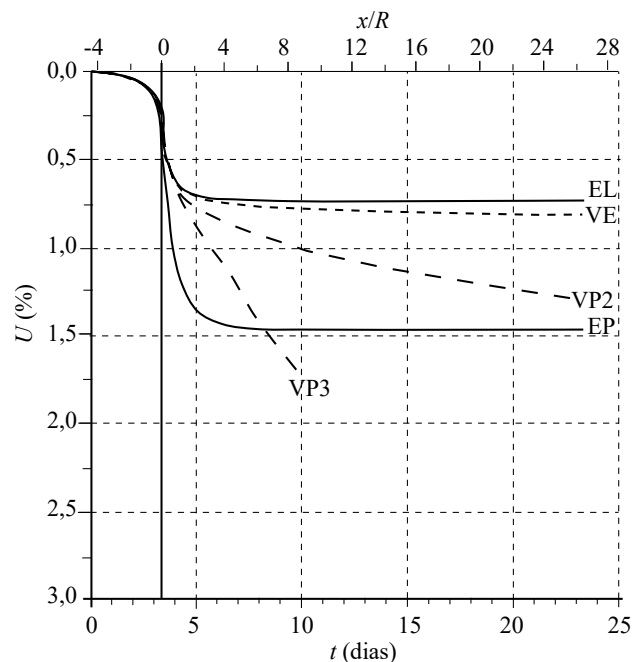
Figura 4.18 – Perfil de convergências, em análises numéricas axissimétricas com maciço elástico (EL), elastoplástico (EP), viscoelástico (VE), viscoplástico com fluência no regime secundário (VP) e em regime terciário (VP3), todos na ausência de revestimento (adaptado de: Sterpi e Gioda (2009, p. 329))
