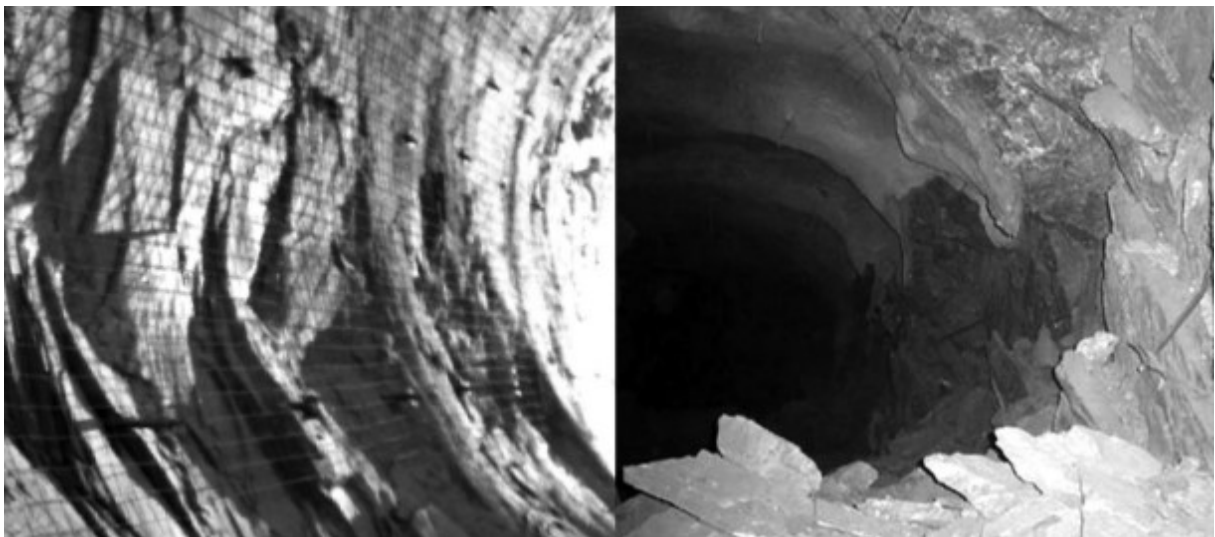
Figura 4.9 – À esquerda uma seção remanescente após moderada fragmentação e quebra em um túnel escavado com TBM e à direita uma seção em que parte do contorno apresentou instabilidade (flambagem) em um túnel escavado de forma não mecanizada (fonte: Diederichs (2007, p. 1084))
