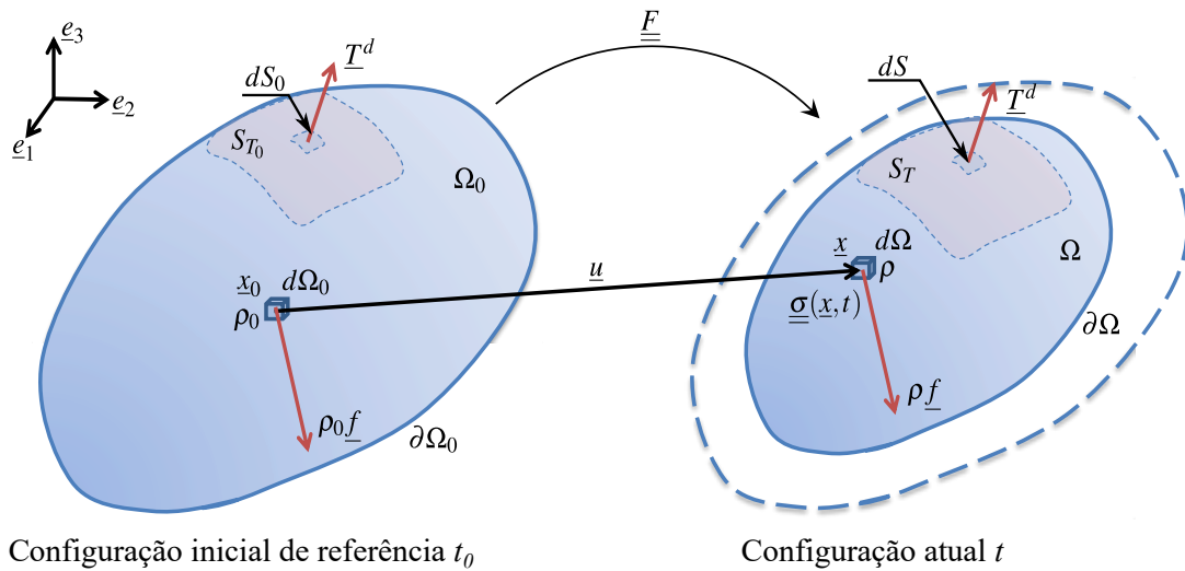
Figura 5.3 – Natureza Euleriana do campo de tensões
