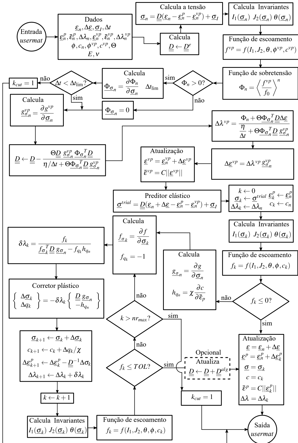
Figura 6.10 – Algoritmo de integração do modelo constitutivo elastoplástico-viscoplástico (omitindo o índice n+1 ).
