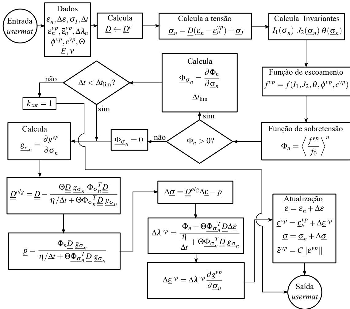
Figura 6.9 – Algoritmo de integração para viscoplasticidade utilizando um esquema de Euler semi-implícito ou totalmente explícito (quando \Theta = 0 ) sem endurecimento/amolecimento (omitindo o índice n + 1 ).
