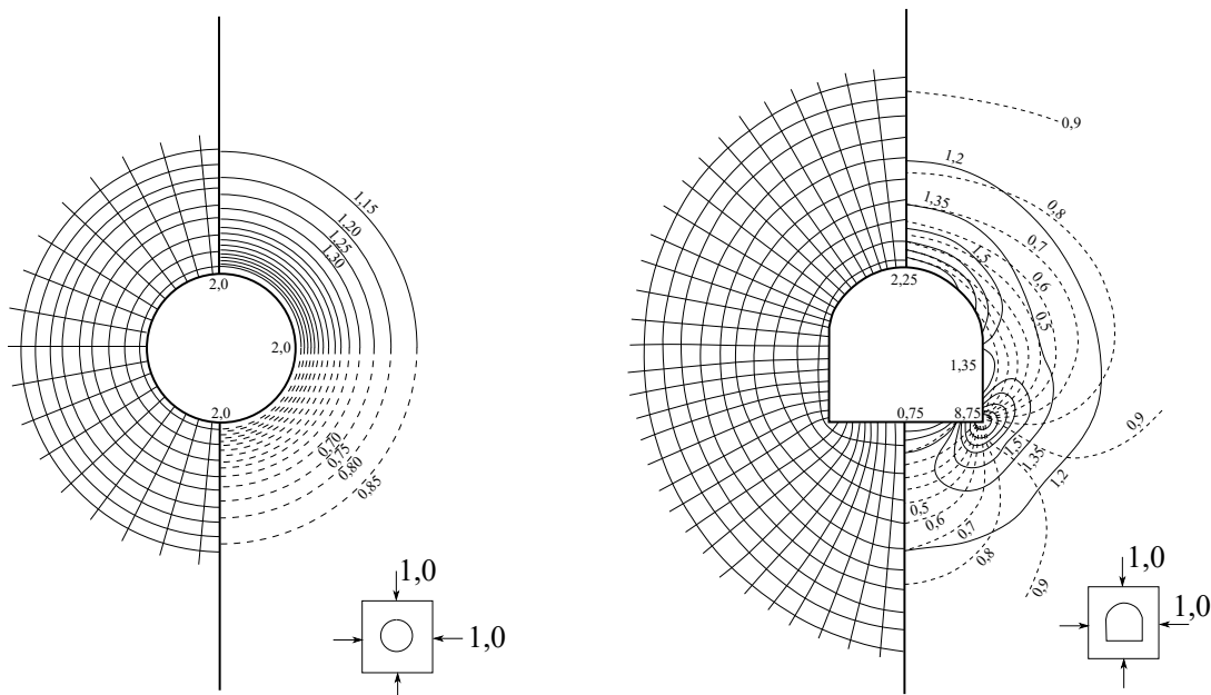
Figura 4.19 – Trajetória das tensões principais e linhas de isotensão, da maior e menor tensão principal, para seção circular (à esquerda) e ferradura (à direita) em condições geostáticas hidroestáticas (adaptado de: Hoek e Brown (1980, p. 469, 484))
