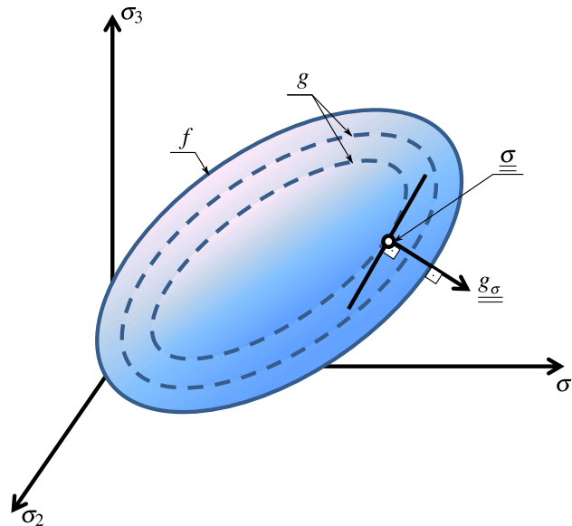
Figura 5.8 – Representação geométrica do vetor de fluxo em plasticidade associada (adaptado de: Chen e Han (1988, p. 182))
