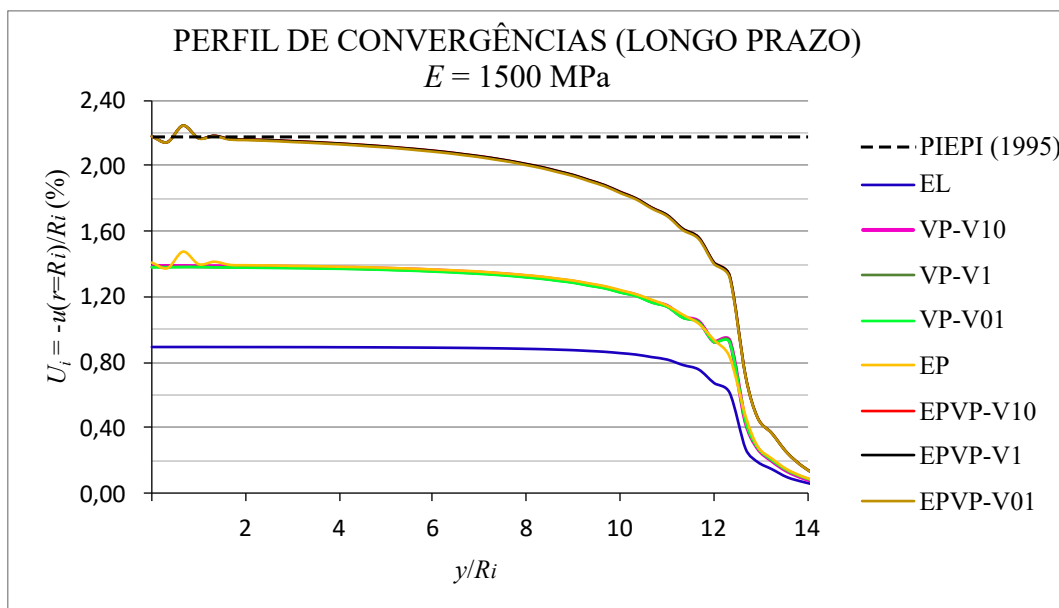
Figura 7.17 – Perfis de convergências no longo prazo para os diversos comportamentos implementados, considerando os parâmetros físicos do maciço de acordo com Piepi (1995) com E = 1500 \text{ MPa}
