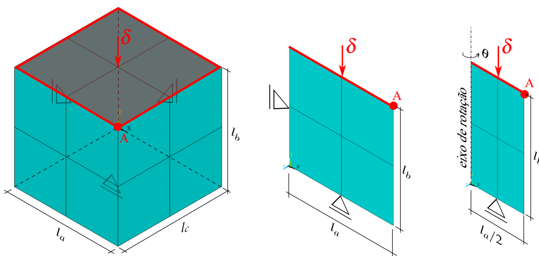
Figura 7.1 – Domínio e discretização de um ensaio triaxial com modelo 3D, EPD e AXI
