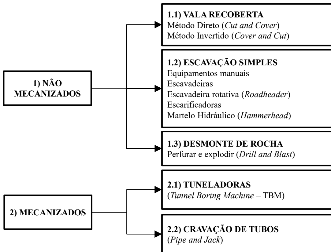
Figura 3.1 – Métodos de escavação de túneis (elaborado pelo autor, com informações de: FEDERAL HIGHWAY ADMINISTRATION (U.S.) (2009), Chapman, Metje e Stärk (2018) e Brox (2017))
