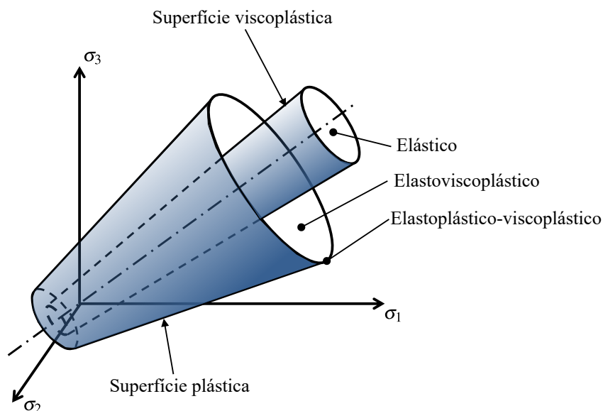
Figura 5.13 – Domínios e superfícies do modelo elastoplástico-viscoplástico (adaptado de: Debernardi e Barla (2009, p. 263))
