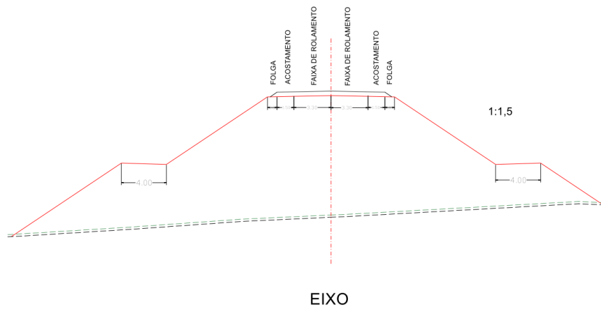
Figura 18: Seção de aterro com banquetas
