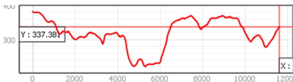
Figura 5: declividade diretriz
