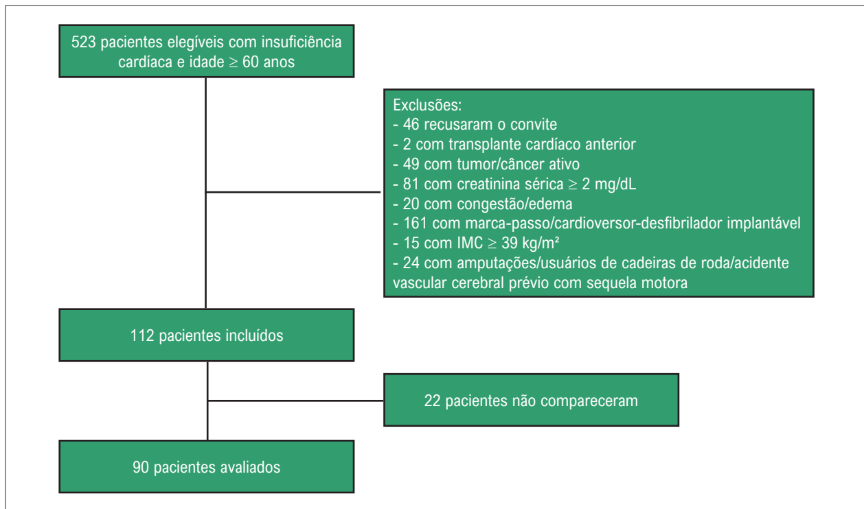
Figura 1 – Fluxograma de recrutamento de pacientes. IMC: índice de massa corporal.
