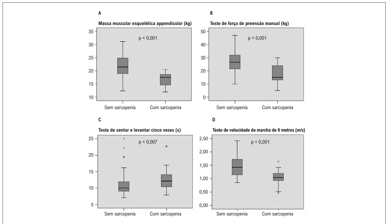
Figura 2 – Gráfico de caixa de critérios diagnósticos para sarcopenia. (A) Massa muscular esquelética apendicular em pacientes sem e com sarcopenia (21,44 kg (18,82 - 24,89) vs. 17,47 kg (14,29 - 18,66) (B) Força de prensão manual em pacientes sem e com sarcopenia (26,50 kg (21,25 - 32) vs. 15 kg (12,75 - 24), (C) Teste de sentar e levantar cinco vezes em pacientes sem e com sarcopenia (10 s (9,03 - 11,93) vs. 12,12 s (10,38 - 14,33), (D) teste de velocidade de marcha de 6 metros em pacientes sem e com sarcopenia (1,42 s (1,14 - 1,72) vs. 1,04 s (0,91 - 1,21).
