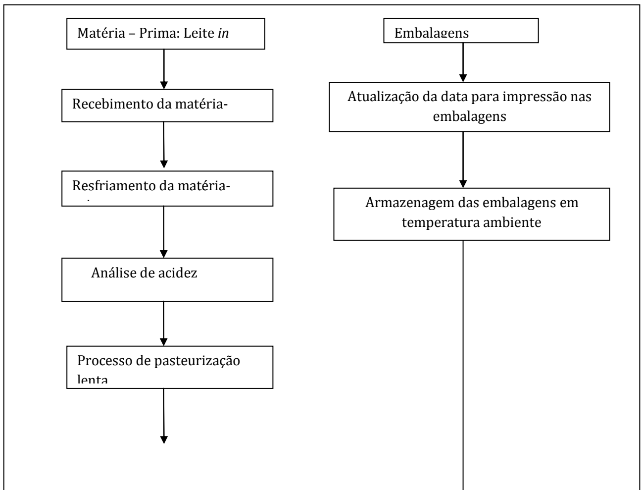
Figura 3 - Fluxograma do cronograma de pasteurização lenta e etapas da produção da Agroindústria Fazenda Ouro Branco
