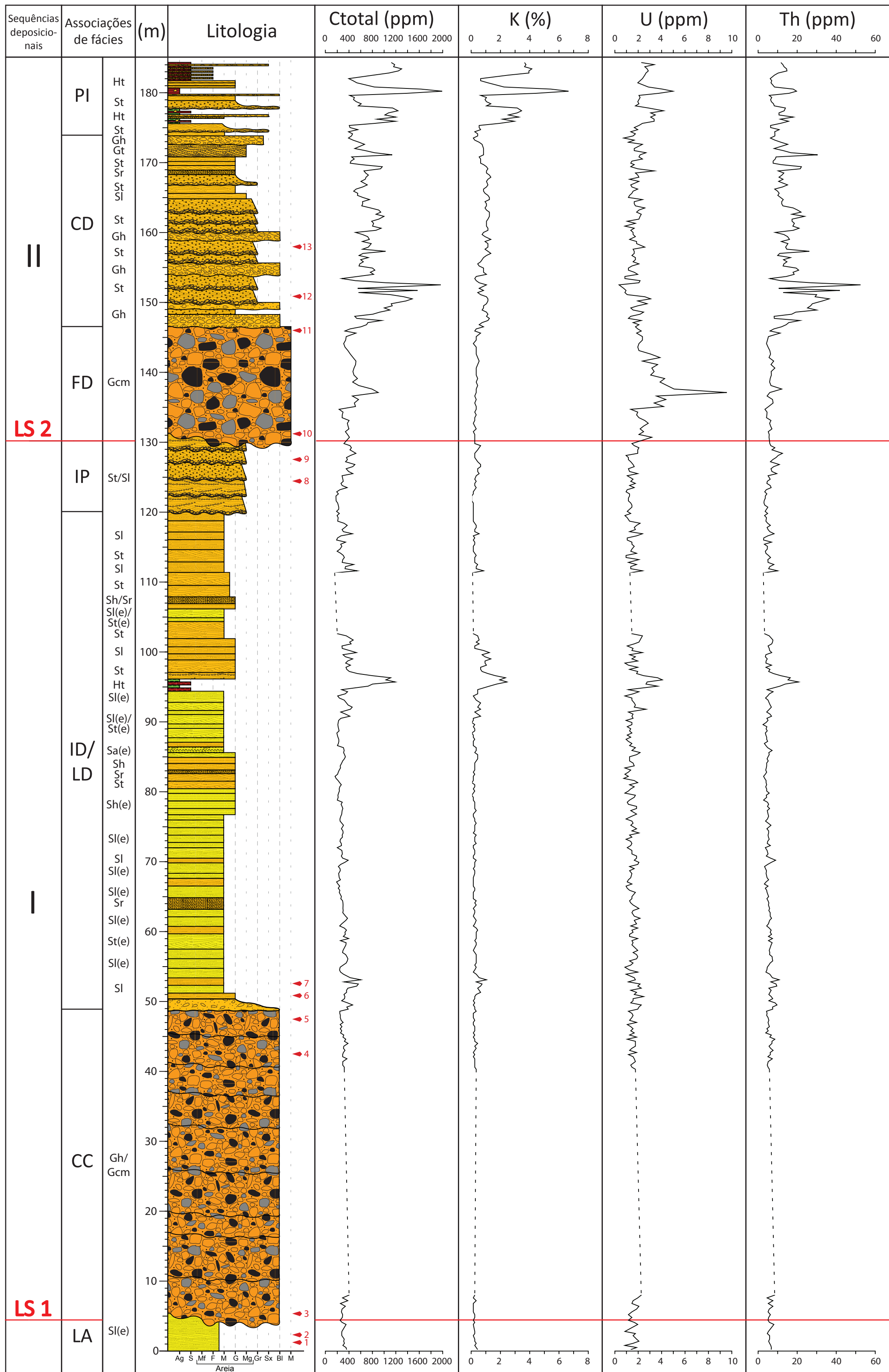
Anexo 1. Perfil colunar com correlação entre os dados da análise de fácies e do levantamento gamaespectrométrico, com interpretação das associações de fácies, limites de sequências (LS1 e LS2) e sequências deposicionais (I e II). (◄) localização de coleta das amostras petrográficas.
