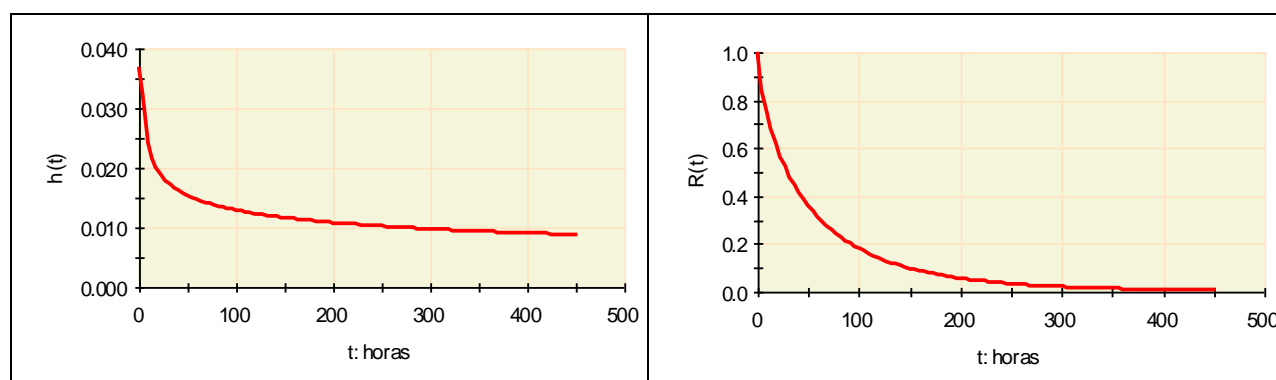
Figura 5.1 – Representação da taxa de falhas (E) e confiabilidade (D) do equipamento.
