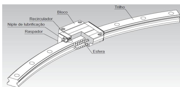
Figura 3.2 – Guia linear da guia R modelo HCR da THK.
