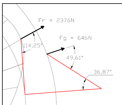
5.5 – Força resultante na guia circular.
