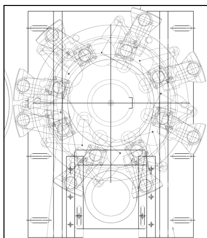
Figura 4.1 – Visualização geral do conjunto desacelerador de produtos.
