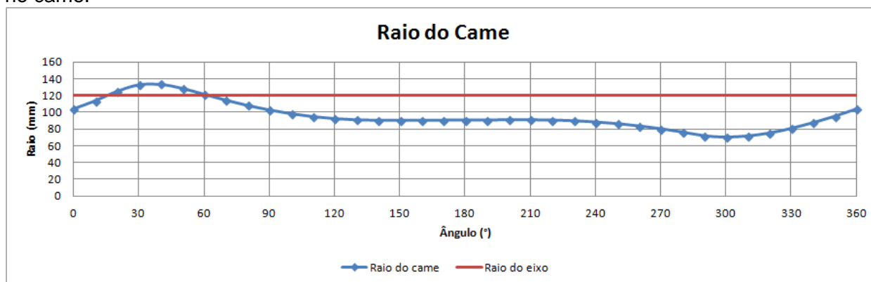
5.2 – Medidas obtidas para o raio do came.
