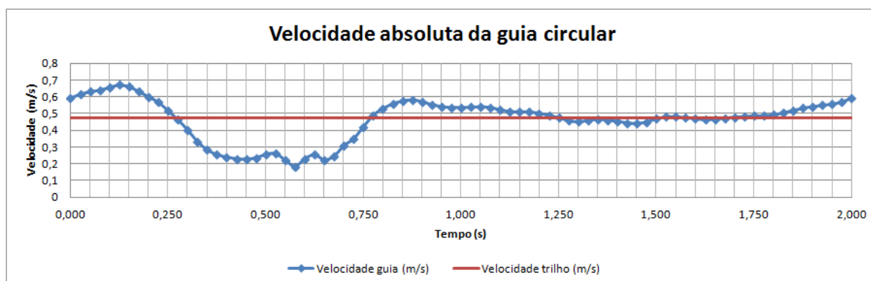
Figura 5.3 – Perfil de velocidade do trilho e da guia circular para 30rpm.
