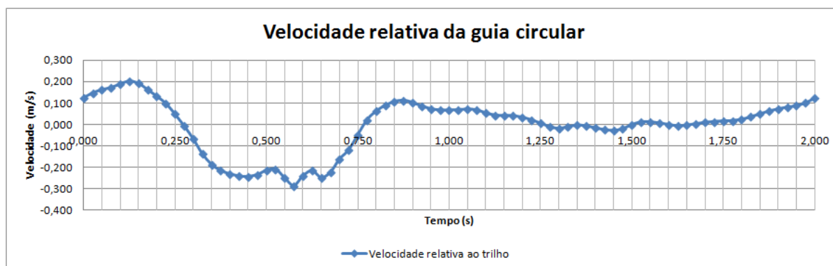
Figura 5.4 – Perfil de velocidade da guia circular relativa ao trilho para 30 rpm.
