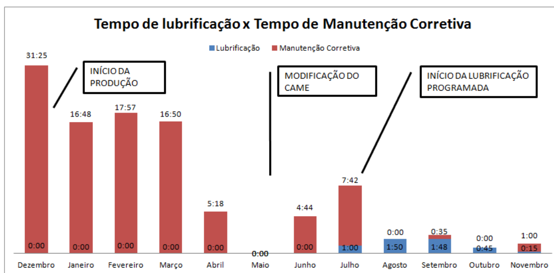
6.1 - Redução da manutenção corretiva após início da lubrificação programada.
