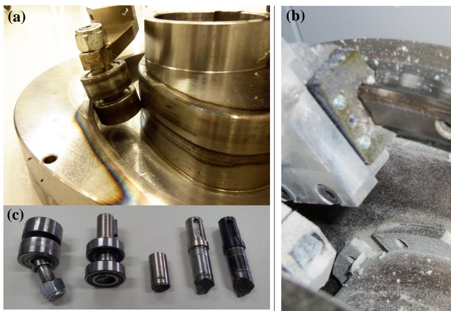
Figura 4.2 – Imagens de algumas falhas no equipamento, em (a) travamento dos rolamentos no came após quebra da guia circular, em (b) oxidação dos trilhos devido à lubrificação insuficiente e em (c) ruptura dos eixos.
