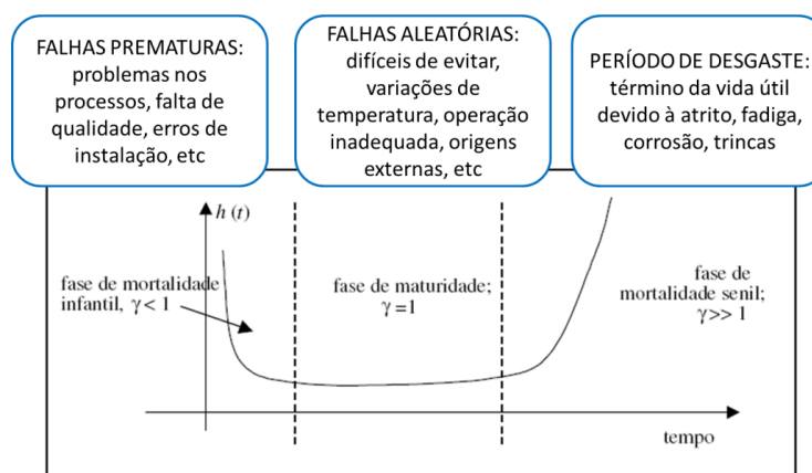
Figura 3.1 – Curva da banheira e ciclo de vida de equipamentos. Adaptado de SELLITO 2005.
