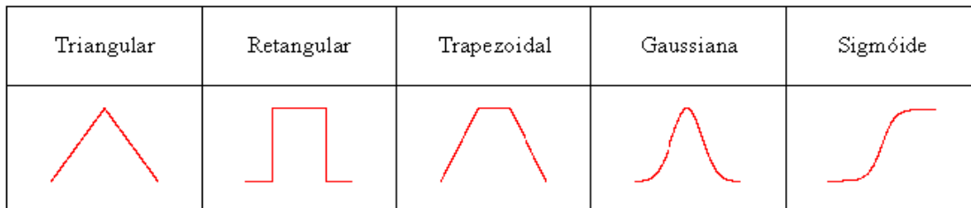
Figura 4.1: Funções de pertinência fuzzy (NASCIMENTO, 2000).
