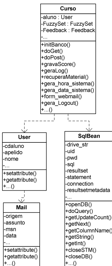
Figura 6.2: Diagrama de Classes
