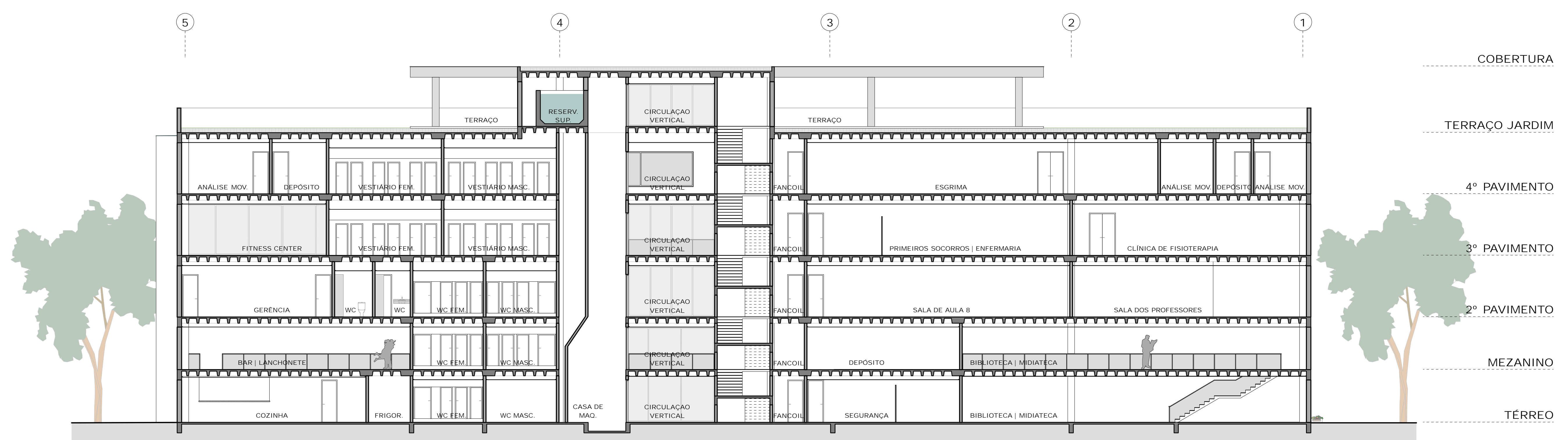
CORTE BB ESCALA 1:125
