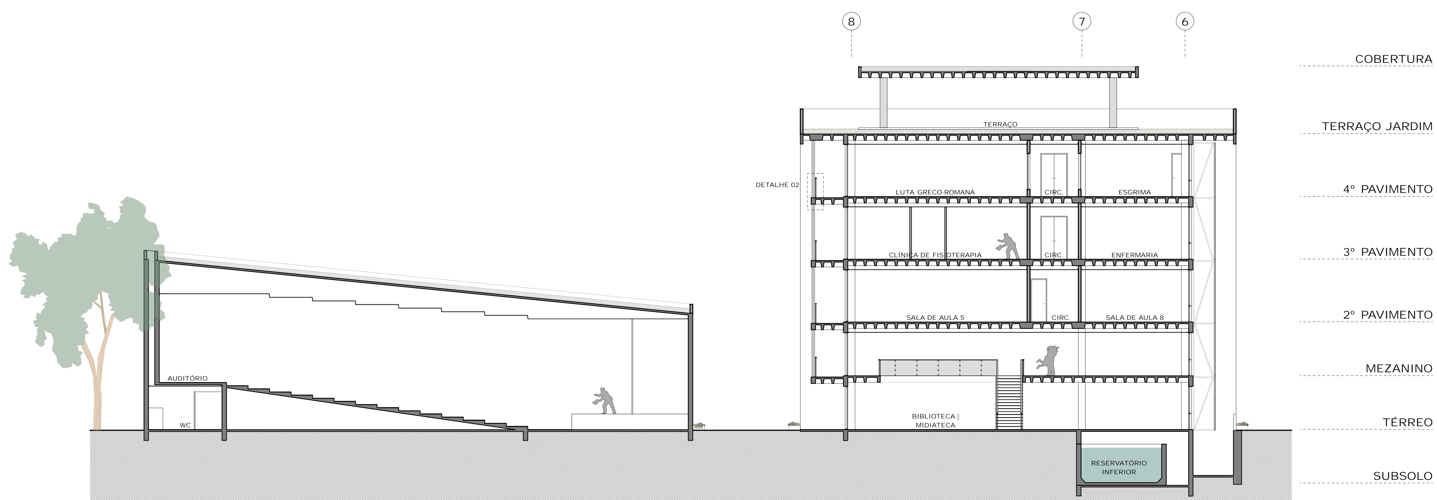
CORTE DD ESCALA 1:125
