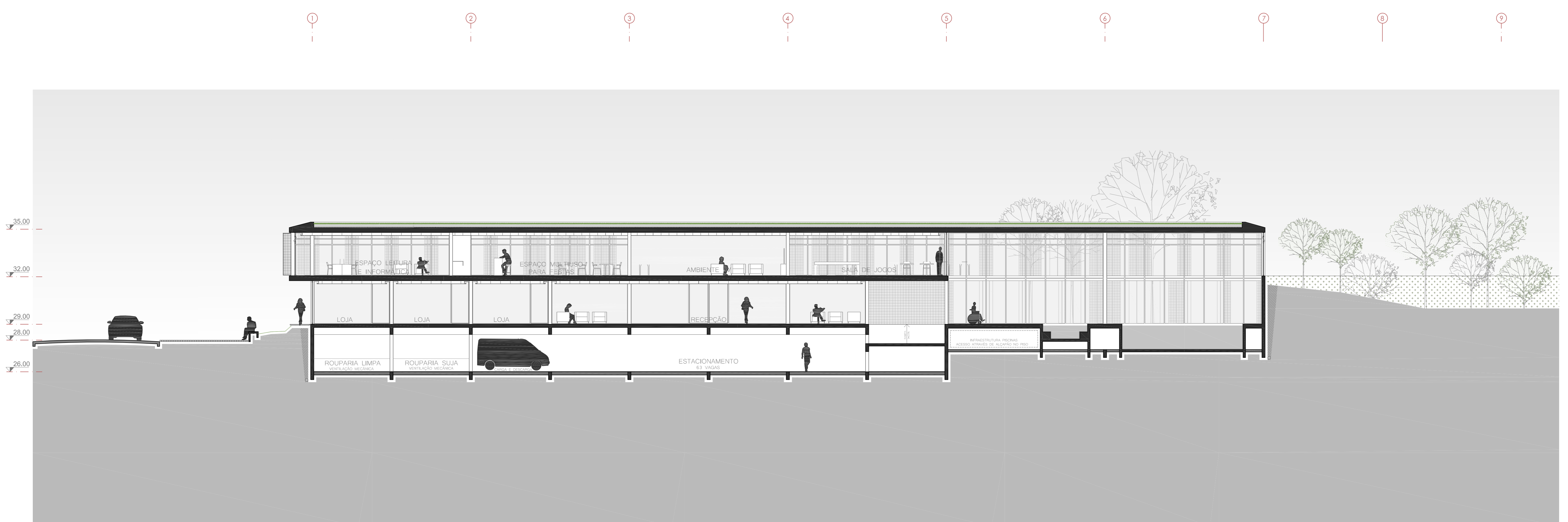
CORTE A ESCALA 1:125
