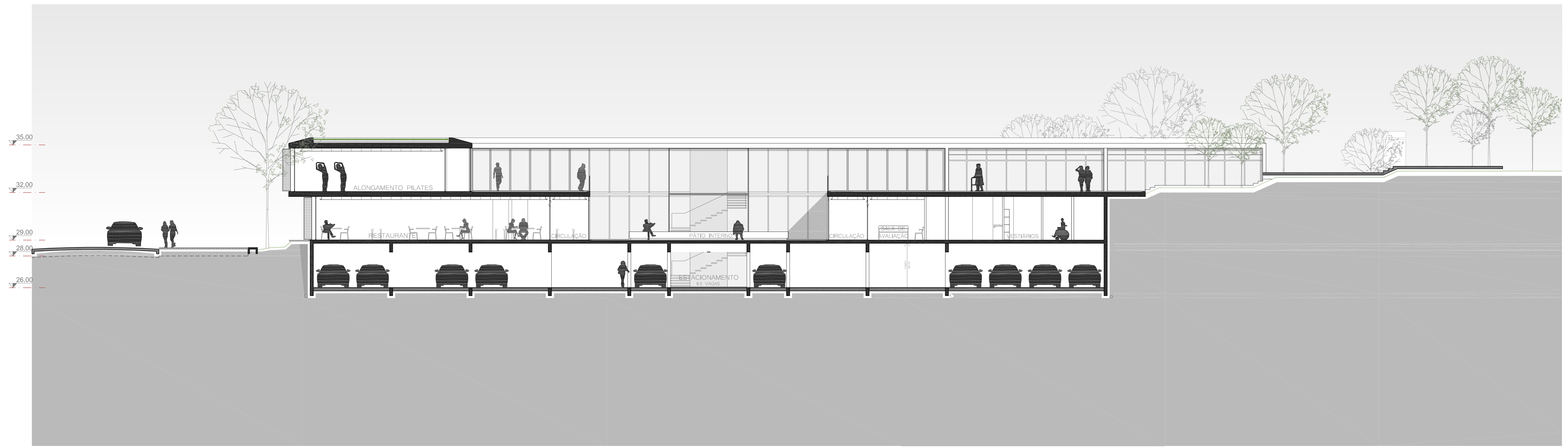
CORTE B ESCALA 1:125
