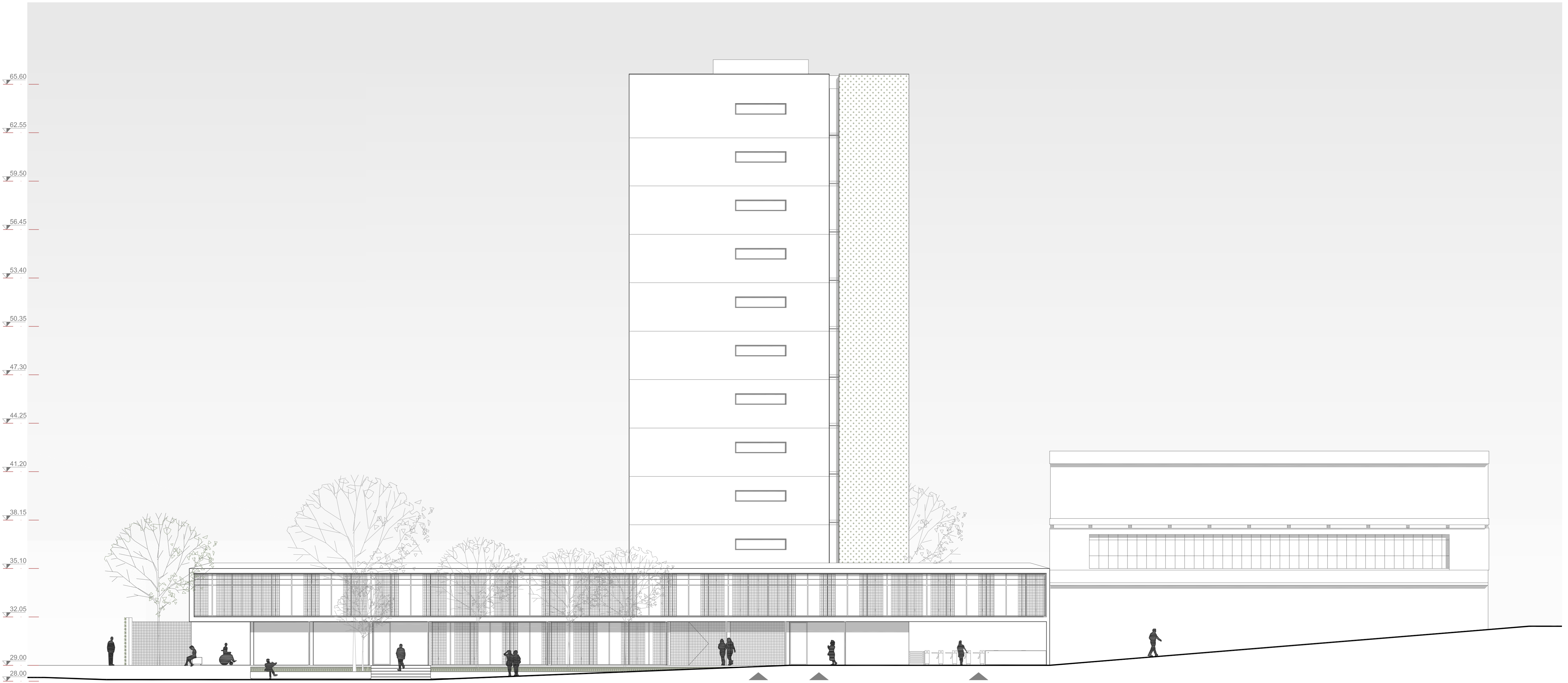
FACHADA LESTE ESCALA 1:125
