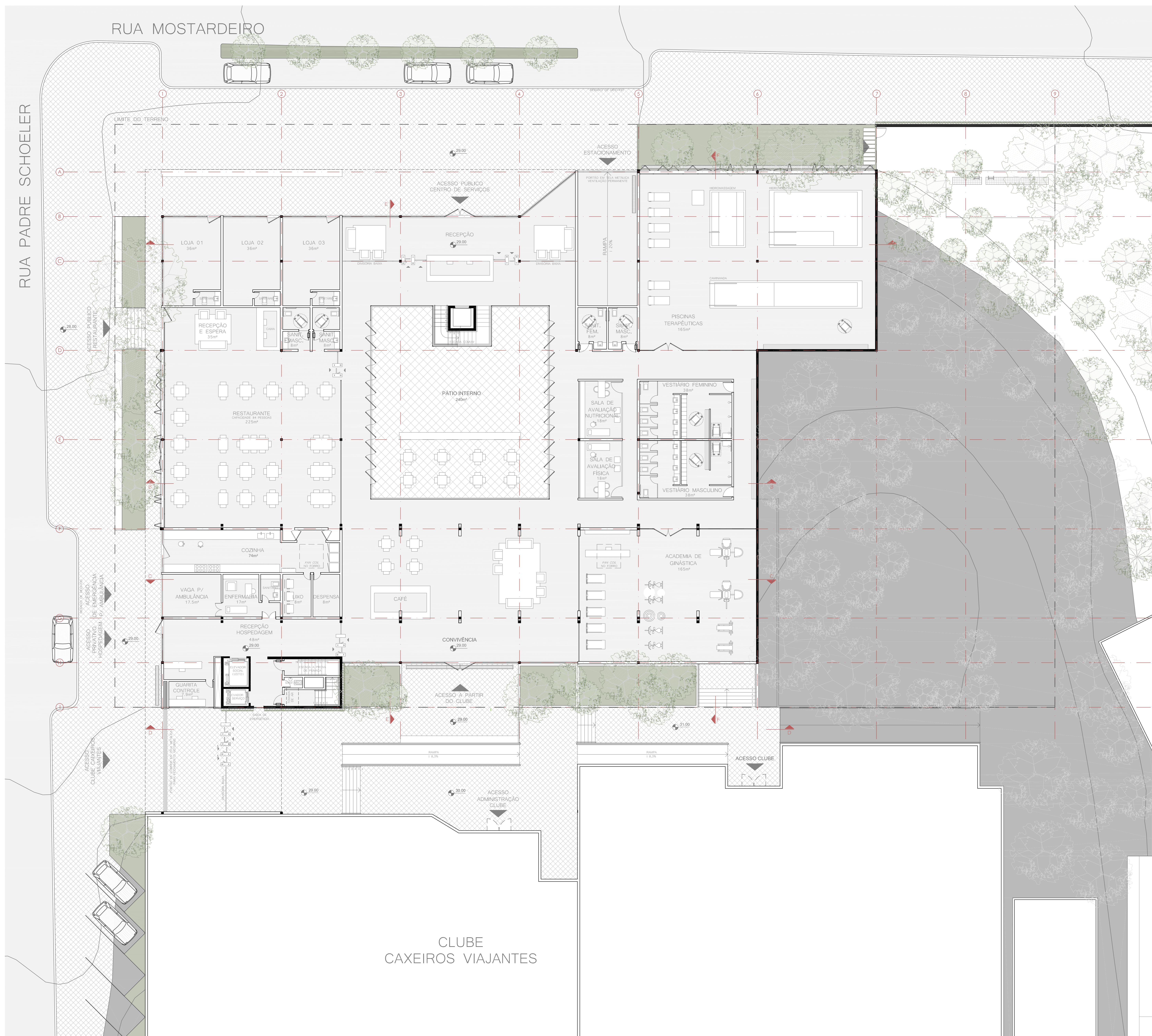
⊙ PAVIMENTO TÉRREO Nv 29.0 ESCALA 1:125
