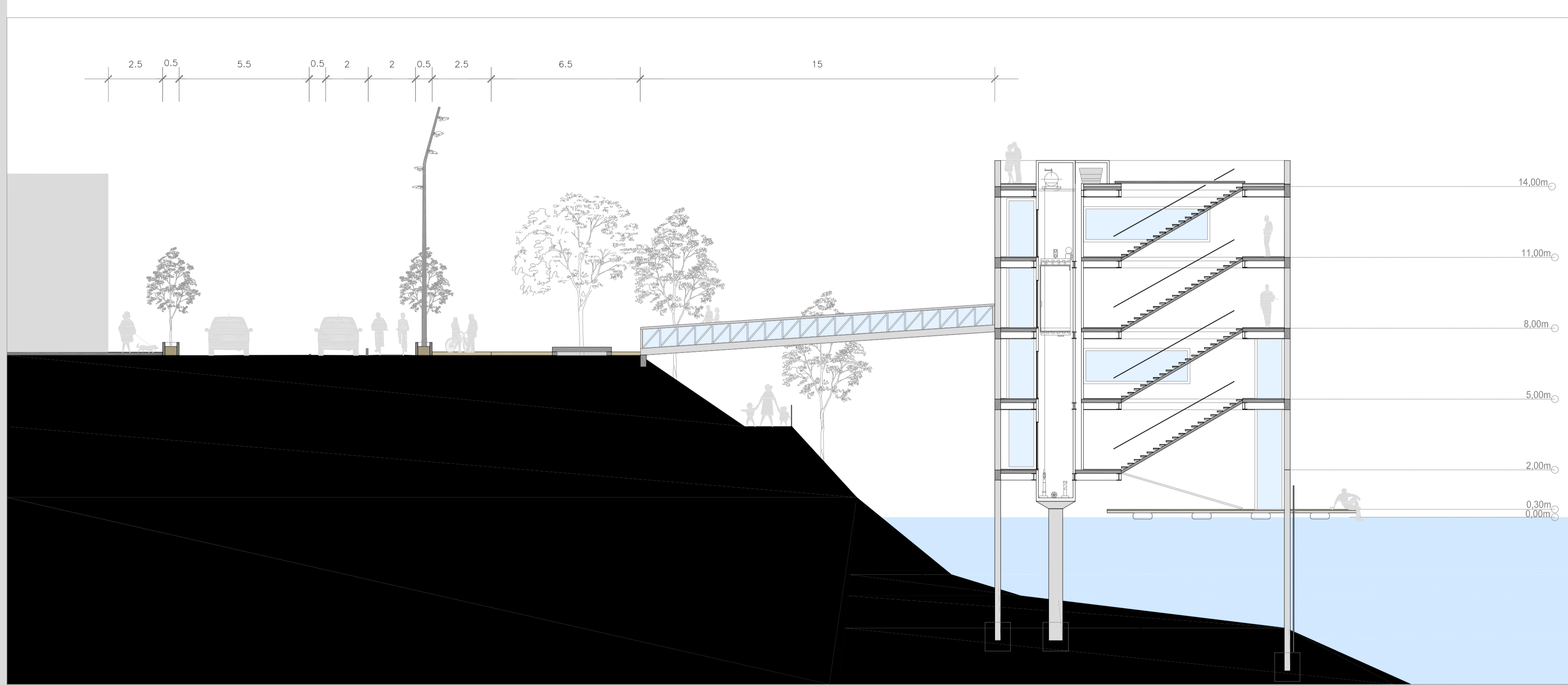
CORTE AA' | Escala 1:125
