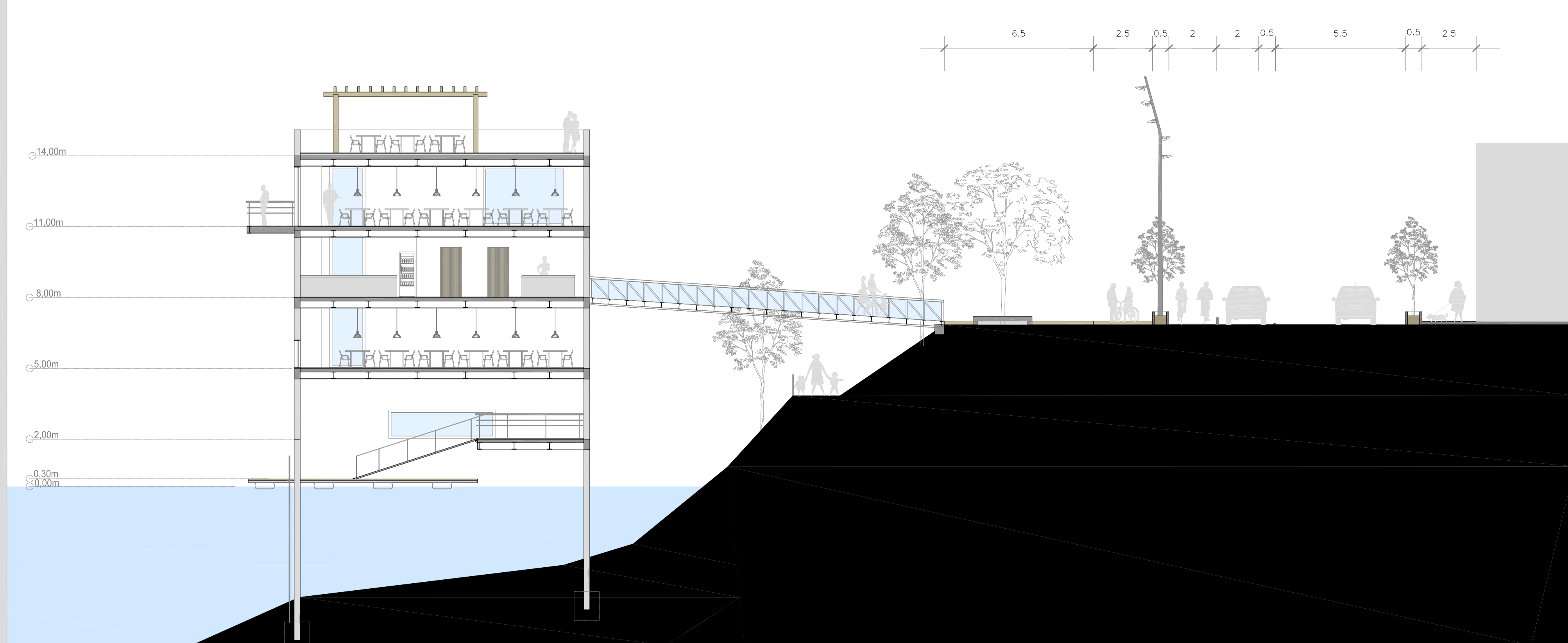
CORTE BB' | Escala 1:125
