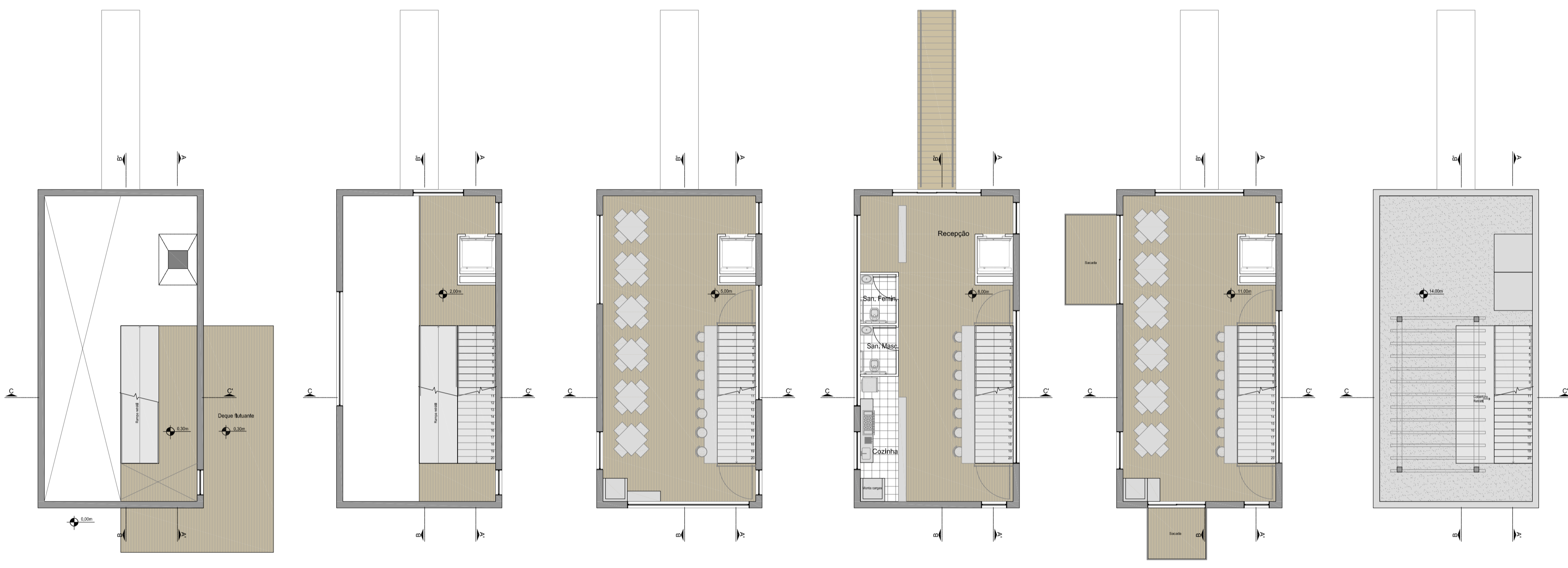
PAVILHÃO RESTAURANTE | Escala 1:125
