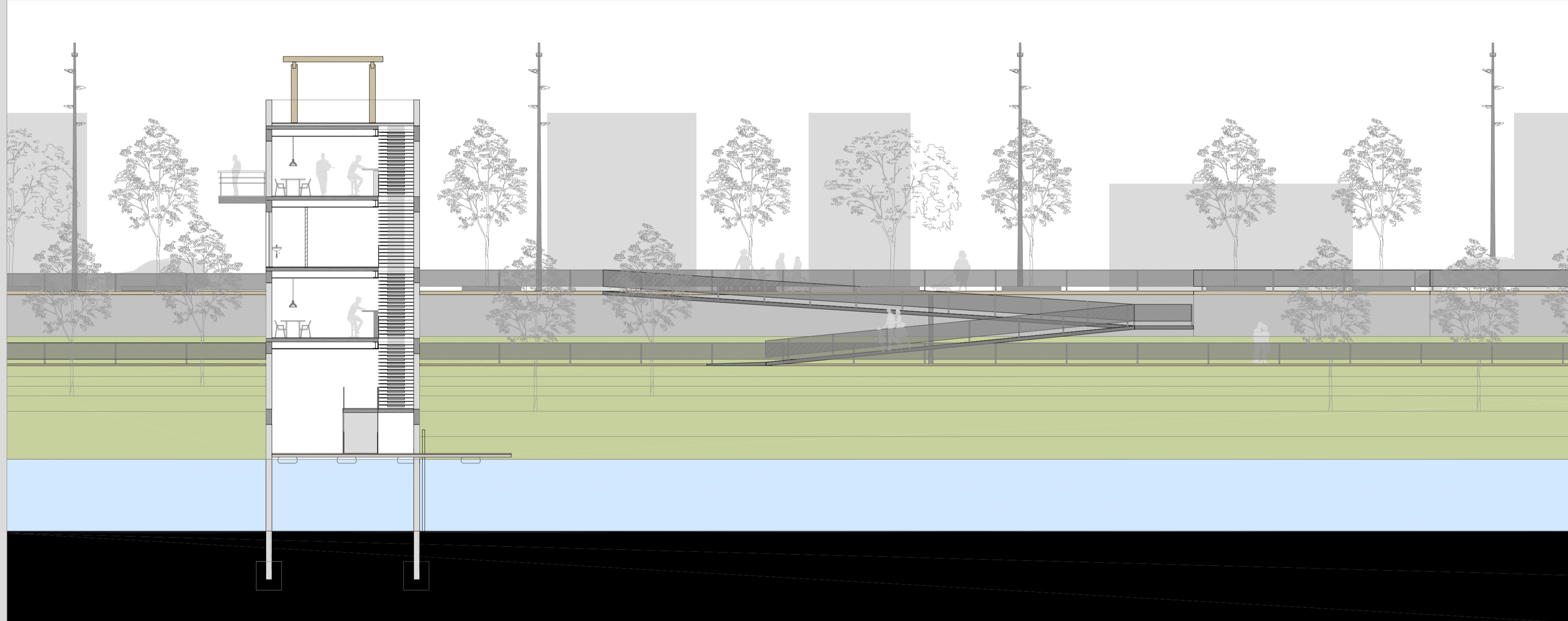
CORTE CC' | Escala 1:125
