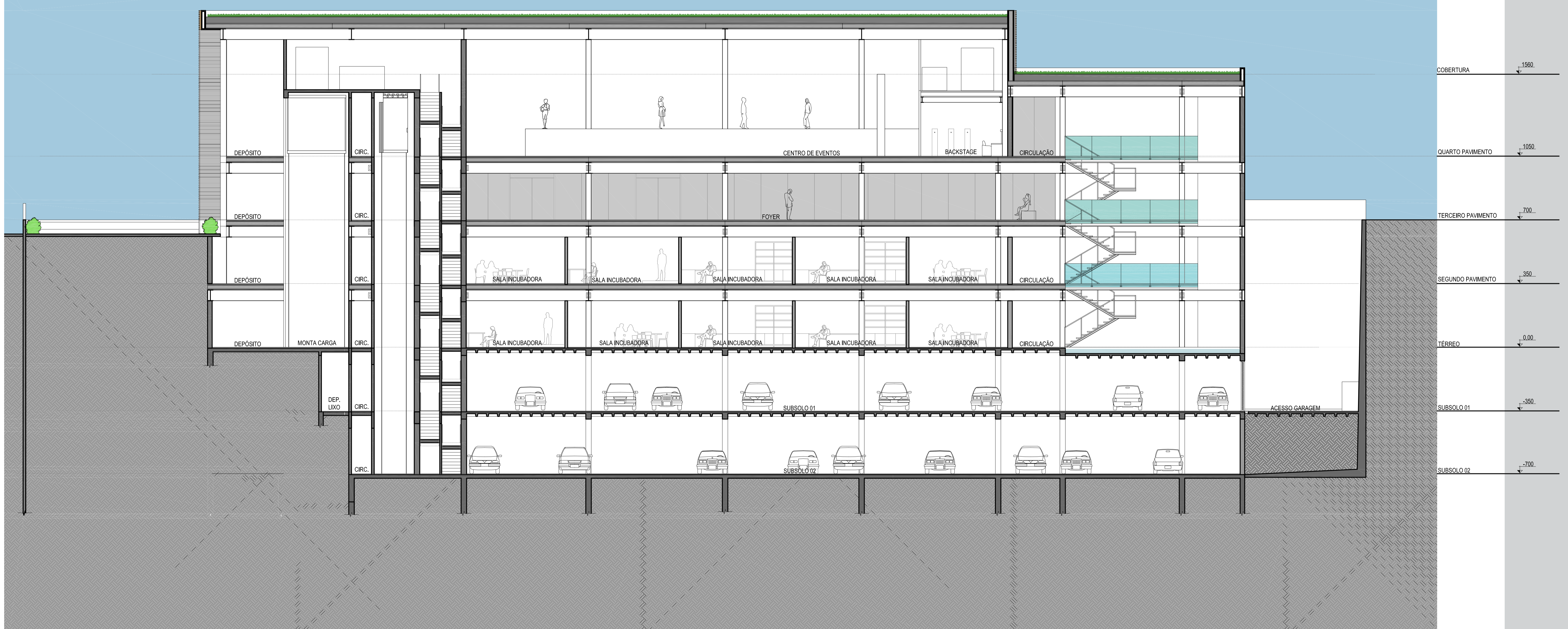
CORTE DD'
