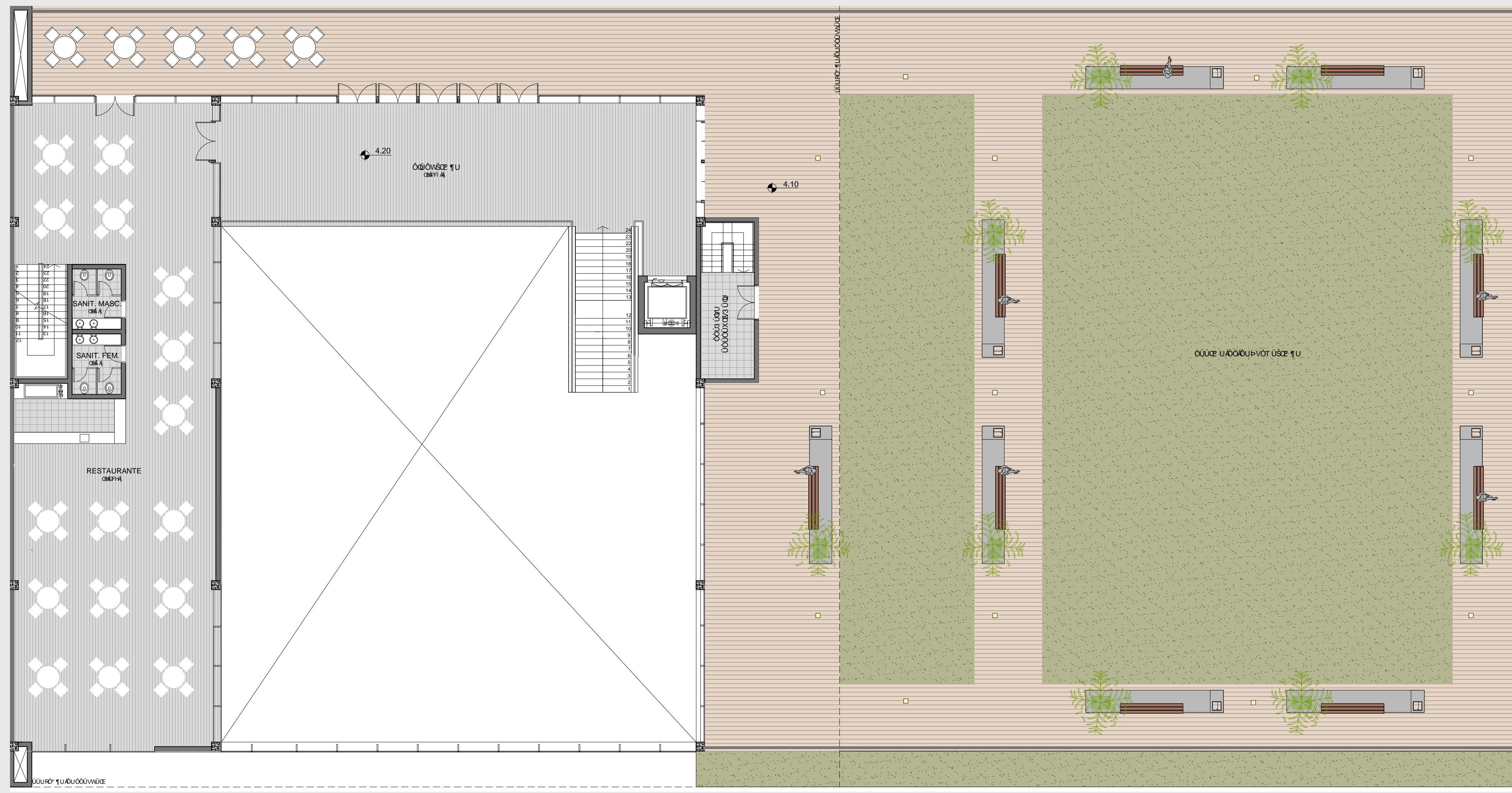
PLANTA BAIXA SEGUNDO PAVIMENTO e 1/125
