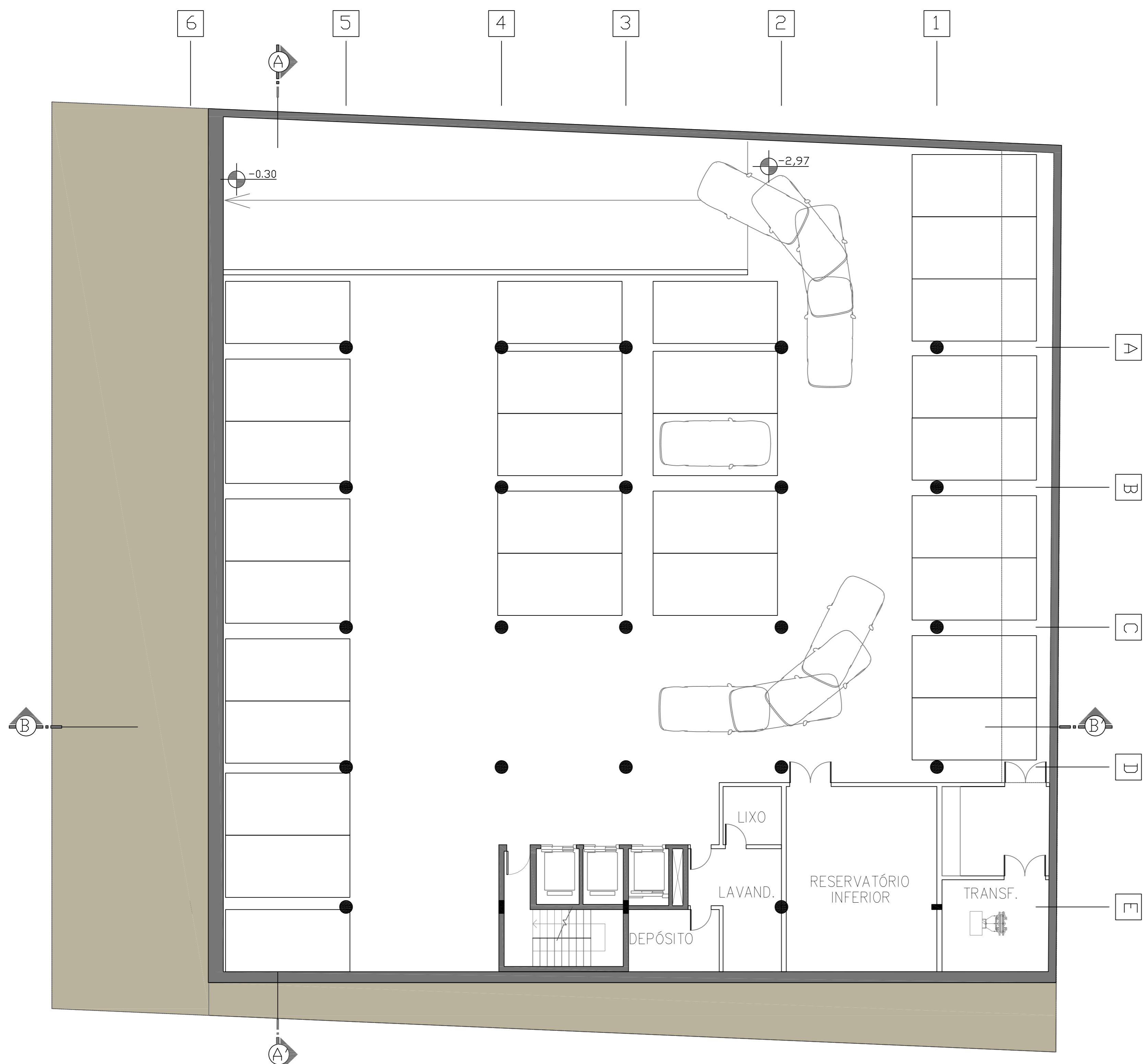
PLANTA BAIXA _ SUBSOLO cota -2,97
