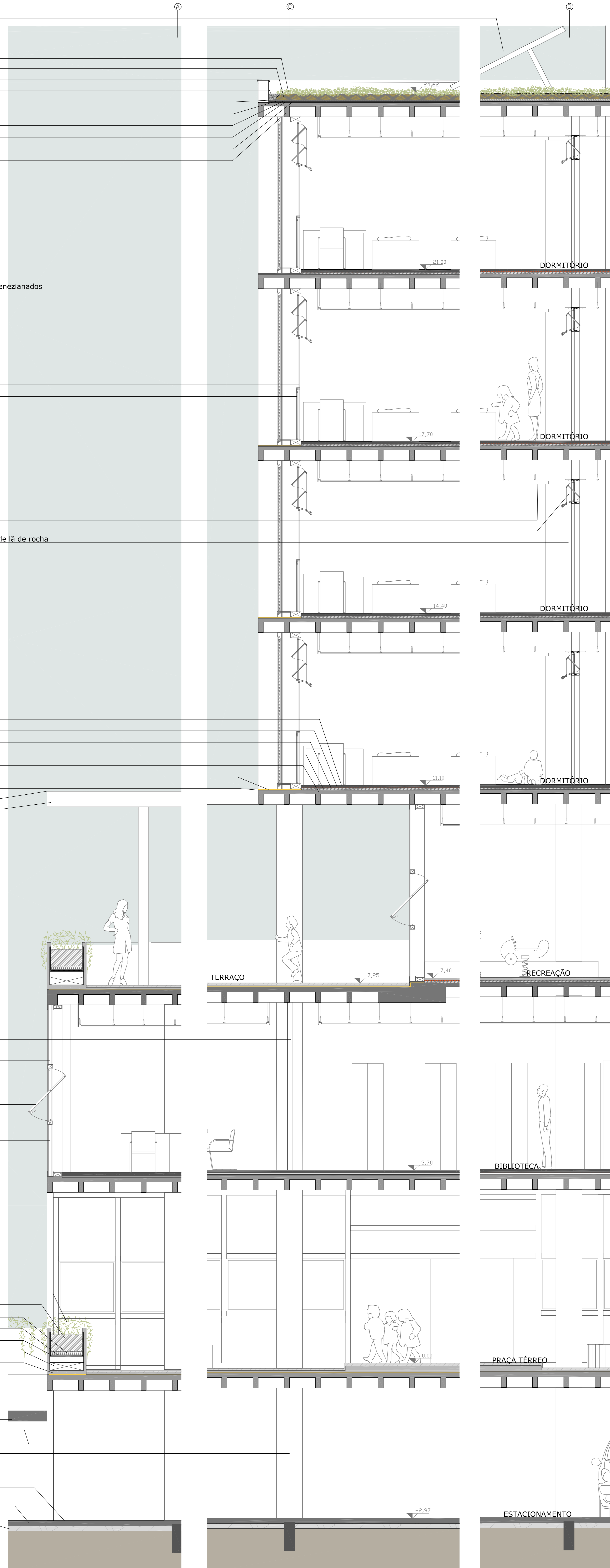
CORTE DE PELE 1/25
