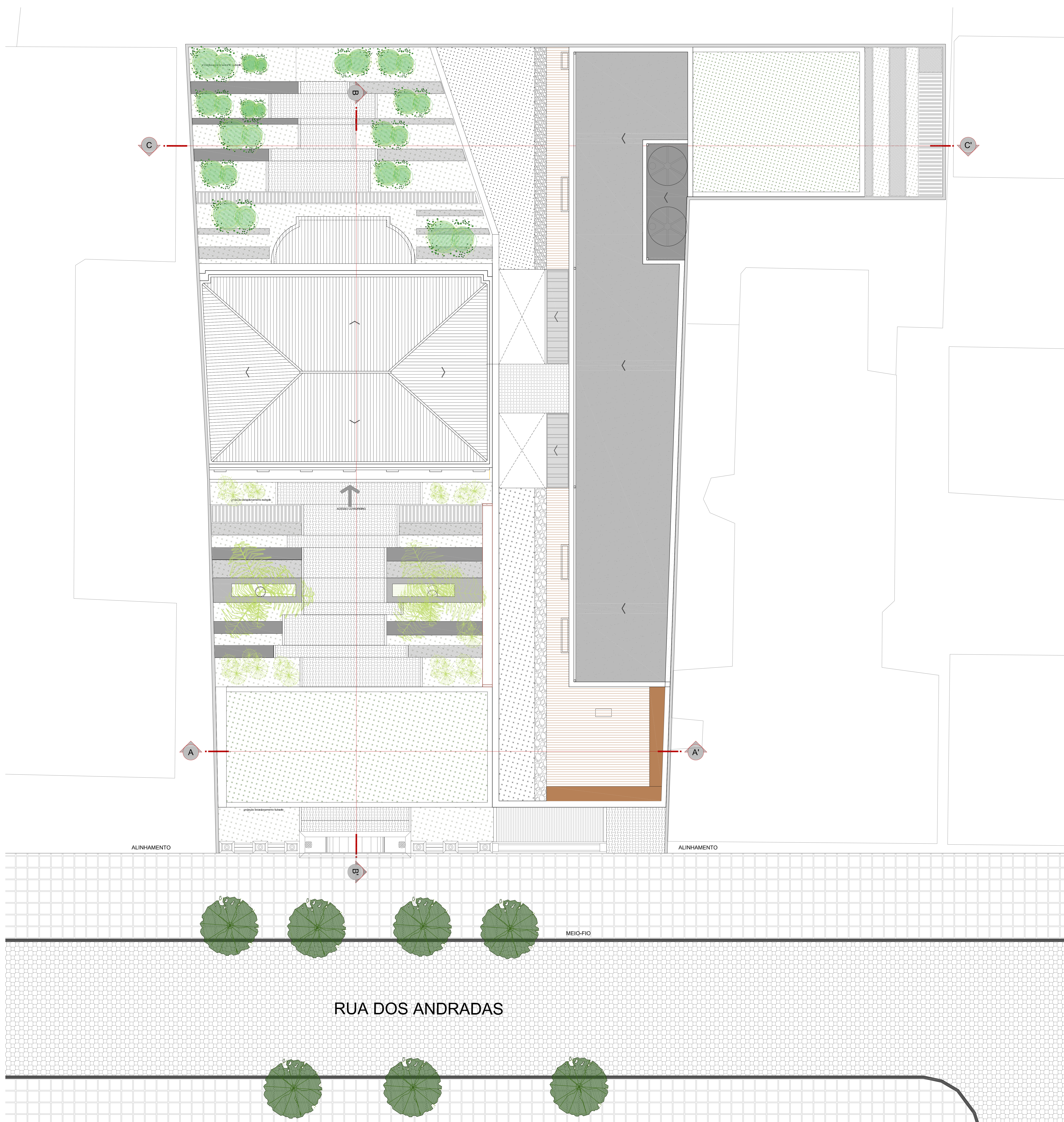
PLANTA BAIXA COBERTURA_esc 1/75
