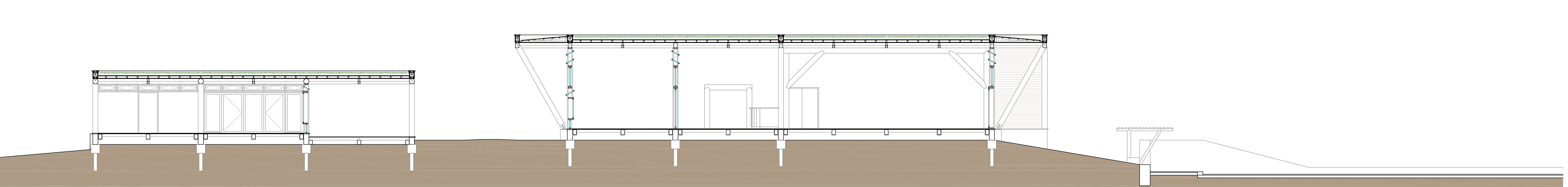
1:100 Secção B-B'
