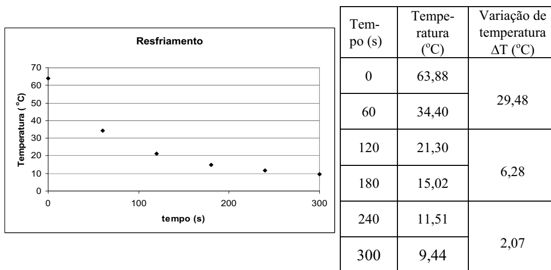
Fig. 3- Dados coletados pelos alunos durante o resfriamento de 25 ml de água imersa em um recipiente contendo água gelada.
