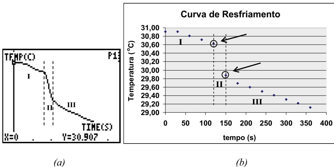
Fig. 4- Gráfico coletado, com utilização do sistema CBL, por um dos grupos de alunos durante a realização do experimento para determinação do calor específico do alumínio. Em (a) temos a representação da temperatura da água, medida em graus Celsius, versus o tempo, medido em segundos, apresentado no visor da calculadora. Em (b) os mesmos dados são ilustrados, com auxílio de uma planilha eletrônica, de forma mais detalhada. Em ambos a separação em regiões foi feita posteriormente como recurso ilustrativo.
