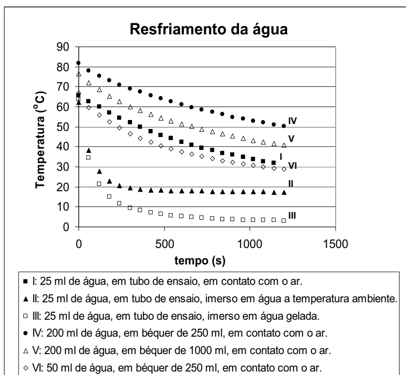
Fig. 2- Curvas de resfriamento da água coletadas pelos alunos em diferentes situações.
