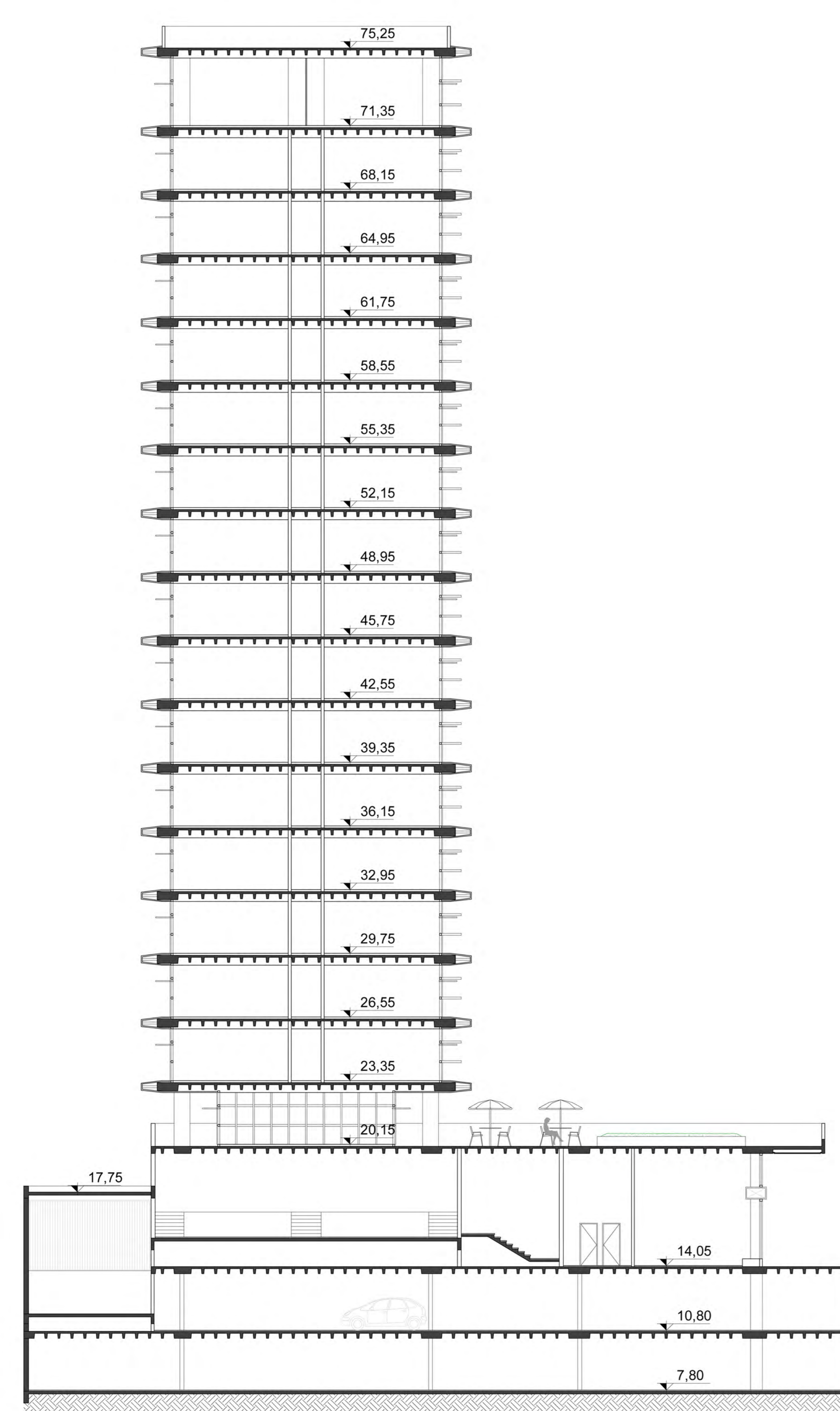
CORTE DD 1/150
