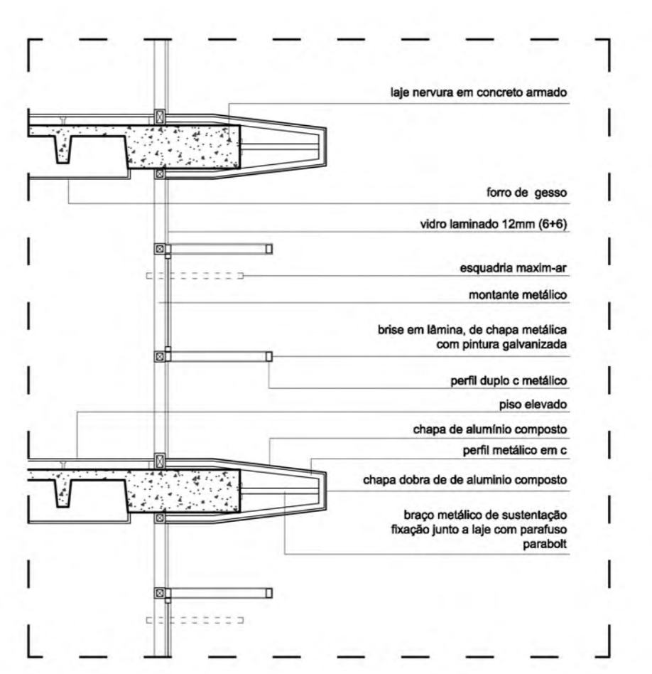
CORTE DE PELE - EDIFICIO ESCRITÓRIOS 1/50
