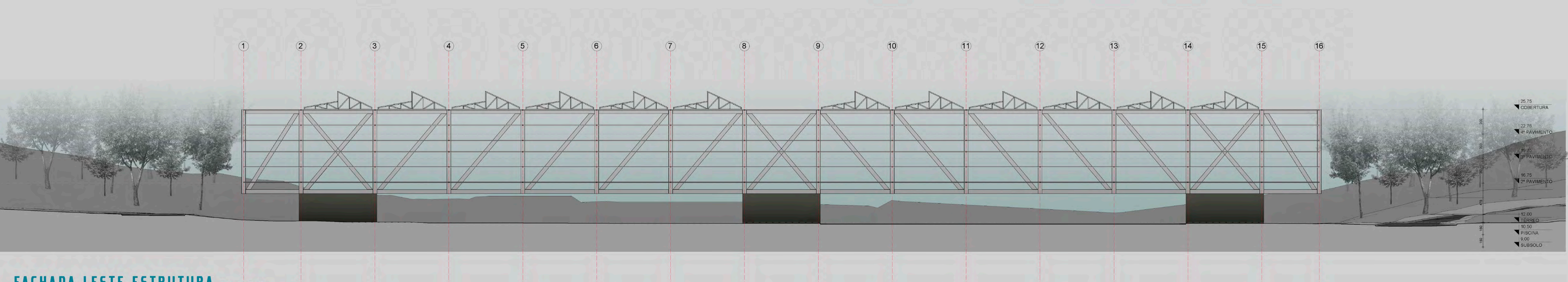
FACHADA LESTE ESTRUTURA 1/200
