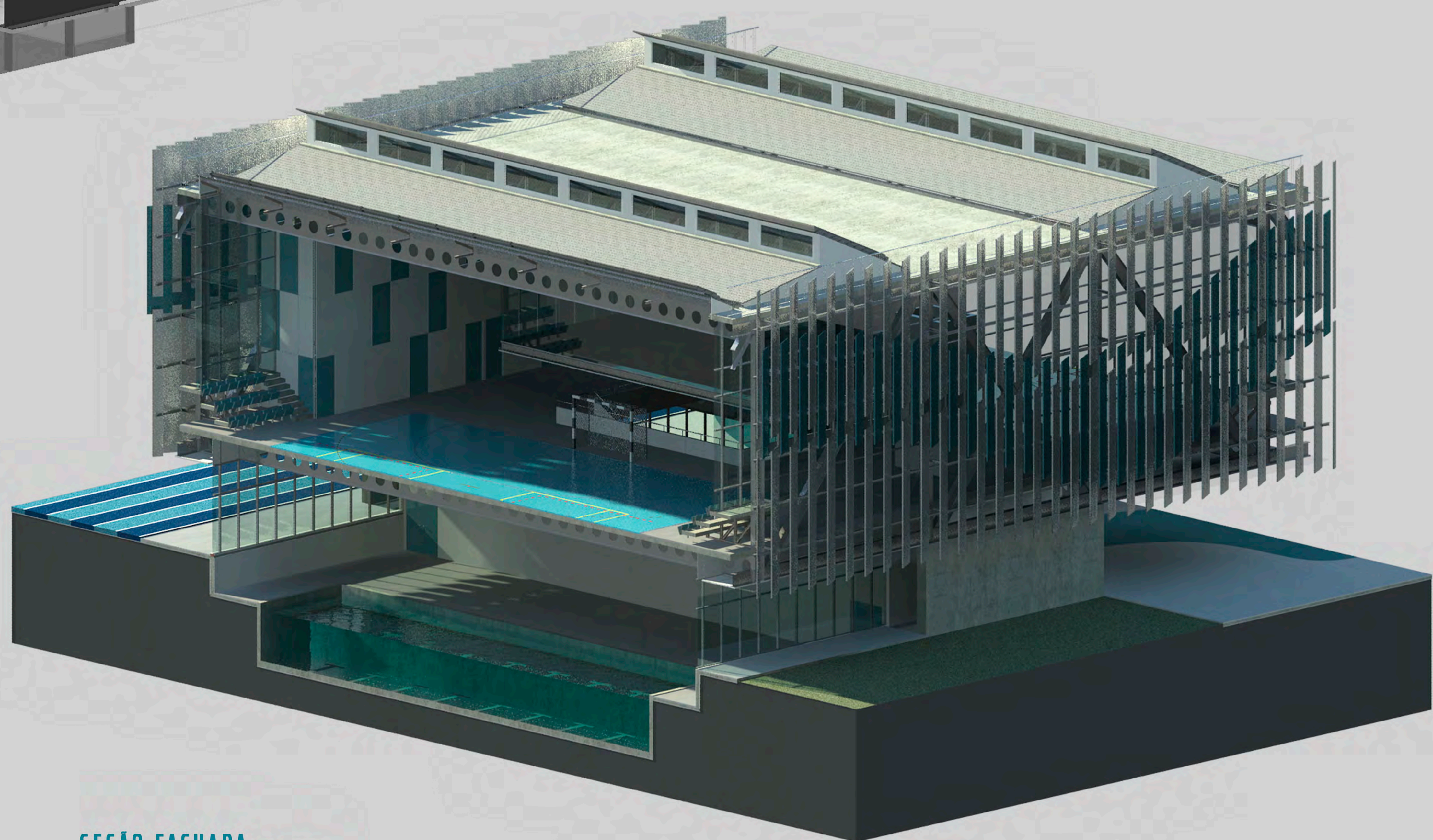
SEÇÃO FACHADA
