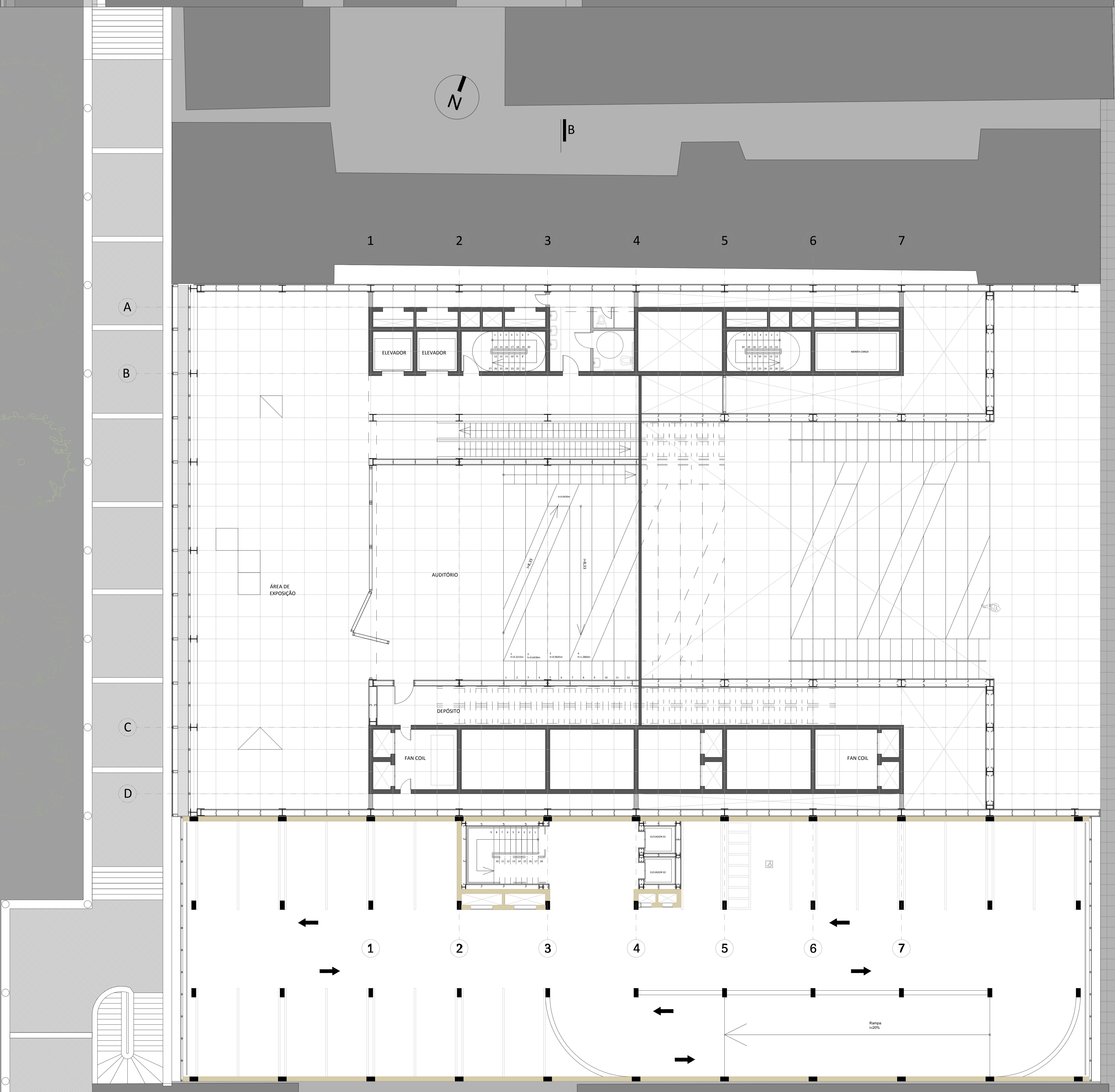
AUDITÓRIO ESCALA 1:100
