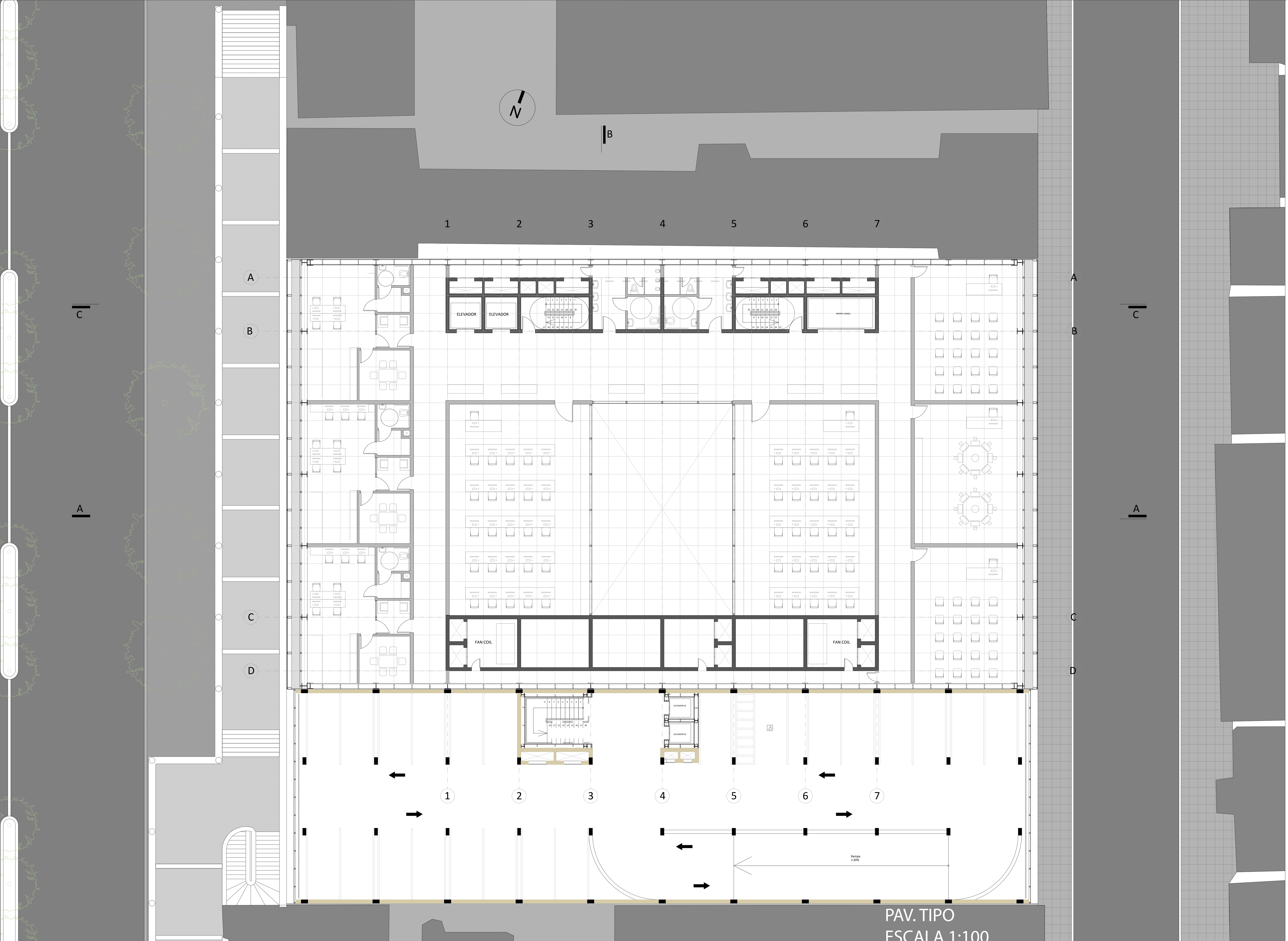
MEDIATECA ESCALA 1:100
